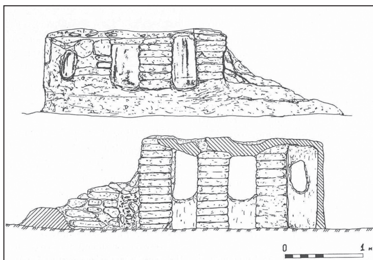
Fig. 2. Coupe du four K3 (d'après MOSCHAKIS 2000a, p. 196).
