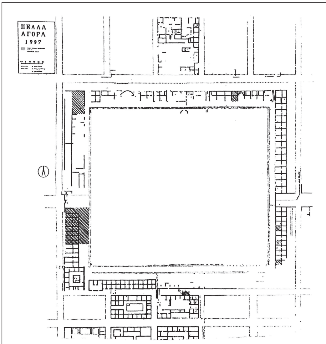
Fig. 2. Plan de l'agora (d'après AKAMATIS 1999b).
