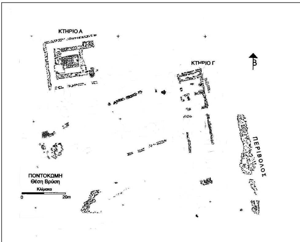
Fig. 2. Plan des bâtiments A et Γ (d'après KARAMITROU-MENTESIDI 2002, p. 617).
