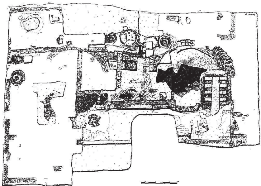
Fig. 3. Plan de l'atelier céramique et coroplastique de la partie nord de la ville (d'après LILIMPAKI-AKAMATI 1997b, p. 175).
