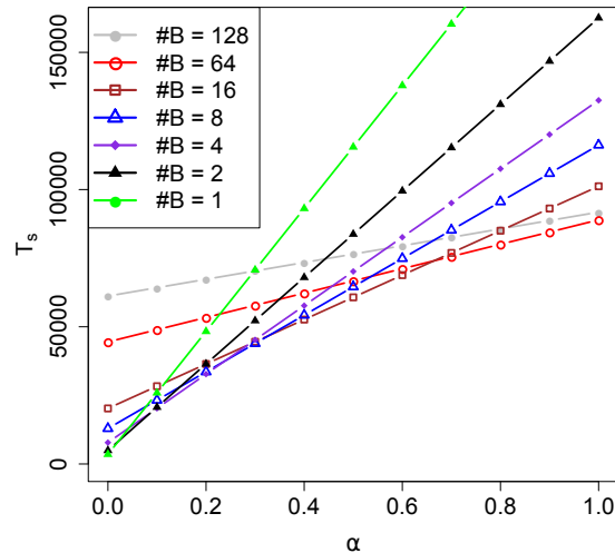
FIGURE 43 – Temps pour atteindre l’optimum global pour la stratégie adaptative poursuit (AP), en unité de fitness T_F = 1 , en fonction du paramètre \alpha pour la taille de lot différé \#B et pour n = 128 nœuds esclaves.
