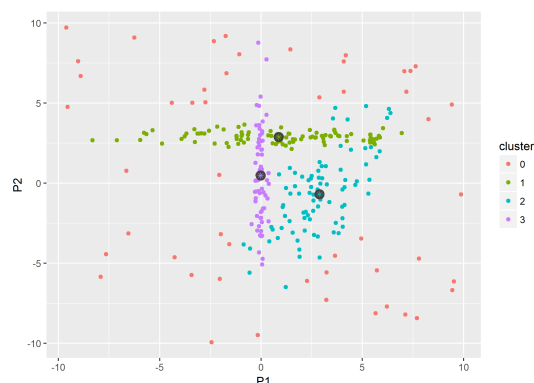
FIGURE 1.15 : Notre algorithme
