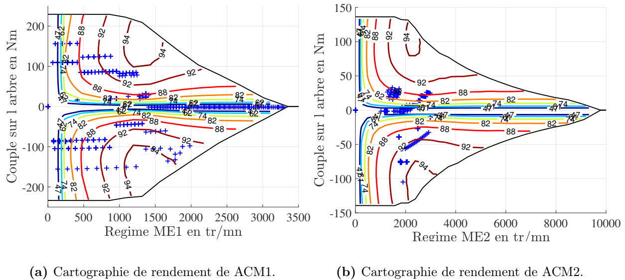
FIGURE 5.7. Cartographie de rendement des ACM dans des véhicules SPHEV1 optimaux à 25 modules de batteries (cas 2).
