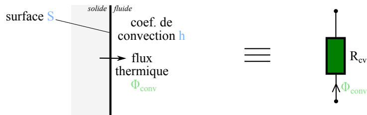
FIGURE 4.12. Représentation de la convection sur une surface par une résistance thermique équivalente. Les variables sont liées par l'équation 4.6.
