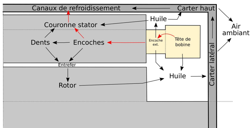
FIGURE 4.13. Zones et flux thermiques dans la machine (plan axial). Le schéma représente 1/4 de la machine (dont la moitié de sa profondeur) et n'est pas à l'échelle. Le flux principal est dessiné en rouge.
