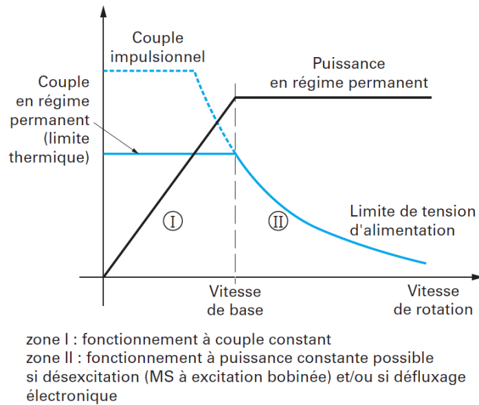
FIGURE 3.3. Caractéristique couple-vitesse type d'une machine synchrone autopilotée [72].
