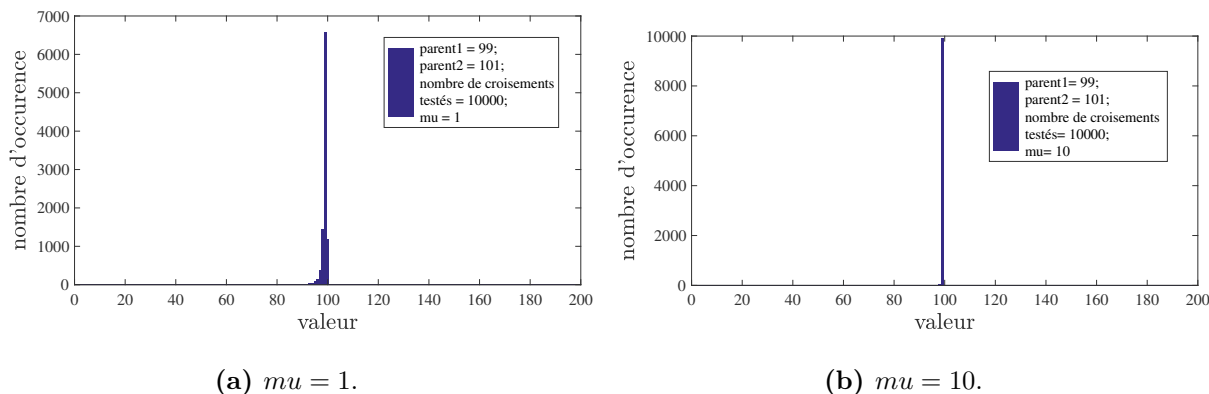
FIGURE A.3. Répartition de l'un des deux enfants obtenus lorsque l'on répète 10 000 fois le processus de croisement entre des parents rapprochés ( parent1 = 99 et parent2 = 101 ) et influence du paramètre \mu .
