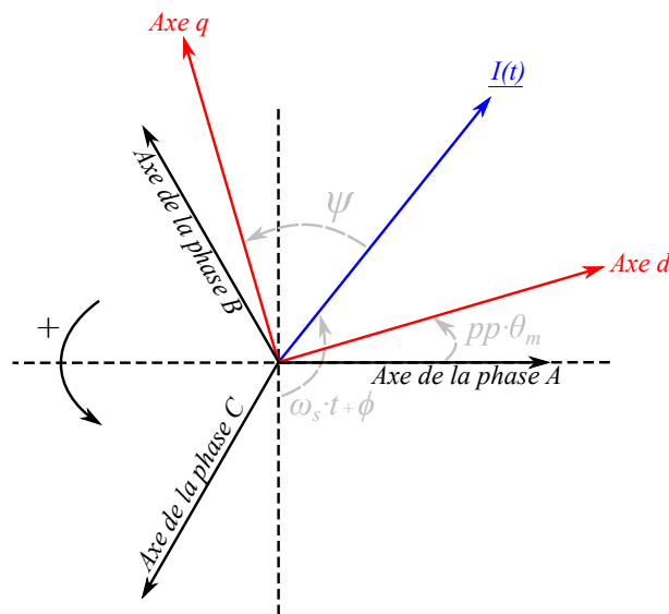
FIGURE 3.2. Notations et repères pour le fonctionnement de la machine. L'angle mécanique est noté \theta_m , le nombre de paires de pôles pp , la pulsation électrique \omega_s , le temps t . \phi est la phase du courant de la phase A pour t=0 . L'angle de commande \psi permet le contrôle entre le stator et le rotor. Dans ce cas précis, le champ magnétique \underline{I}(t) est en avance sur l'axe d ( \psi \in [-\pi/2, \pi/2] ) si l'on considère une rotation dans le sens positif. C'est donc un fonctionnement moteur. Les notations sont celles utilisées dans [1].
