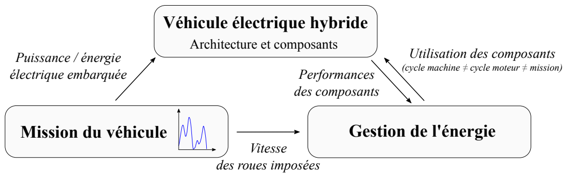
FIGURE 2.5. Le VEH dans son environnement. Nécessité d'une approche système.
