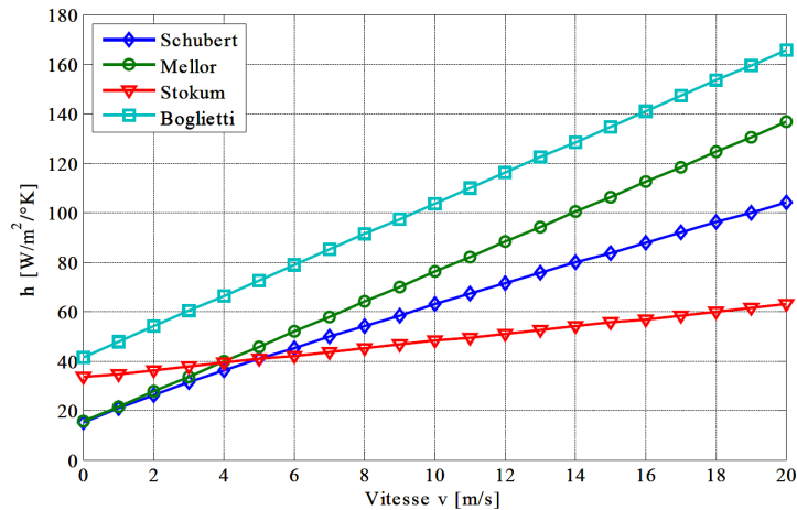
FIGURE 4.4. Évolution du coefficient de convection h autour des têtes de bobine en fonction de la vitesse périphérique du rotor [92]. Ce graphique a été construit à partir des données de [95, 107 – 109], où le fluide entourant les têtes est simplement de l'air dans la plupart des cas.
