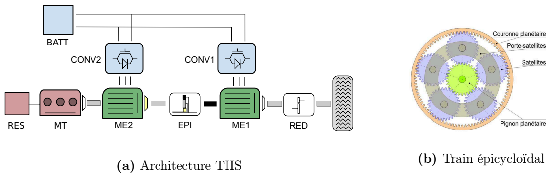
FIGURE 2.4. Exemple d'architecture à dérivation de puissance : le THS ( Toyota Hybrid System ). EPI représente un train épicycloïdal : le moteur est relié au porte satellites, la machine ME2 au pignon planétaire dit “soleil” et la machine ME1 à la couronne planétaire.
