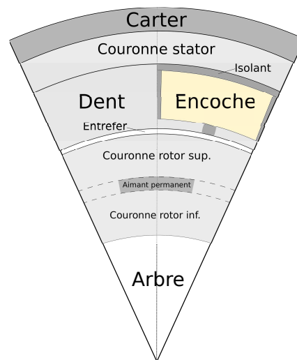
FIGURE 4.14. Simplification en cellules cylindriques de la machine (coupe axiale). Le schéma représente 1/16^{\text{ème}} de la machine ( 1/2 pôle) et n'est pas à l'échelle. Notons que les 3 dents et les 3 encoches sont regroupées en 2 zones distinctes mais que les surfaces réelles d'échanges seront considérées lors du calcul des résistances thermiques.
