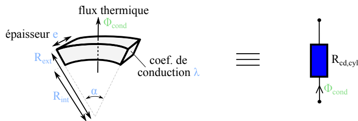
FIGURE 4.11. Représentation de la conduction à travers une portion de cylindre par une résistance thermique équivalente. Les variables sont liées par l'équation 4.5.
