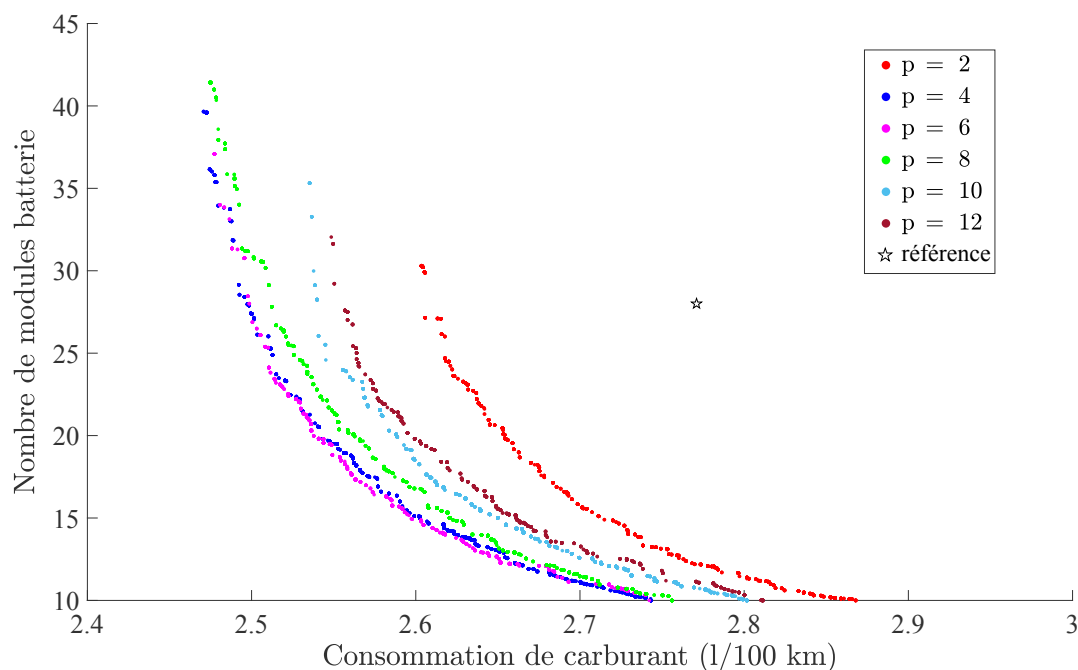
FIGURE 3.13. Comparaison des fronts de pareto obtenus pour les différentes valeurs de p .
