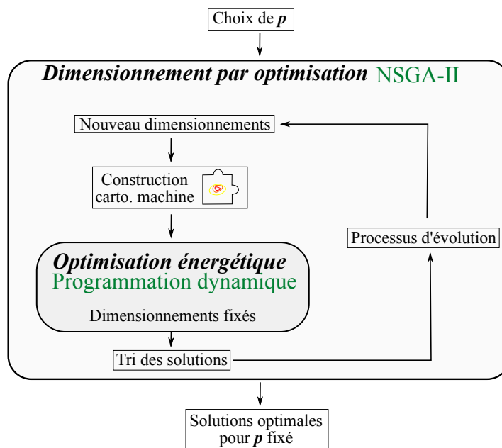
FIGURE 3.12. Processus d'optimisation lancé pour chacune des valeurs possibles pour p .
