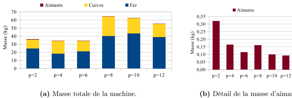
FIGURE 4.25. Comparaison de la masse des machines électriques dans des véhicules du front de pareto et embarquant 28 modules de batterie, selon la valeur de p . La contrainte thermique est prise en compte.
