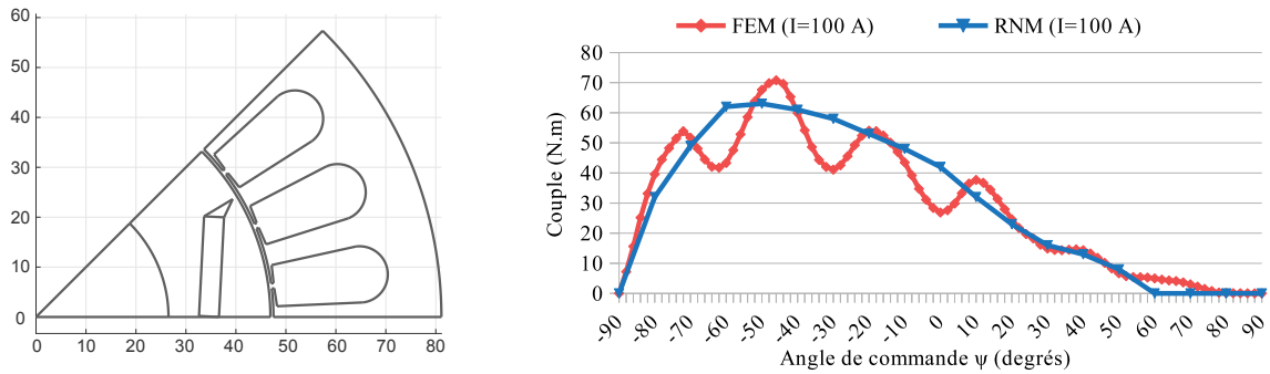
(a) Dessin de la machine (1/2 pôle) en millimètre. Sa profondeur est de 127,45 mm. (b) Validation du couple pour une machine à 4 pôles : comparaison des modèles FEM et RNM. Le courant est fixé à 100 A
