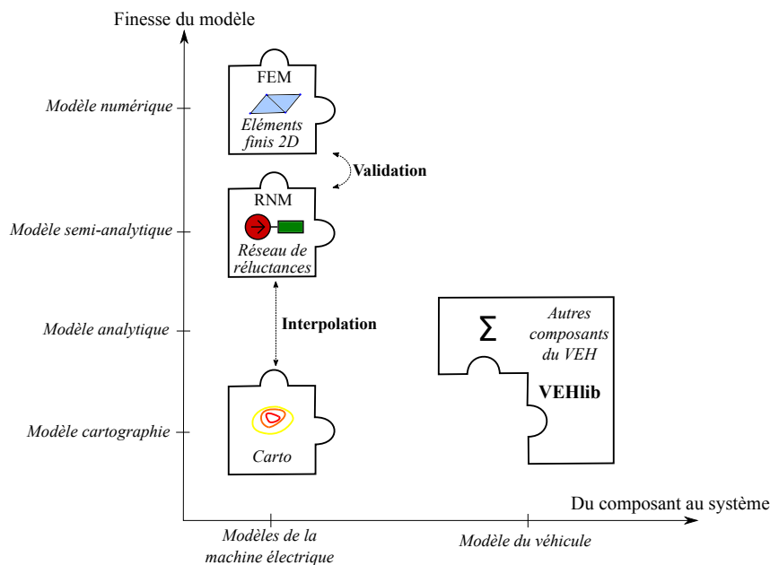
FIGURE 2.11. Classification des modèles utilisés par Vincent Reinbold.
