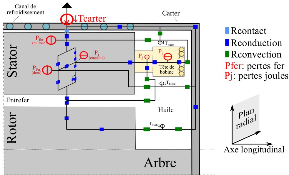
FIGURE 4.17. Réseau de résistances thermiques complet de la machine.
