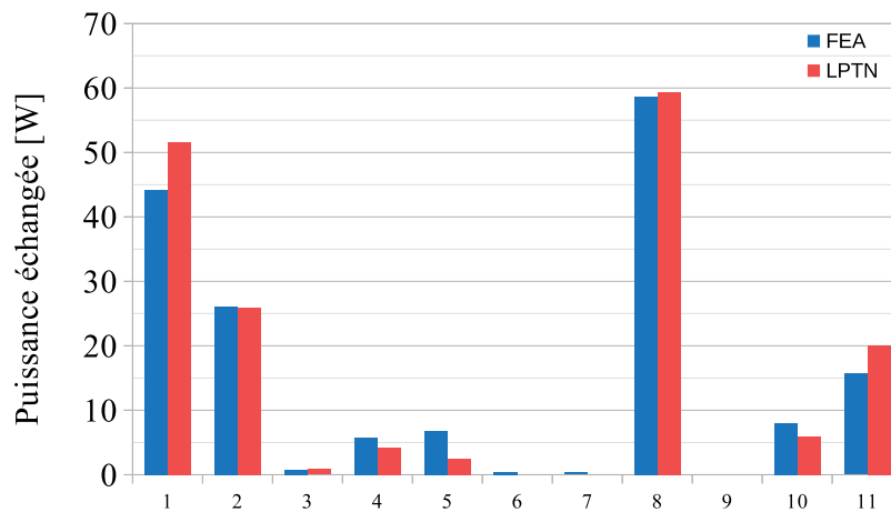
FIGURE 4.19. Flux de chaleur dans la machine. Comparaison des modèles par éléments finis (FEA, en bleu) et par réseau de résistances (LPTN, en rouge). Voici la correspondance entre les nombres en abscisse et les échanges mesurés :
