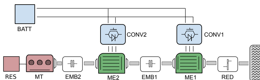
FIGURE 2.3. Architecture série/parallèle à deux embrayages.
