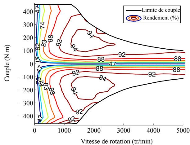
FIGURE 2.13. Exemple de cartographie de rendement de la machine électrique.
