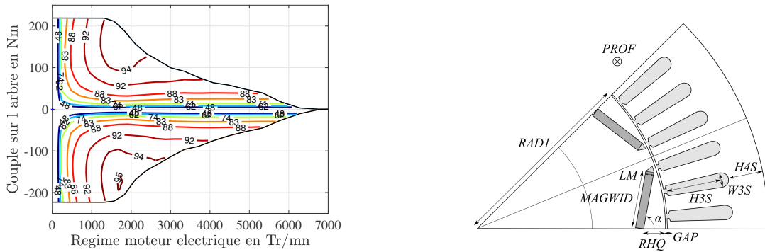
(a) Modèle simple : cartographie de rendement issue du modèle de l'association convertisseur/machine (ACM1) de la Toyota Prius 2004 ( cf. figure 5.3). Notons que le modèle thermique est considéré. (b) Modèle fin : description des variables géométriques associées à la machine électrique ( \mathbb{X}_{me} ).
