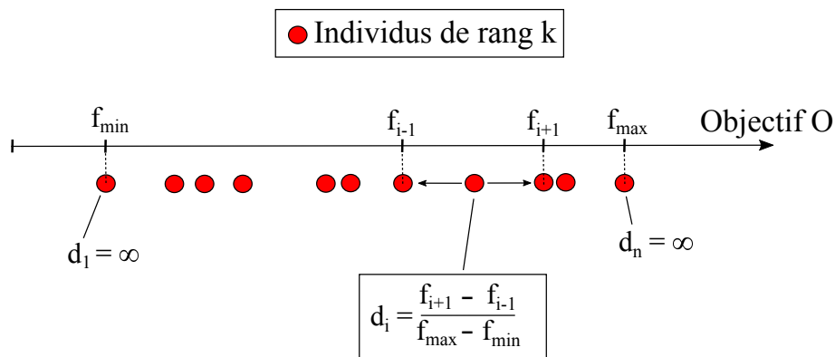
FIGURE A.2. Calcul de la crowding distance pour un individu i de rang k selon l'objectif O .
