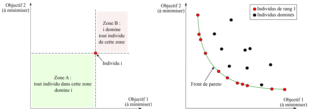
(a) Définition du concept dominé/non-dominé pour l'optimisation multi-objectifs, où les objectifs 1 et 2 sont à minimiser. (b) Définition du concept de front de pareto.
