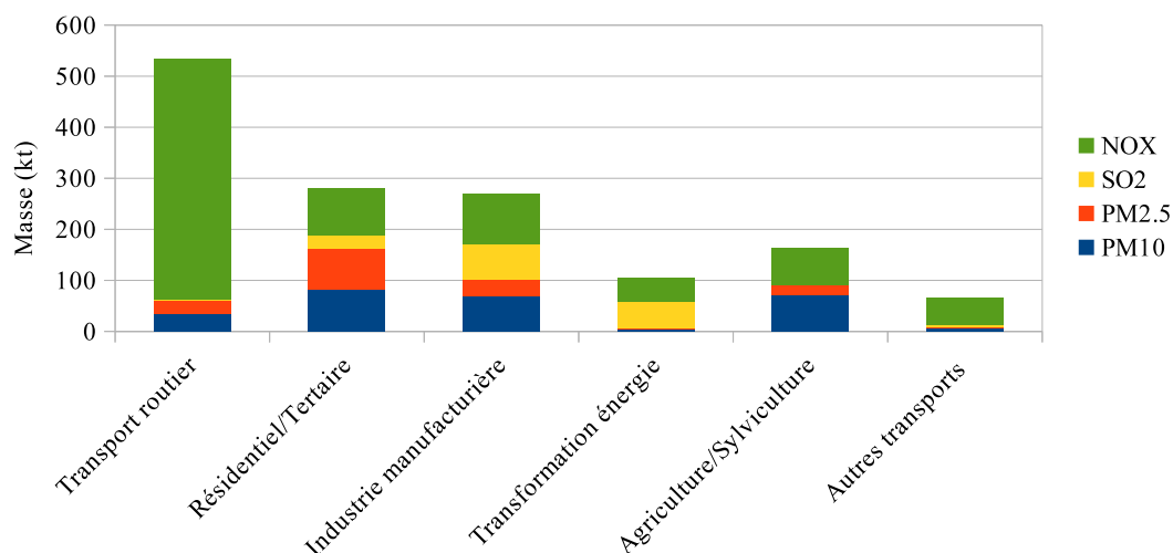
FIGURE 1.3. Émissions des principaux polluants atmosphériques par secteur, en kt, en France (2015). Les oxydes d’azote ( NO_x , dont NO_2 ) sont très toxiques et à l’origine de l’ozone troposphérique, qui cause le “smog”. Le dioxyde de soufre ( SO_2 ) et les particules fines ( PM ) sont les autres polluants considérés.
