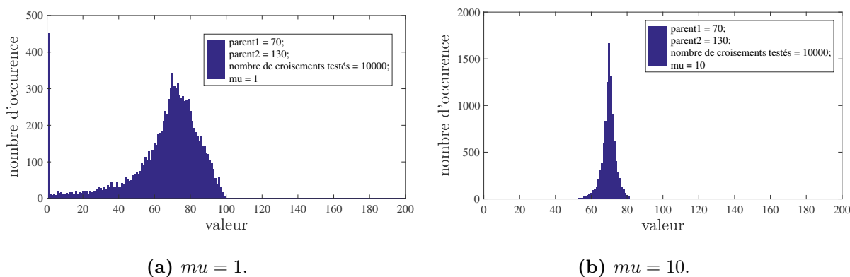
FIGURE A.4. Répartition de l'un des deux enfants obtenus lorsque l'on répète 10 000 fois le processus de croisement entre des parents éloignés ( parent1 = 70 et parent2 = 130 ) et influence du paramètre \mu . Notons que l'enfant ne peut pas sortir de l'intervalle [1; 200] .
