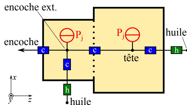
FIGURE 4.16. Modèle de la tête de bobine dans le plan axial. En plus des échanges par conduction, des échanges convectifs (en vert) ont lieu avec l'huile sur toutes les surfaces externes de la tête et de l'encoche ( h_{oil} = 25 \text{ W} \cdot \text{m}^{-2} \cdot \text{°C}^{-1} ).
