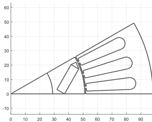
(a) Dessin en millimètre (1/2 pôle) de la machine à 6 pôles obtenue pour un système optimal. Sa profondeur active (hors têtes de bobine) est de 111,6 mm.
