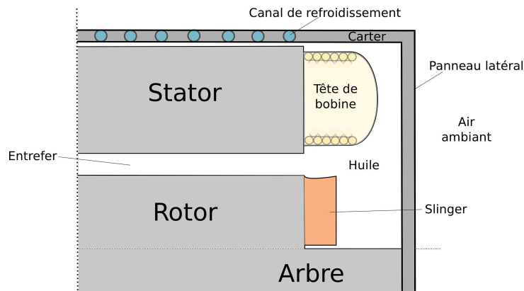
FIGURE 4.6. Description de la machine d'un point de vue thermique (plan axial). Le schéma représente 1/4 de la machine (dont la moitié de sa profondeur) et n'est pas à l'échelle.
