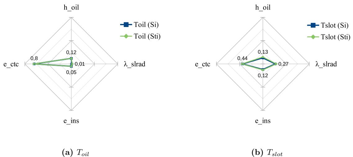
FIGURE 4.22. T_{oil} et T_{slot} : indices de Sobol de 1 er ordre ( S_i ) et indice total ( S_{Ti} ) obtenus pour les paramètres thermiques h_{oil} , e_{ctc} , e_{slins} et \lambda_{slrad} .
