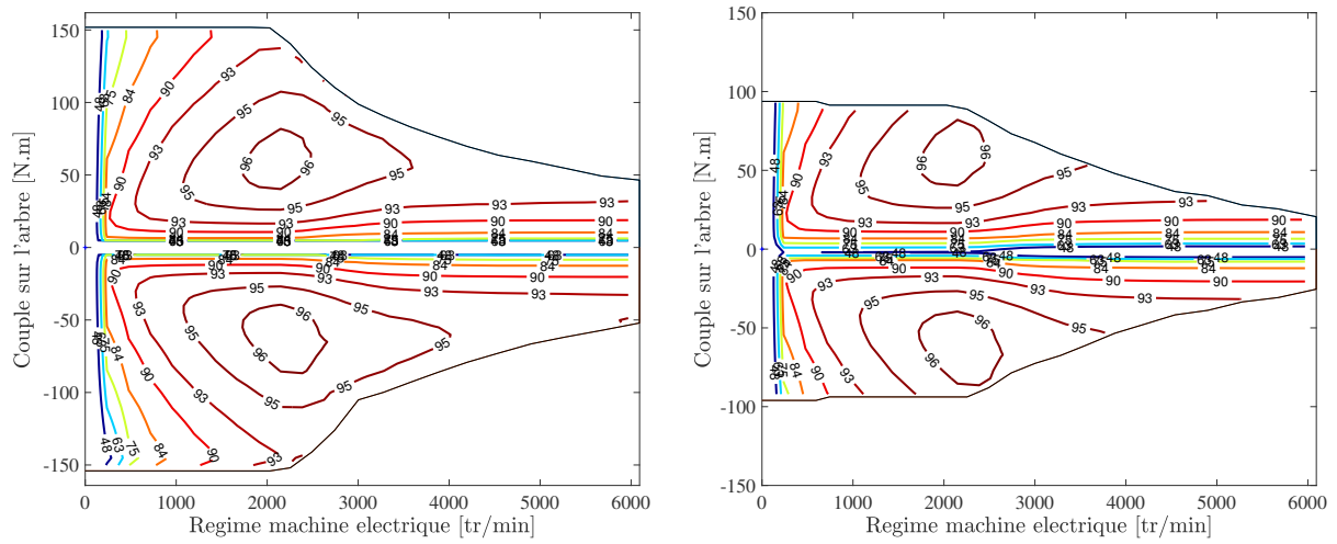
(a) Cartographie d'une machine à 4 pôles sans contrainte thermique. (b) Cartographie de la même machine avec la contrainte thermique.
