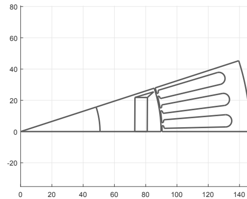
(b) Dessin en millimètre (1/2 pôle) de la machine à 10 pôles obtenue pour un système optimal. Sa profondeur (hors têtes de bobine) est de 77,1 mm.
