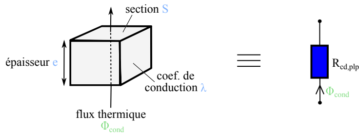
FIGURE 4.10. Représentation de la conduction à travers un parallélépipède par une résistance thermique équivalente. Les variables sont liées par l'équation 4.4.
