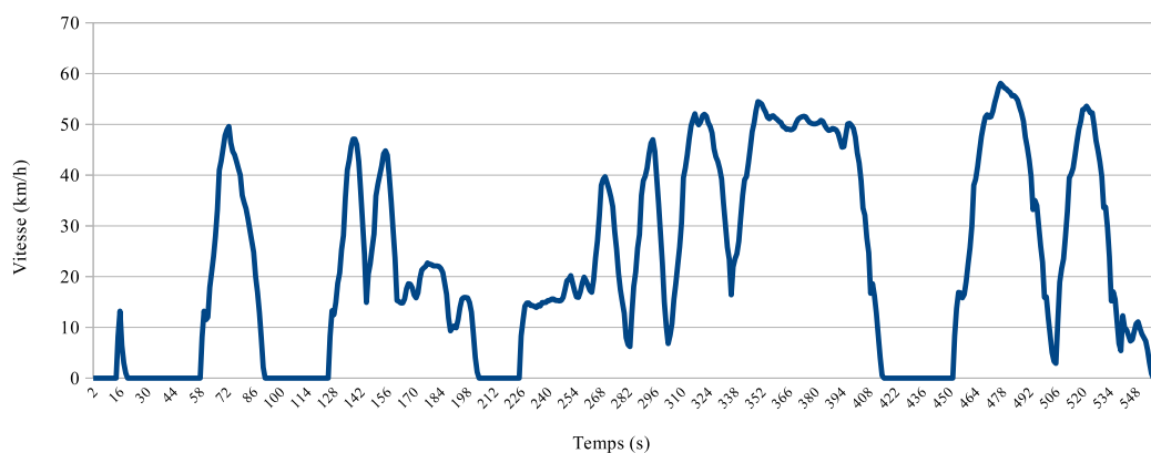
FIGURE 2.6. Cycle de conduite Hyzem urbain.
