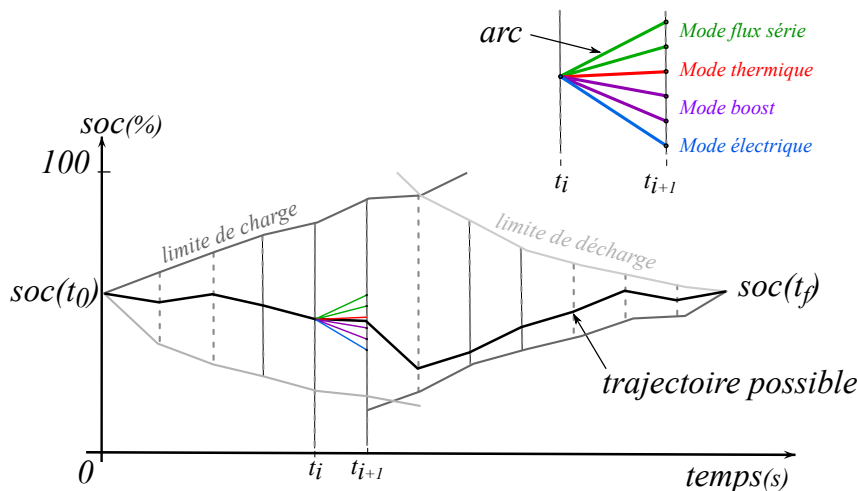
FIGURE 2.10. Représentation du problème de gestion de l'énergie, tel qu'il est abordé via un algorithme de programmation dynamique. Notons l'égalité entre l'état de charge initial ( \text{soc}(t_o) ) et final ( \text{soc}(t_f) ).
