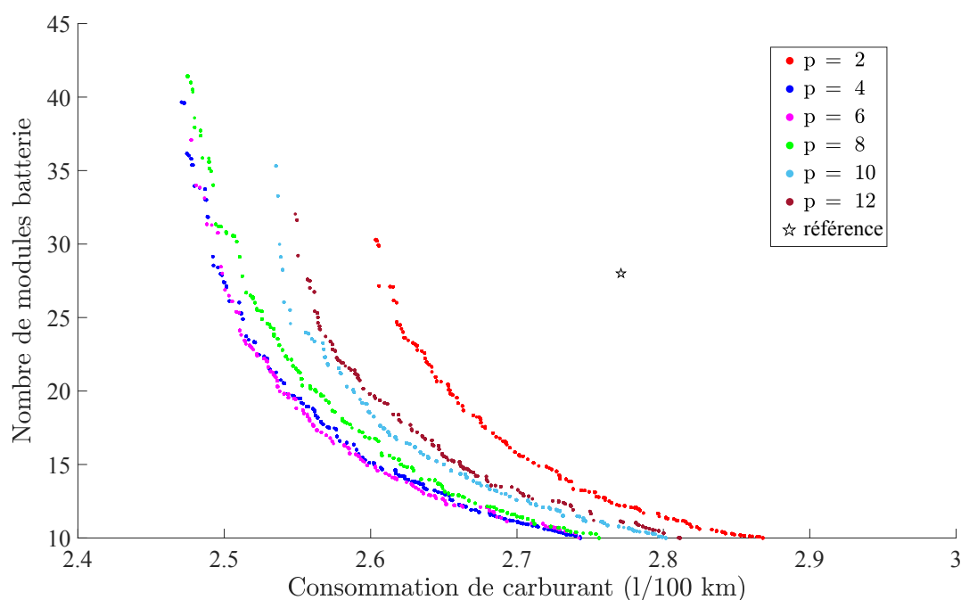
FIGURE 3.13. Comparaison des fronts de pareto obtenus pour les différentes valeurs de p .
