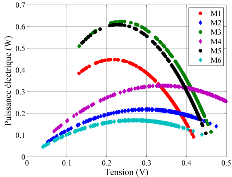
Figure III.12 Puissance électrique générée par les six modules Bi 2 Te 3 de ThermoGen pour une température d'entrée de 300 °C et un débit d'air de 117 kg.h -1
