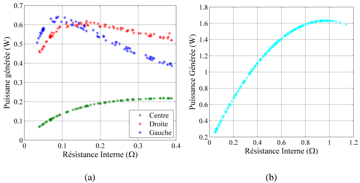
Figure IV.14 Puissance expérimentale mesurée pour T_{entrée} = 300\text{ °C} et débit = 47\text{ kg.h}^{-1} pour : (a) les branches gauche, droite et centrale (b) tous les modules en série
