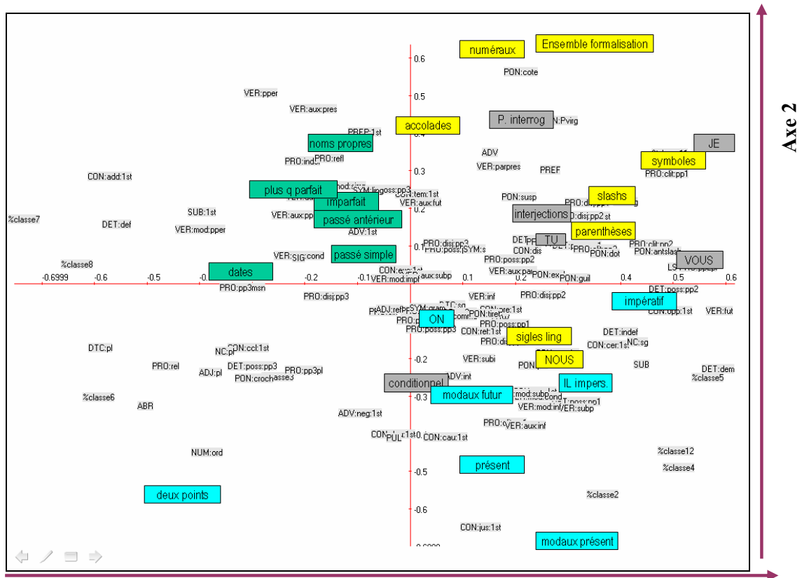
Figure 6.10. Positionnement des variables sur les deux premiers axes factoriels – corpus « auteurs ».
