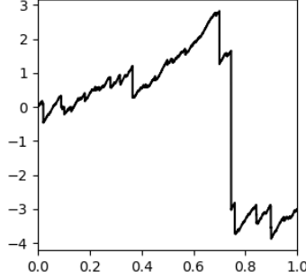
(b) Processus (6/5) -stable, à saut négatif, avec compensation des sauts par dérive "infinie", avec taux de sauts x^{-11/5} \mathbf{1}_{x<0} dx .
