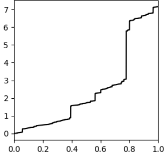
(a) Processus (4/5) -stable, à saut positif, sans compensation des sauts par dérive, avec taux de sauts x^{-9/5} \mathbf{1}_{x>0} dx .
