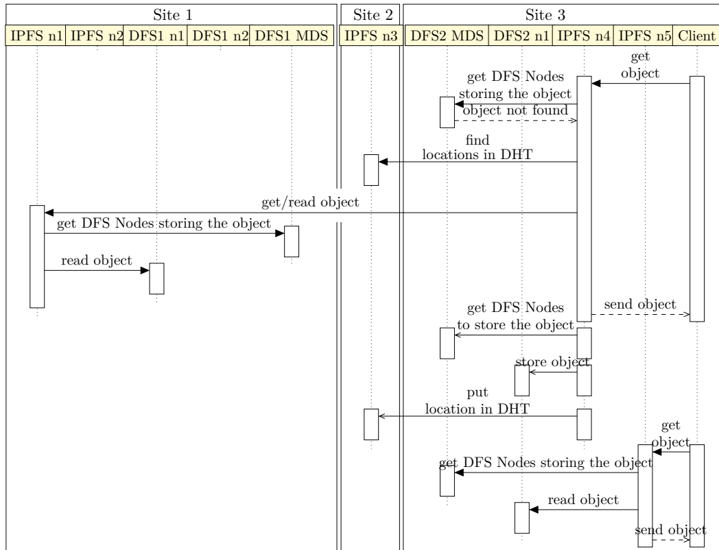
(c) – Lecture d'un objet stocké sur un site distant.
