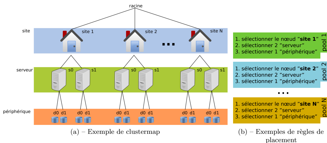
FIGURE 4.4 – Exemples de clustermap (a) ainsi que les règles de placement associées aux pools dans un contexte de Fog (b). Le site stockant les réplicas est précisé dans chaque règle. Par exemple, tous les objets appartenant au « pool N » sont stockés sur le site N.
