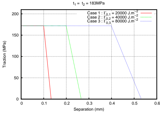
FIG. L.1: Loïs de traction séparation à T_0 fixé
