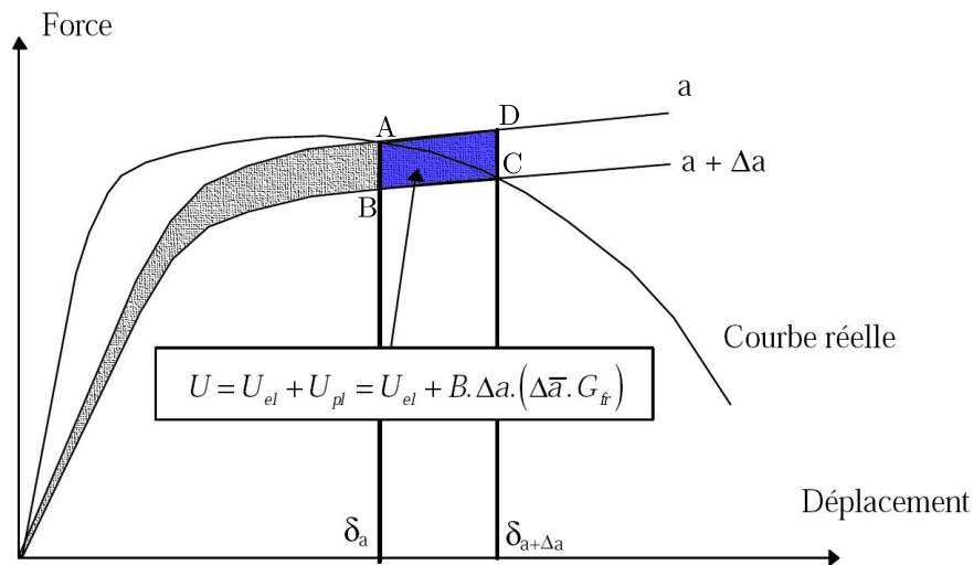
FIG. 3.12: Interprétation géométrique de G_{fr} [MAR 99]
