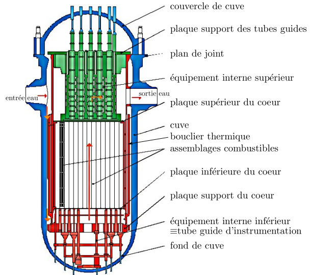
FIG. 1.2: Assemblage d'une cuve [VER 04] FIG. 1.3: Schéma de la cuve d'un réacteur 900MW
