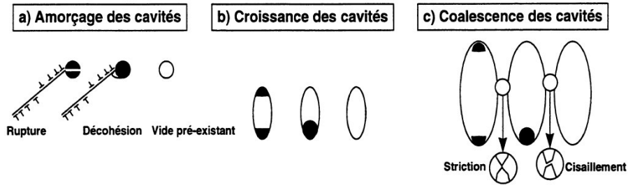
FIG. 3.1: Endommagement ductile [MIA 95]
