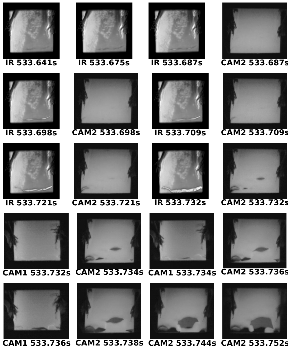
FIG. I.15: Images de la propagation de fissure
