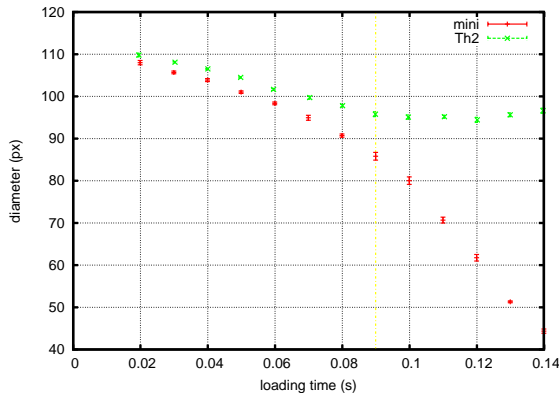
FIG. M.24: EP18-diamètre
