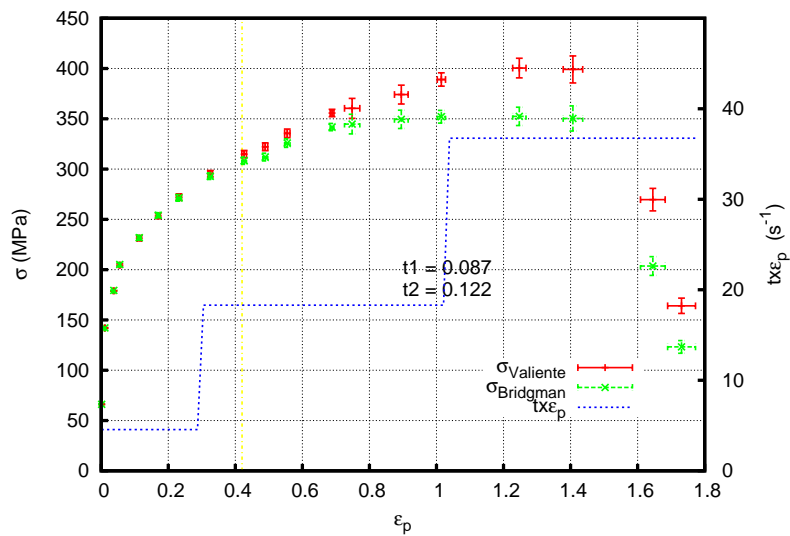
FIG. M.20: EP22-Déformation plastique équivalente
