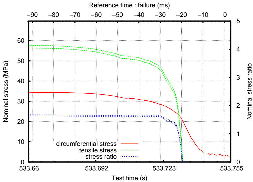
FIG. I.14: Contraintes nominales pendant la propagation instable de la fissure
