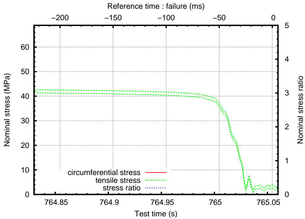
FIG. G.16: Contraintes nominales pendant la propagation instable de la fissure
