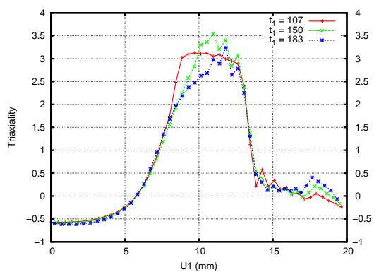
FIG. 4.20: Répartition du taux de triaxialité (environ 4mm de propagation, \Gamma_0 = 50 \text{ kJ.m}^{-2} , t_2 = 183 \text{ MPa} )
