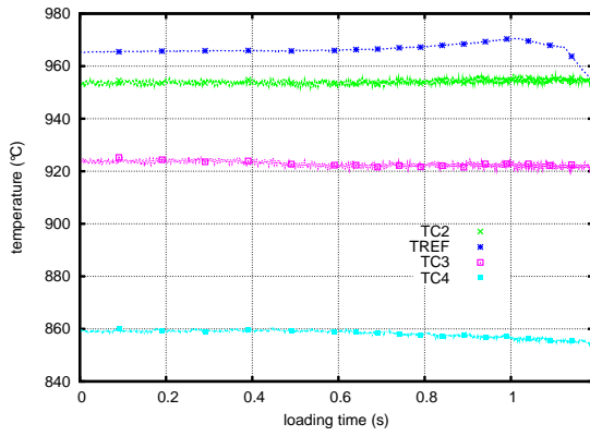
FIG. M.12: EP16-Température
