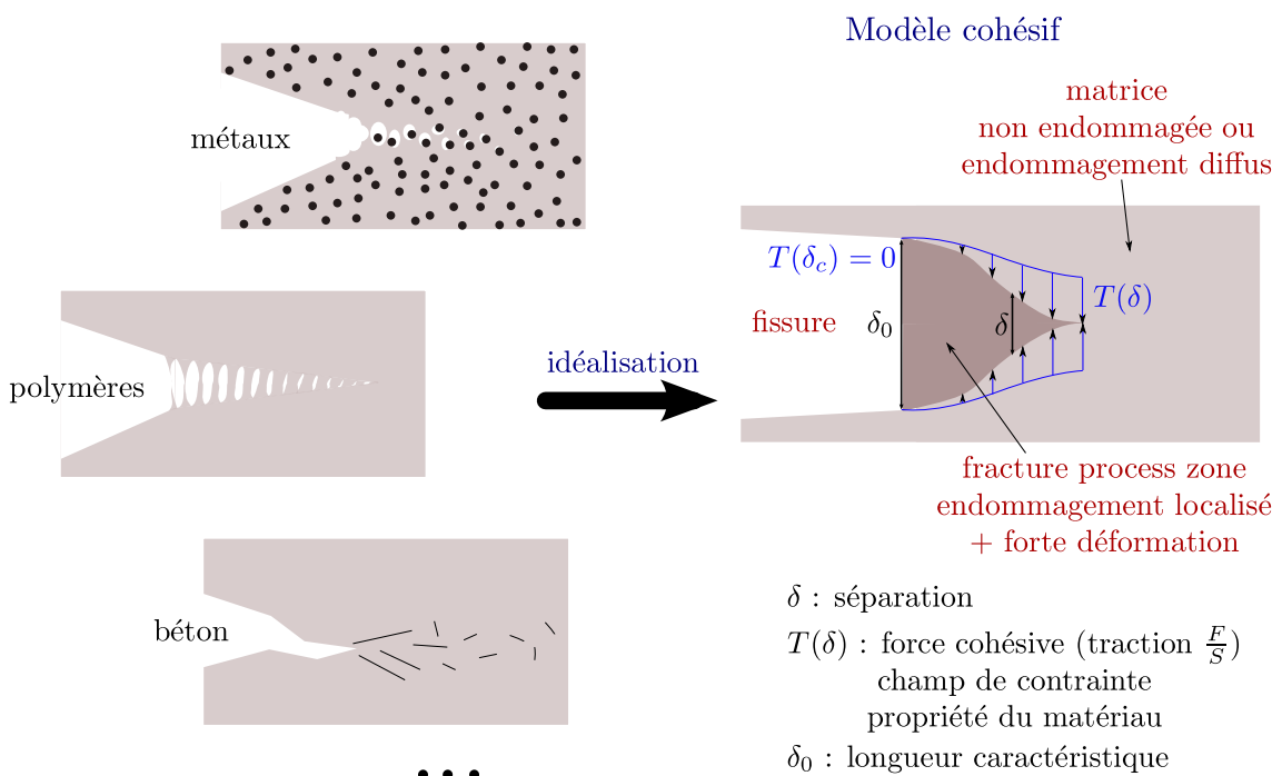
FIG. 3.4: Modèle cohésif
