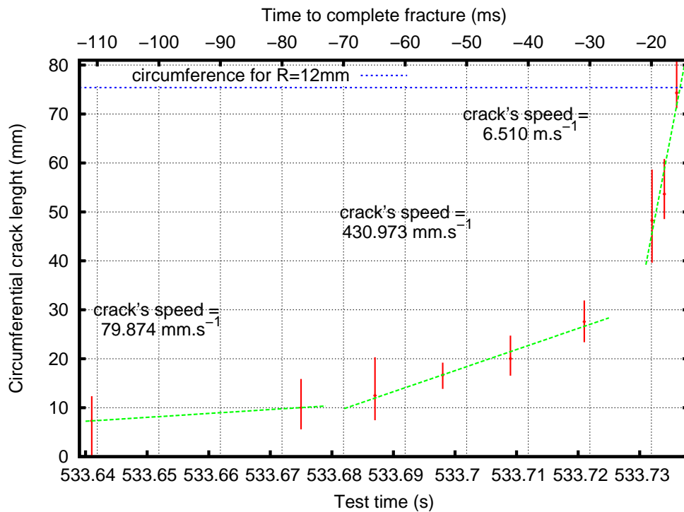
FIG. I.17: Propagation circconférentielle
