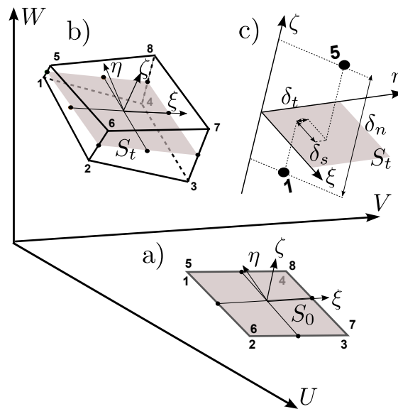
FIG. 4.5: élément d'interface dans sa configuration initiale (a), sa configuration déformée (b) et caractérisation de la séparation de deux noeuds dans la configuration déformée (c)
