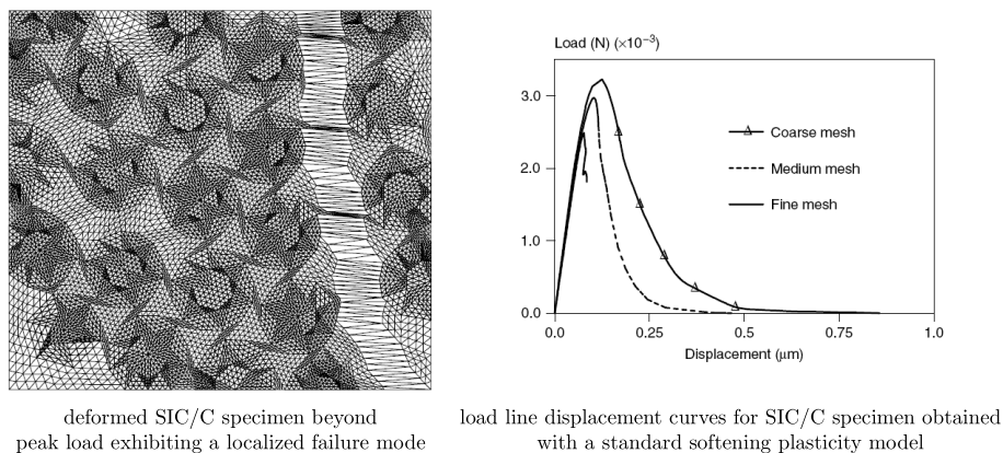
FIG. 3.3: Approche locale : dépendance au maillage [BOR 04]
