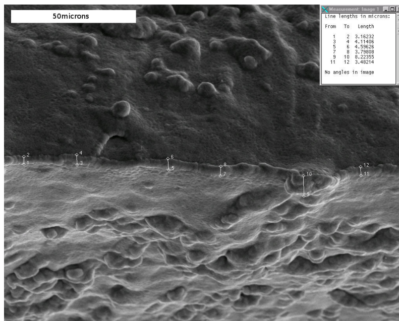
FIG. I.27: Faciès de rupture : vue de dessus
