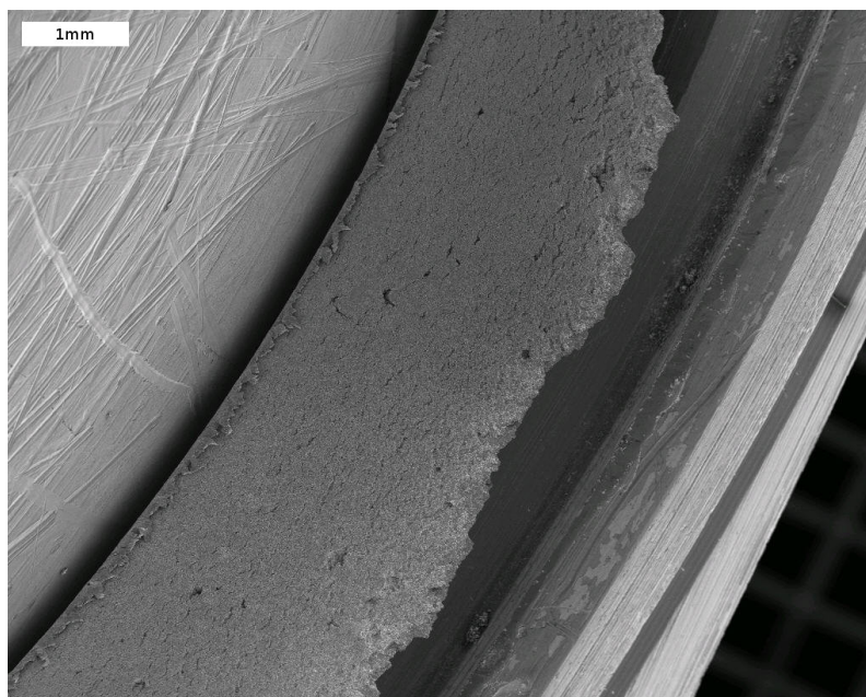
FIG. D.36: Paroi interne : vue de côté
