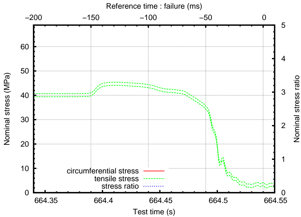
FIG. E.16: Contraintes nominales pendant la propagation instable de la fissure
