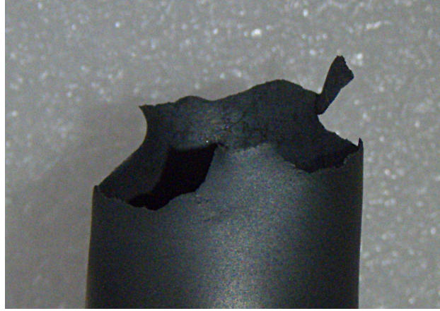
FIG. E.22: Planéité de la trajectoire de la fissure
