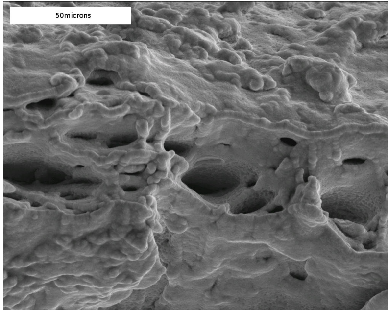
FIG. J.28: Faciès de rupture : vue de dessus
