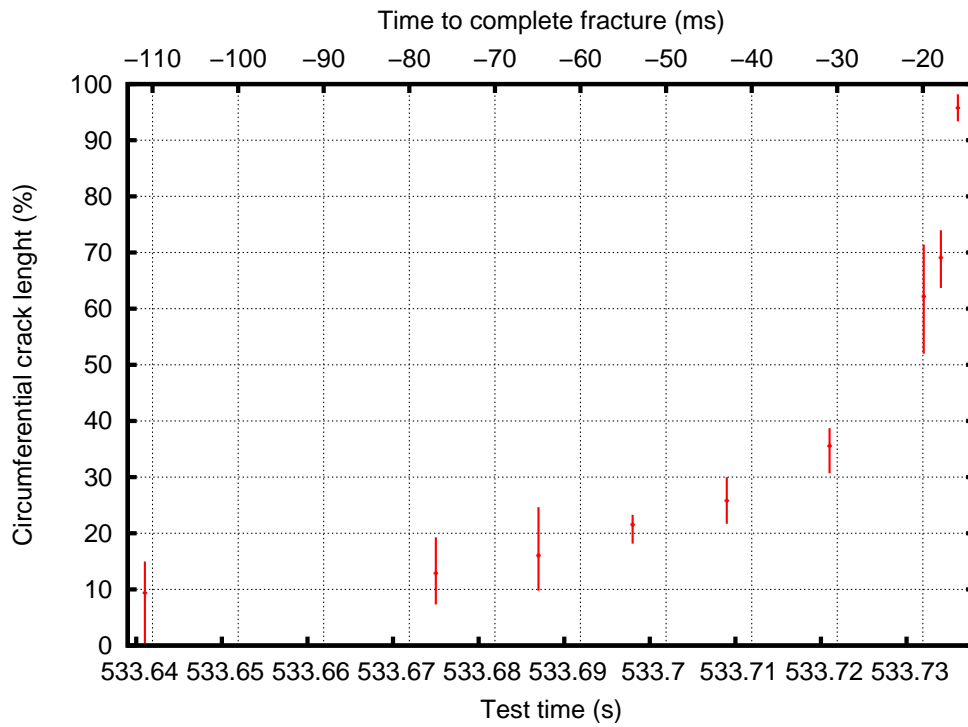
FIG. I.16: Propagation circconférentielle
