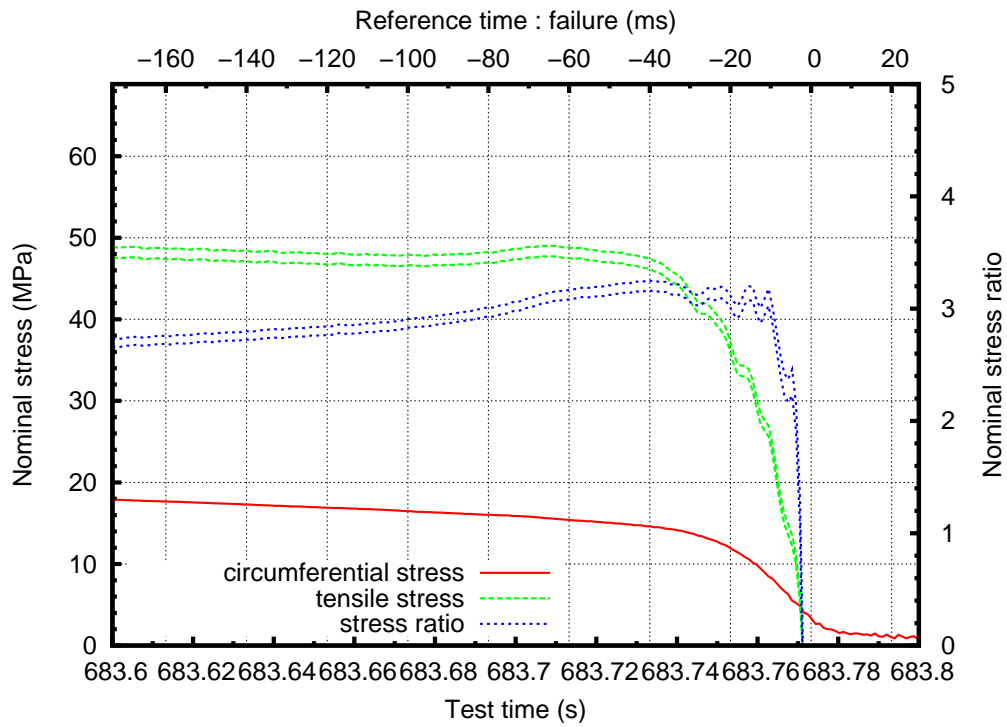
FIG. D.16: Contraintes nominales pendant la propagation instable de la fissure
