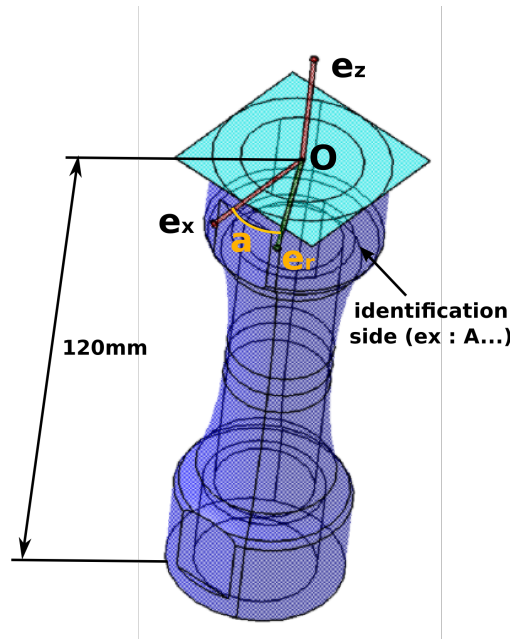
FIG. I.2: Repère de métrologie
