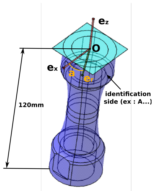
FIG. K.2: Repère de métrologie
