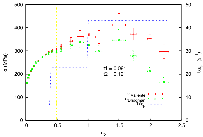
FIG. M.5: EP12-Déformation plastique équivalente
