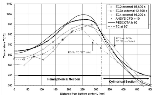
FIG. 1.14: FOREVER : distribution thermique de la maquette lors de l'essai [ALS 05]
