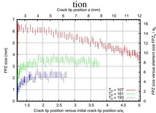
FIG. L.8: Influence de T_0 sur la taille de la fracture process zone
