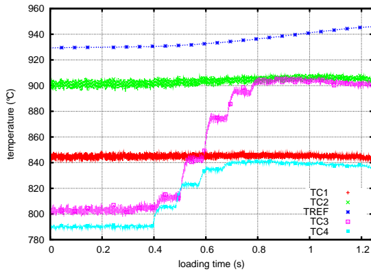
FIG. M.7: EP13-Température
