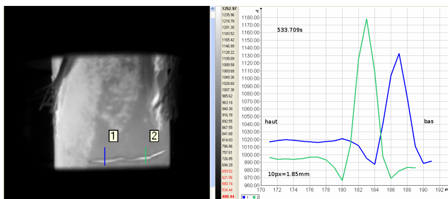
FIG. I.23: Distribution de température mesurée sur un profil coupant la fissure
