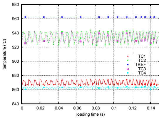
FIG. M.32: EP20-Température
