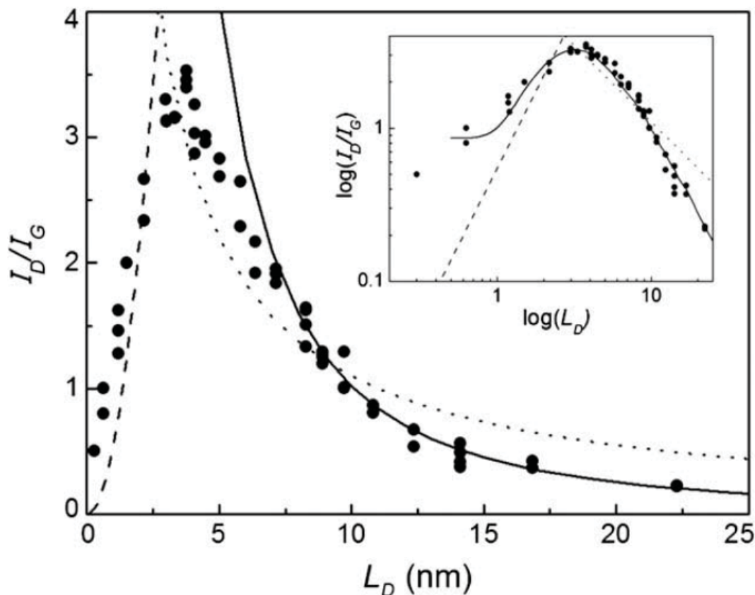
Figure 3.2.11 Figure issue de Lucchese et al. [28] . Les courbes en pointillés correspondent à 0,0055L_D^2 d'après la publication de Ferrari et Robertson , les points à 11/L_D soit 2,5 fois la loi de Tuinstra et Koenig ( 4,4/L_D ) et la ligne correspond à 102/L_D^2 , une valeur approchée de leur propre modèle. L'encart montre la même figure en représentation LogLog où la ligne représente cette fois-ci leur modèle complet.
