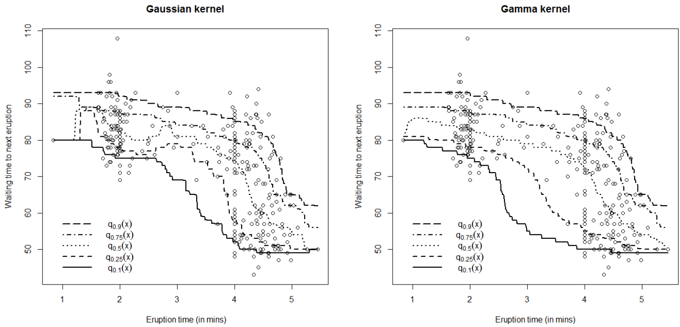
FIGURE 3.5 – Courbes de référence avec le noyau Gaussian/Gamma .
