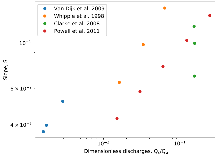
FIGURE 1.10 : Pente du cône en fonction du rapport des flux. Modifié d'après Van Dijk et al. (2009).
