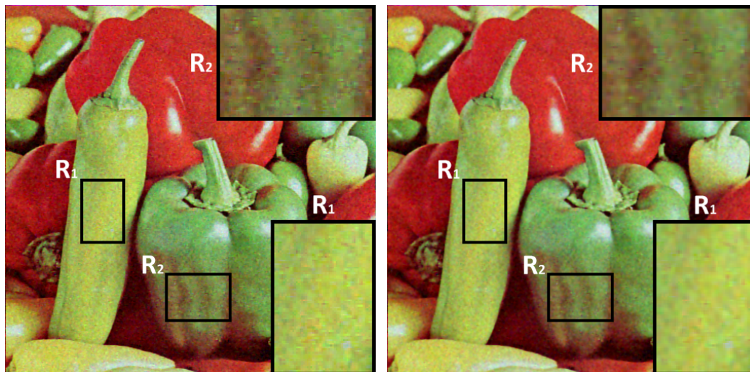
(c) OMP (26.52 - 0.552)
