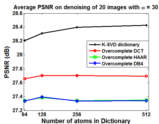
(d) \sigma = 30
