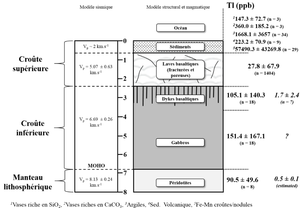
Figure 1 : Abondance relative du thallium dans les différents compartiments de la lithosphère océaniques. Les données présentées ici montrent une estimation de la composition de la lithosphère océanique au niveau des dorsales. Les phénomènes de zone de subduction n'apparaissent pas. Les données en gras proviennent de : De Albuquerque et al. (1971), Heinrichs et al. (1980), Sahl et al. (1978), Rekhämper et al. (2002), Nielsen et al. (2006a, 2014, 2016, 2017), Jenner et al. (2012) et Kelley et al. (2013). Les données en italiques sont issues de la compilation des données des articles de Nielsen et al. (2006a, 2014, 2016, 2017). Le schéma est adapté de Juteau et Maury (2008).
