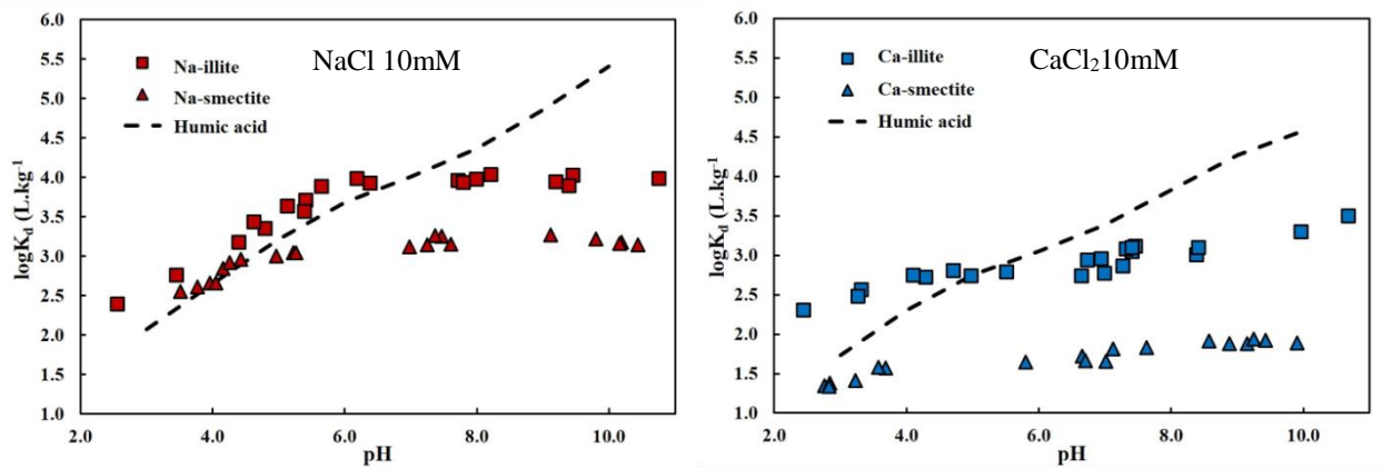
Figure 1 : Comparaison des interactions matière organique thallium et illite/smectite et thallium.
