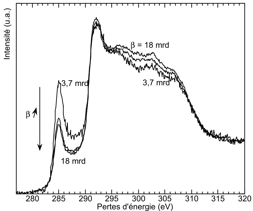
Figure 112 : spectres C-K de la fibre K-1100 pour trois angles \beta différents normalisés au maximum
