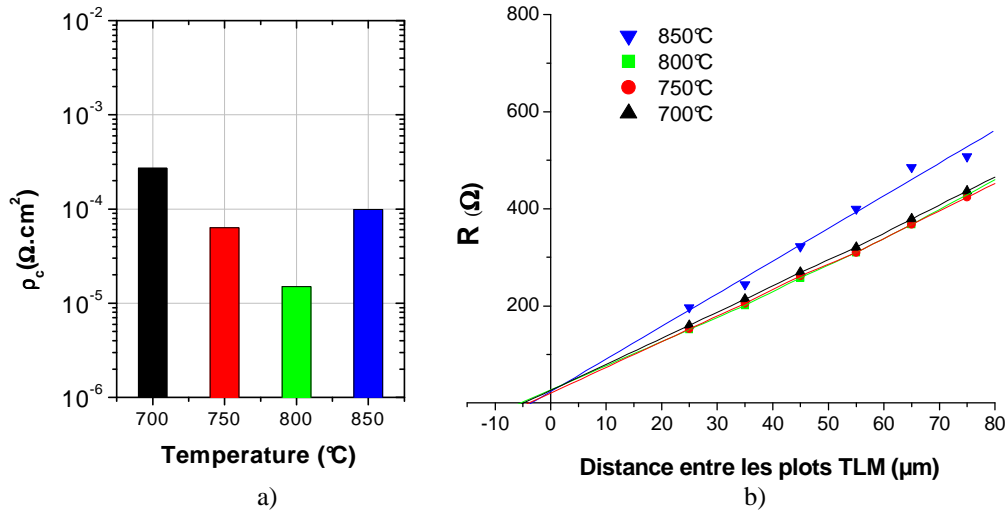
Fig.II.3.70 Dépendance de la résistance spécifique du contact Ni(10)/Ti(40)/Al(240)/Ni(10nm) vs la température de recuit utilisée pour former ces contacts (a). Résistance mesurée entre plots TLM en fonction de la distance entre les plots pour différentes températures de recuit (b).
