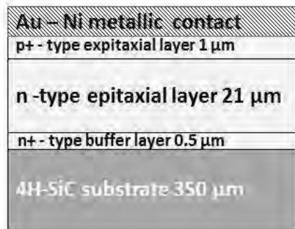
Fig.II.5.10 Structure du détecteur de neutrons rapides réalisé en SiC
