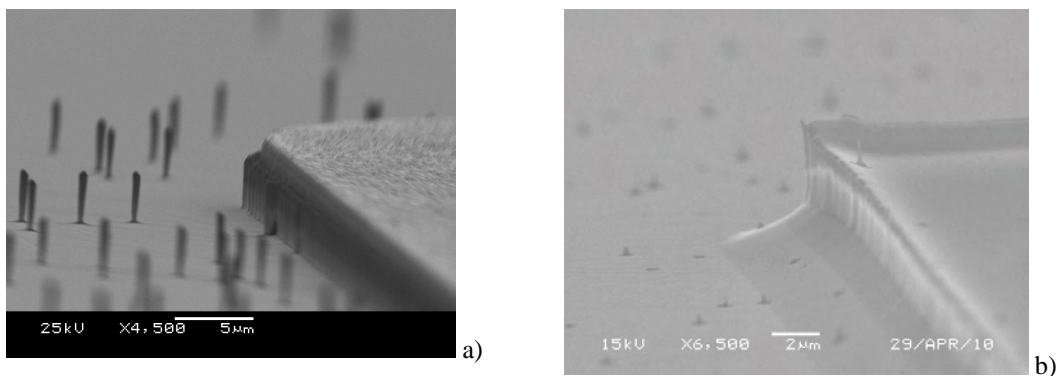
Fig. II.3.40 Exemples de micromasking produit par le dépôt de particules en provenance du masque à proximité du flanc gravé (a) ou de la cathode en aluminium (b) [RI37].
