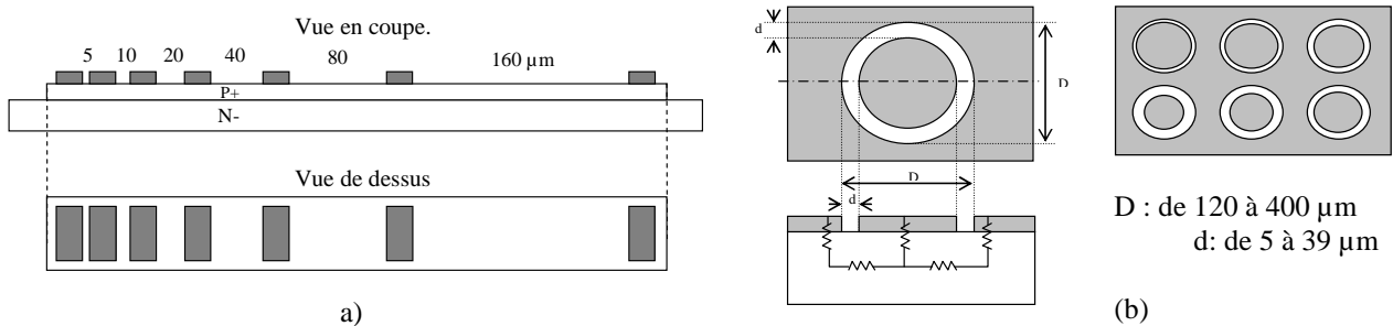
Fig. II.3.61 Structures de test utilisées: TLM mesa (a) et CTLM (b)
