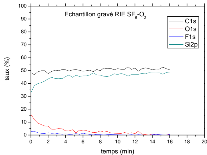
Fig. II.3.19 Analyse XPS d'une surface de SiC gravée par RIE montrant une contamination de fluor et oxygène
