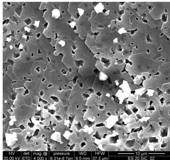
Fig. III.1.3. Cliché MEB de la surface d'une croissance VLS ancienne configuration sous gaz vecteur argon
