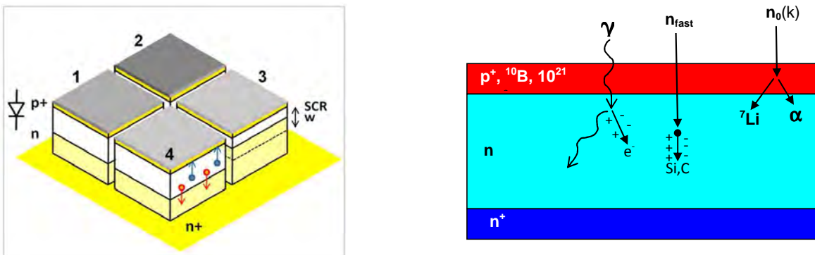
Fig. II.5.5 Schéma de principe du détecteur SiC multipixels proposé dans le cadre du projet ISMART (à gauche) et vue en coupe de la structure PiN utilisée (à droite).
