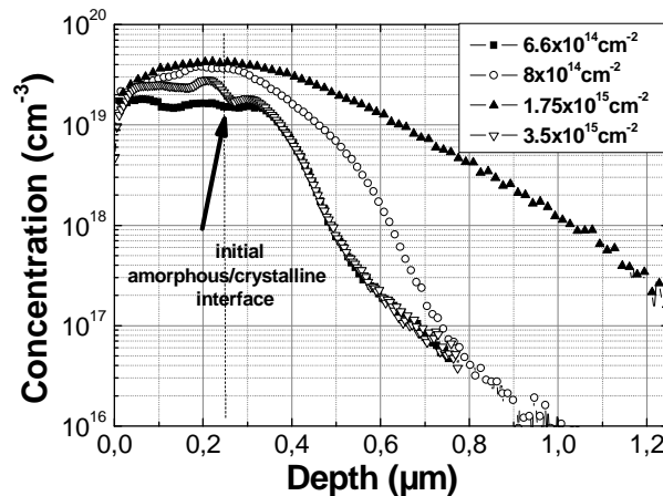
Fig. II.3.11 Mesures SIMS montrant la redistribution des dopants aluminium après recuit sur des couches SiC initialement amorphisées par des implantations aluminium à différentes doses [RI12]
