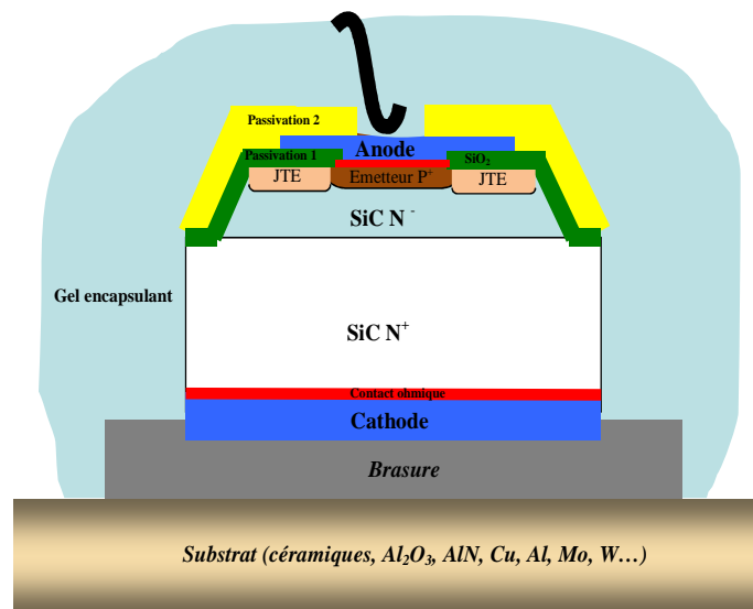
Fig. II.3.1 : Structure d'une diode PiN de puissance en SiC
