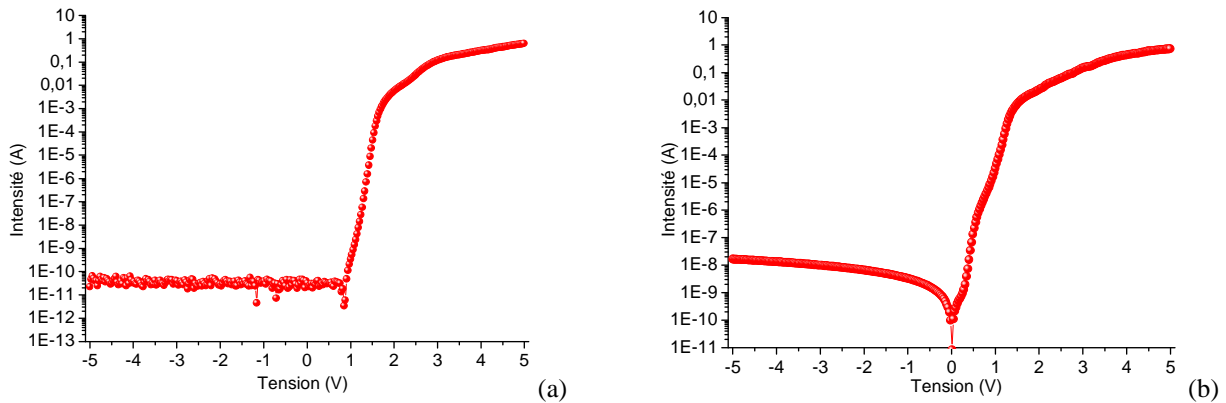
Figure II.3.81. Effet du recuit de métallisation Ni/Ti/Al/Ni sur les courants de fuites des PiN réalisés avec des couches VLS nouvelle configuration.
