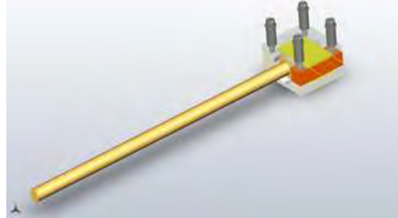
Fig.II.5.10 Structure du détecteur de neutrons rapides réalisé en SiC
