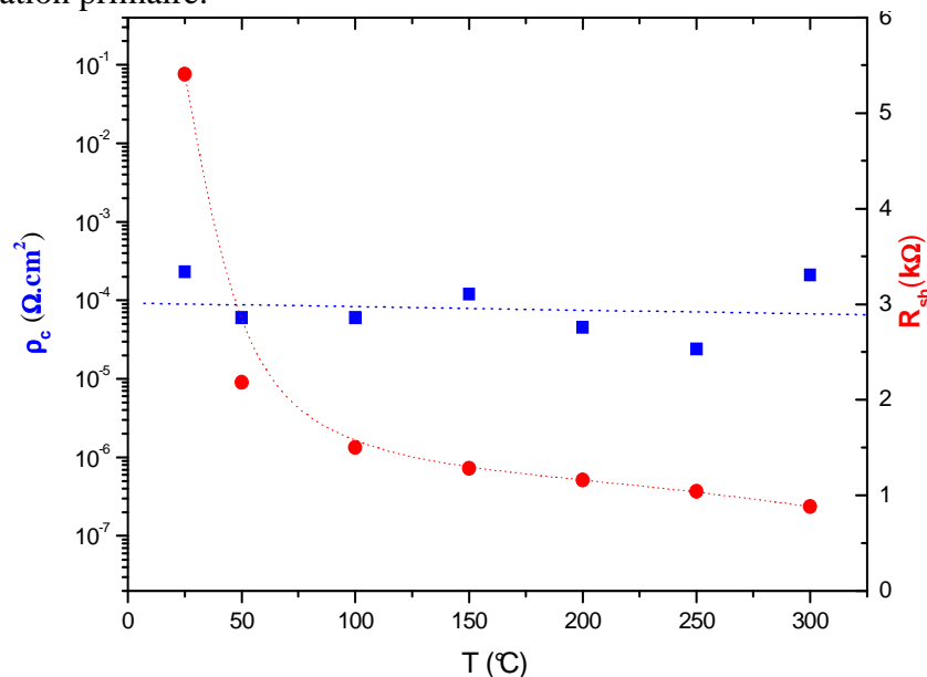
Fig.II.3.73 Dépendance des résistances carrées et spécifiques de contact durant le stress thermique pour des contacts Ni(10)/Ti(40)/Al(240)/Ni(10 nm) formés sur SiC après recuit à 800 °C sous argon 1atm.
