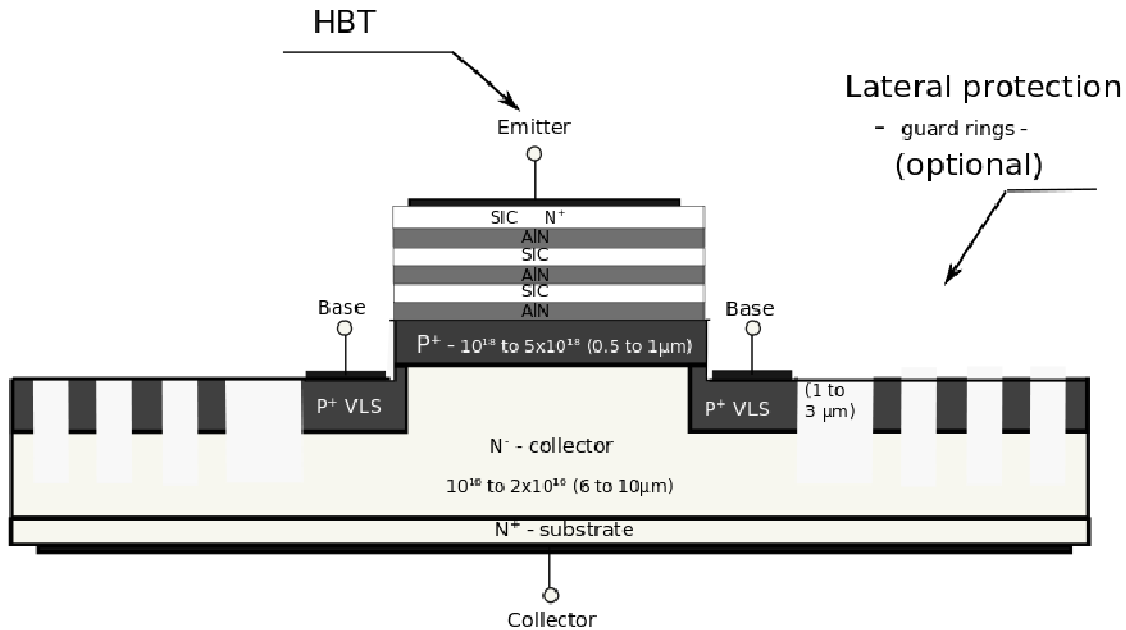
Fig. II.6.4 Structure verticale d'un HBT sur SiC que nous avons envisagé en 2014 avec le laboratoire LMI lors du dépôt du projet ANR Excelsic.
