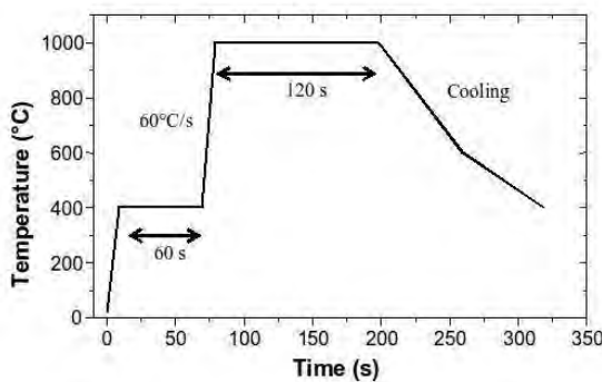
Figure II.3.62 Profil du recuit thermique sur les contacts Ni/Al [RI24].
