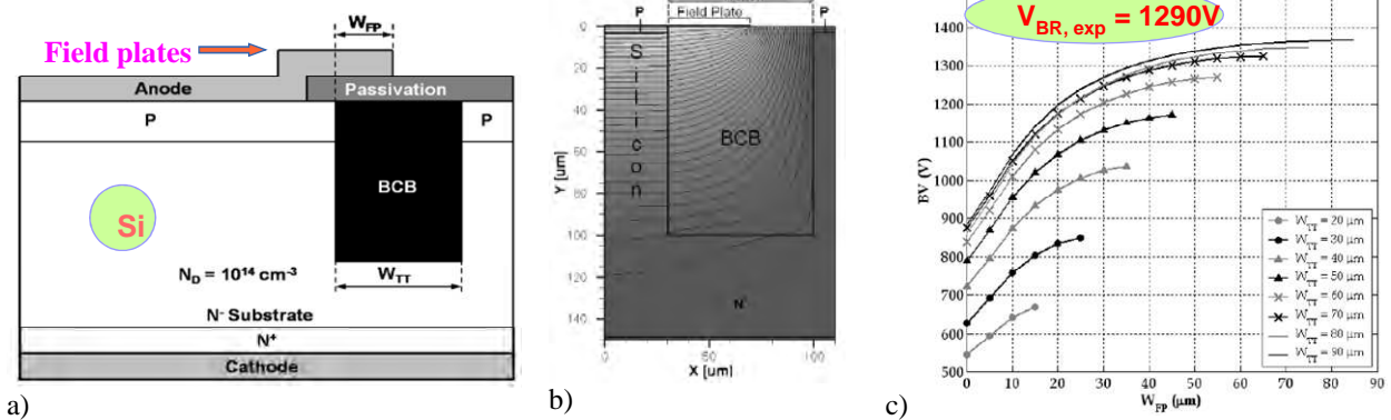
Fig. II.3.45 Diode verticale silicium conçue et fabriquée au LAAS validant le concept de protection périphérique DT^2 [Theo'08]. La DT^2 est gravée dans la couche faiblement dopée 10^{14} \text{ cm}^{-3} 520 \mu\text{m} et remplie de BCB (a). Répartition des équipotentielles sous polarisation inverse, simulation par éléments finis (b) Tenue en tension théorique versus le recouvrement de la plaque de champ et la largeur de la DT^2 (c)
