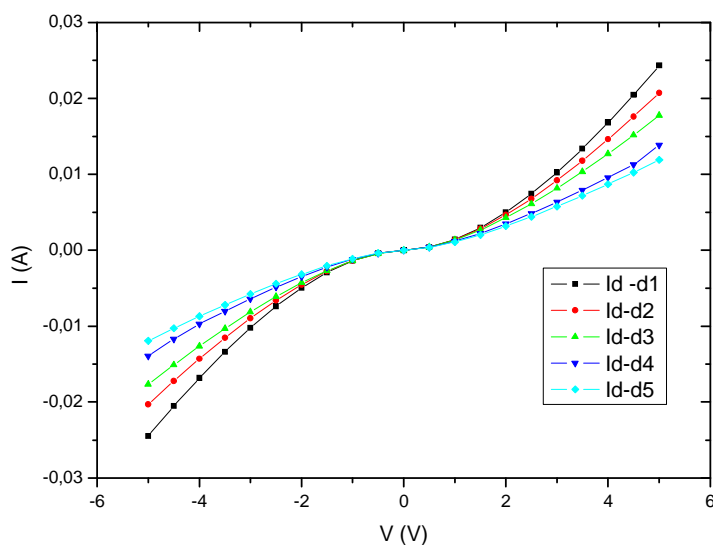
Figure II.3.82. Caractéristiques I-V obtenues entre des plots TLM créés sur une des couches VLS nouvelle configuration avec une métallisation aluminium 800 nm sans recuit.
