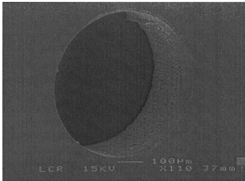
Fig. II.3.53. Image MEB d'une gravure d'un substrat complet de SiC de 300 µm [Chab'01].
