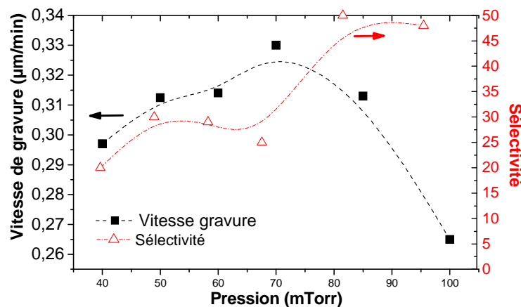
Fig. II.3.34 Influence de la pression de travail sur la cinétique de gravure et sur la sélectivité du masque nickel avec un plasma SF_6/O_2 (25sccm/6,7sccm) à une puissance de 250 W [CN6].
