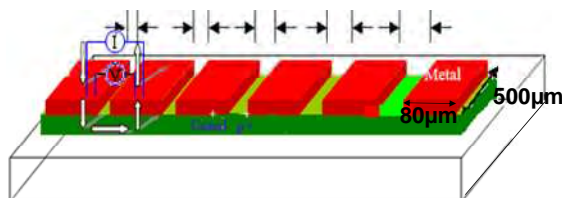
Fig. II.3.66 Structure TLMs avec un espacement entre les plots métalliques de 25, 35, 45, 55, 65 et 75 \mu\text{m} .
