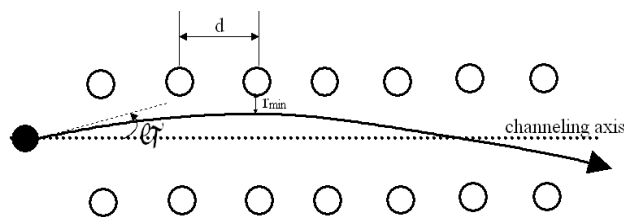
Fig. II.3.12 Présentation schématique d'un axe de canalisation lors de l'implantation ionique dans une structure cristalline
