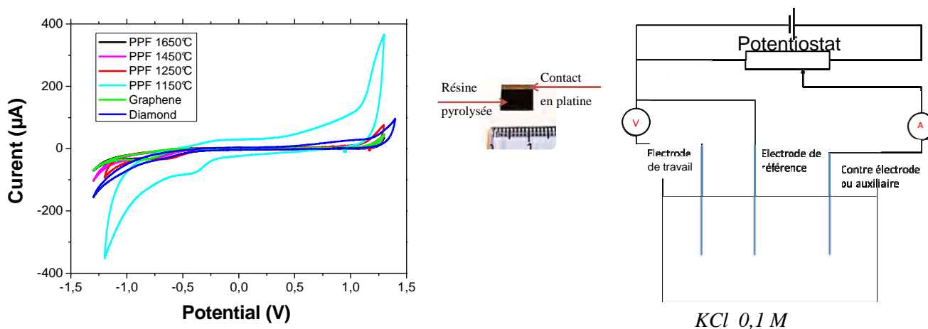
Fig.II.5.12 Domaine d'électroactivité par voltampérométrie avec 3 électrodes (carbonnée, Ag/AgCl, Pt)
