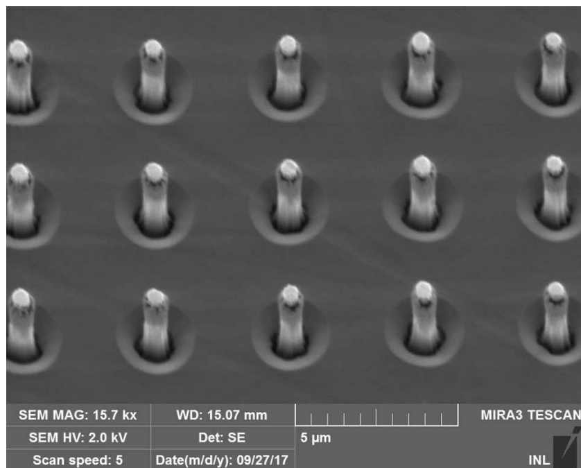
Fig.III.5.4: Surface structurée de SiC avec des piliers réalisés à Lyon en utilisant mes procédés de gravure plasma développés pour les composants SiC de puissance haute tension.
