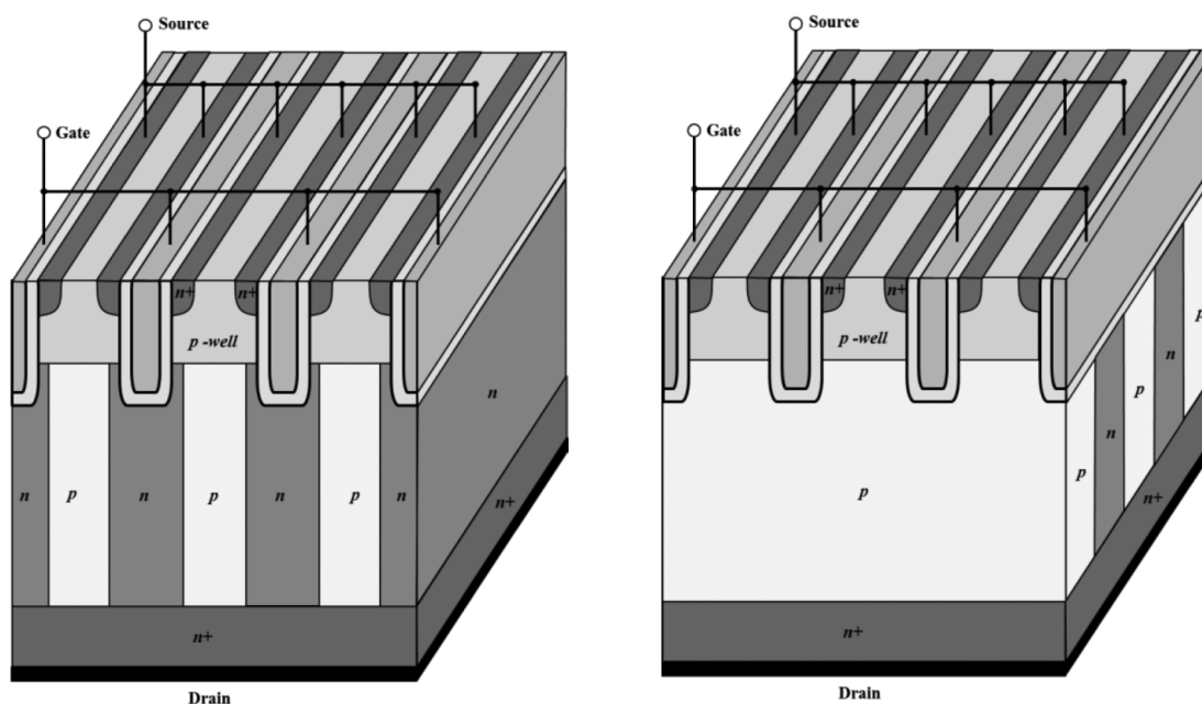
Fig. III.1.1. Présentation schématique 3D des structures des trench-MOSFET à super-jonctions (SJ) avec les couches SJ parallèles (à gauche) et perpendiculaires (à droite) aux tranchées du MOSFET
