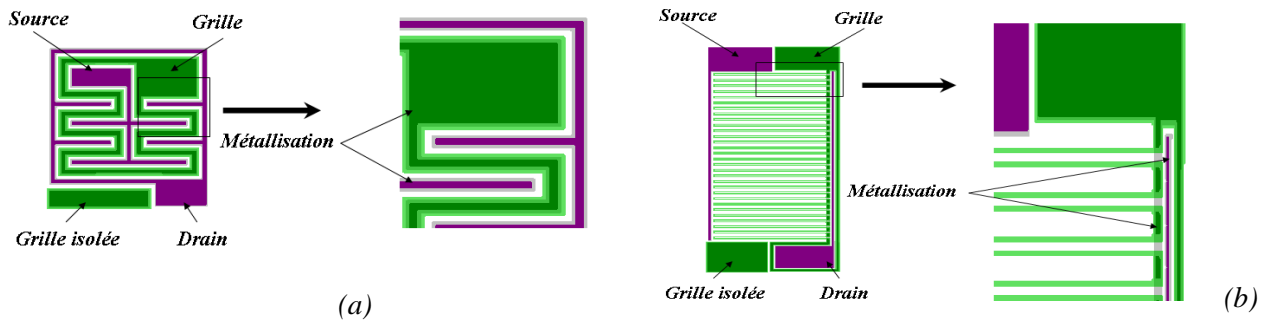
Fig II.4.12 Structure des JFET en serpentín avec une grille P^+ métallisée sur toute sa largeur (a) et structure en peigne avec une grille P^+ partiellement métallisée (b).
