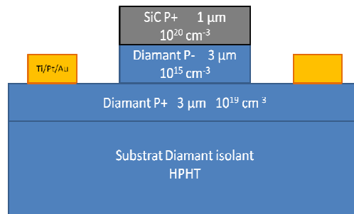
Fig. II.3.56. Présentation schématique de la diode verticale à hétérojonction SiC/Diamant que nous avons développée dans le cadre du projet ANR VLOC.
