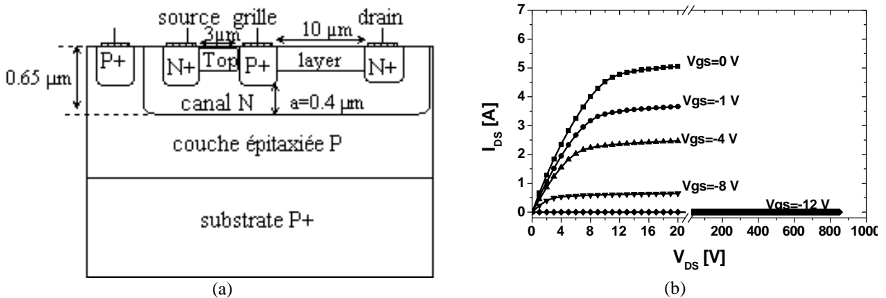
Figure II.4.4 La structure du LJFET à canal N (a) et ses caractéristiques électriques obtenues par simulation TCAD (b)
