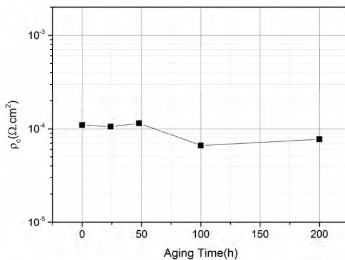
Figure II.3.77. Test de vieillissement à 600^\circ C des contacts Ti_3SiC_2 formés à 1000^\circ C . Evolution de la résistance spécifique de contact.
