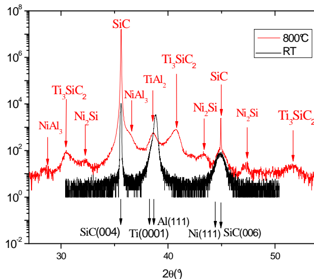
Fig.II.3.72: Analyses par diffraction X du contact Ni/Ti/Al/Ni avant et après le recuit à 800 °C.
