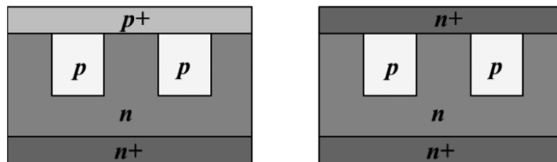
Fig. III.1.2. Diode (à gauche) et résistor (à droite) à superjonctions fabriqués par [Kosu'14]
