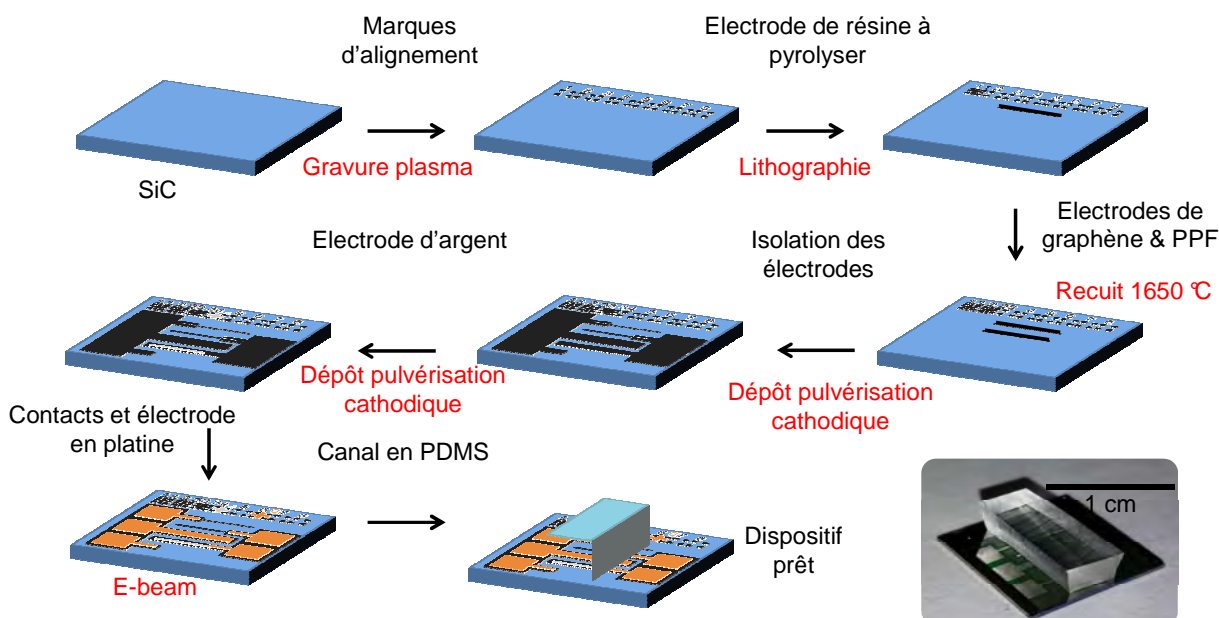
Fig. II.5.17 Enchaînement technologique pour l'intégration des électrodes PPF et graphène dans un dispositif microfluidique sur SiC.
