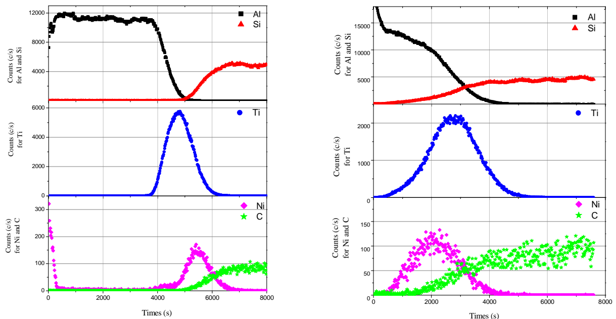
Fig. II.3.71 Analyses SIMS des contacts Ni/Ti/Al/Ni avant (à gauche) et après (à droite) le recuit à 800 °C.
