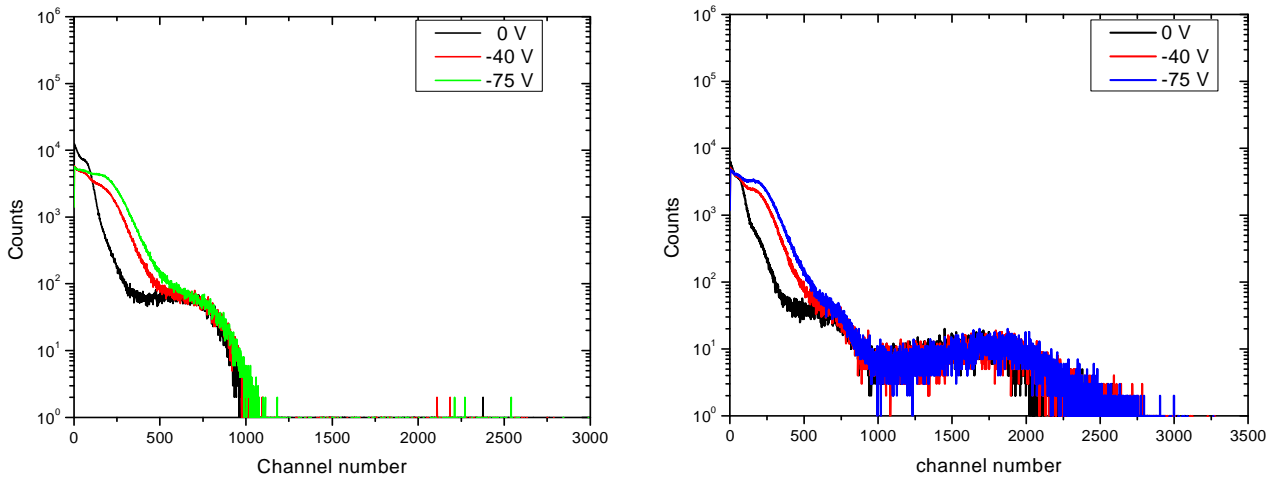
Fig. II.5.9 Mesures au SCK CEN avec des détecteurs sans (à gauche) et avec (à droite) couche active de ^{10}\text{B} .
