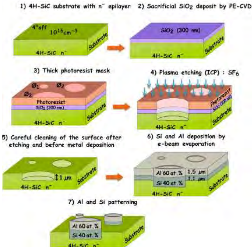
Fig. II.3.24. Enchaînement des étapes technologiques pour la définition des empilements Al/Si avant la croissance VLS [RI84].
