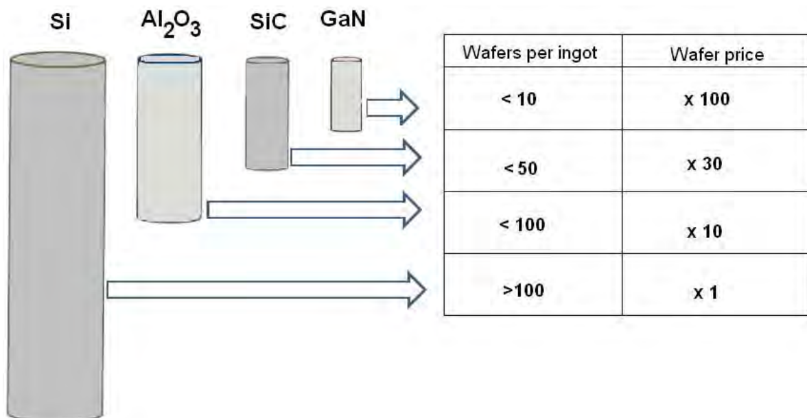
Fig. II.2.5 : Présentation schématique des hauteurs des "lingots" de croissance en Si, \text{Al}_2\text{O}_3 , SiC et GaN avec le nombre de wafers obtenus après sciage et leurs coûts [Amor'15].
