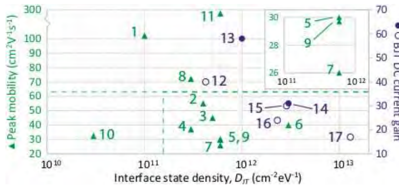
Fig. III.3.2 Synthèse des mobilités dans les canaux d'inversion des MOSFET et des gains des BJT [Sidd'16].
