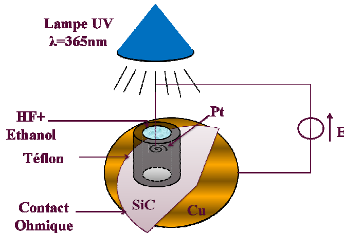
Fig. II.3.54. Banc expérimental de porosification du silicium sur la plateforme Nanolyon de l'INSA.
