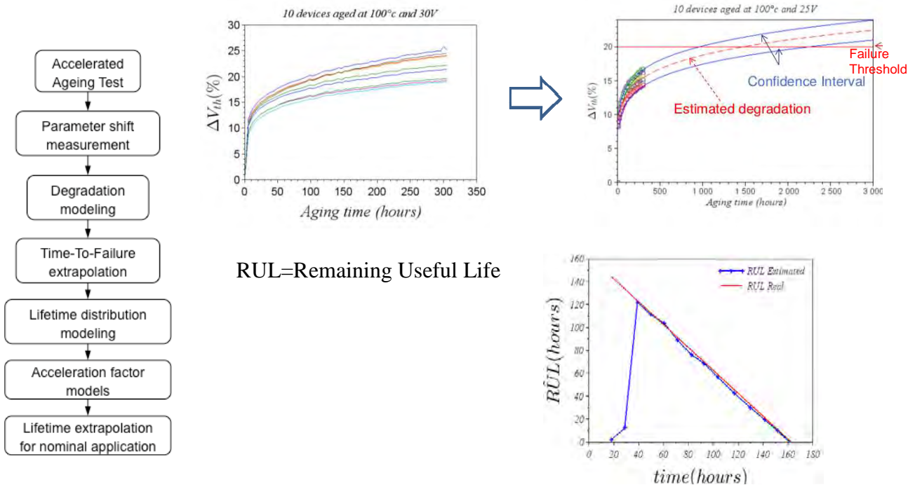
Fig. III.2.1 : Démarche et résultats sur la prédiction du temps de vie des composants MOSFET SiC [Sant'16].
