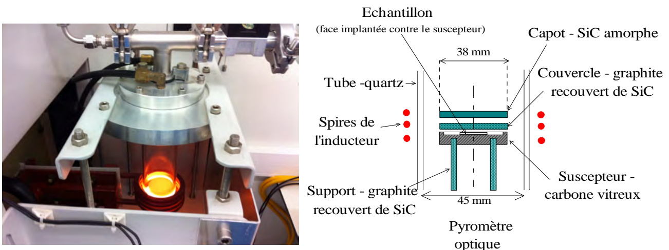
Fig. II.3.4 : Image de la partie chauffante du four à induction JIPELEC du laboratoire, dédié au recuit SiC post-implantation (à gauche) et la présentation schématique du port-substrat (à droite).
