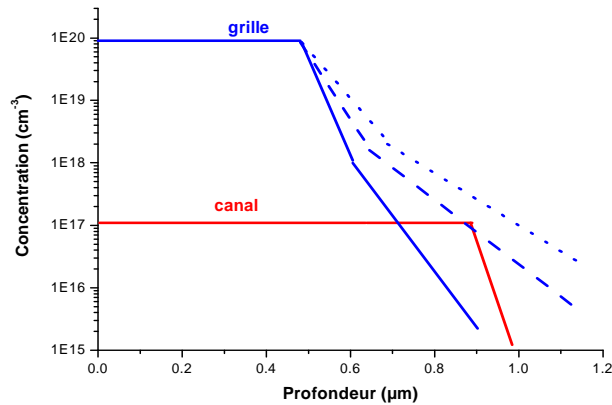
Fig II.4.10. Présentation schématique du profil du canal caché par la queue de canalisation de l'implantation de la grille en surface.
