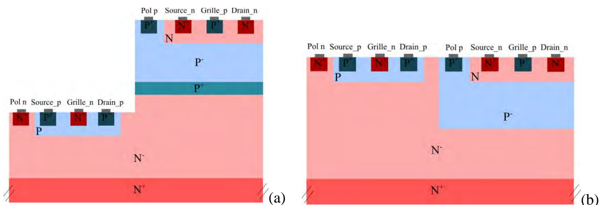
Fig. II.4.11 Structure du bras puissance de l'onduleur monolithique gravé (a) et planar (b) avec les JFET P et N intégrés sur le même substrat.
