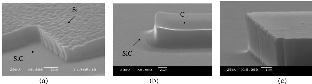
Fig. II.3.42. Surfaces de SiC-4H gravées en utilisant des masques en silicium (a), carbone (b) et nickel (c). Dans le cas du silicium et carbone, les masques sont encore présents en haut des flancs SiC gravés [RI37].
