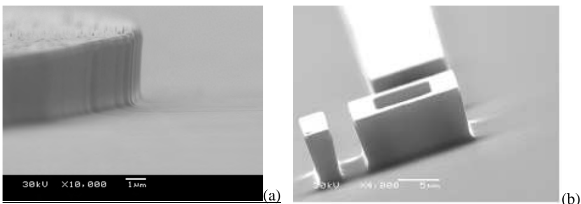
Fig. II.3.38 : Micrographies MEB sur des échantillons SiC-4H gravés avec un plasma 25 sccm SF_6 et 6,7 sccm O_2 à (a) 250 W, 60 mTorr, 10 min et (b) 250 W, 60 mTorr, 20 min.
