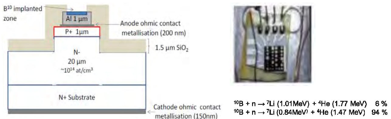
Fig. II.5.7 Structure du détecteur de neutrons thermiques réalisé en SiC et les réactions nucléaires qui y réagissent
