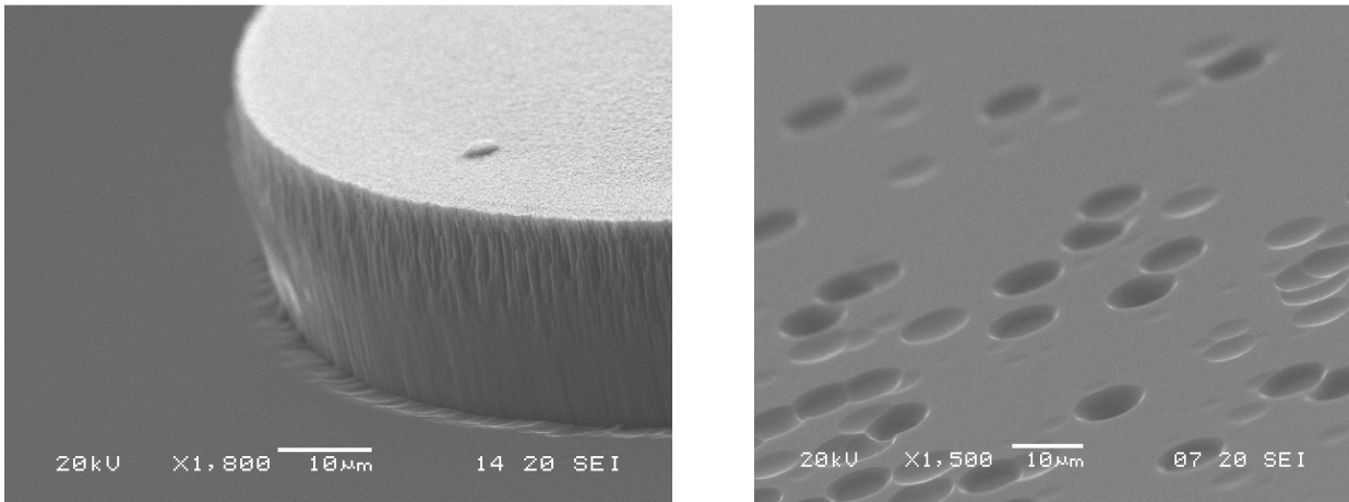
Fig. II.3.50 Images prises au MEB des parois gravées en SiC ainsi que sur une zone révélatrice des défauts dans le substrat après gravure.
