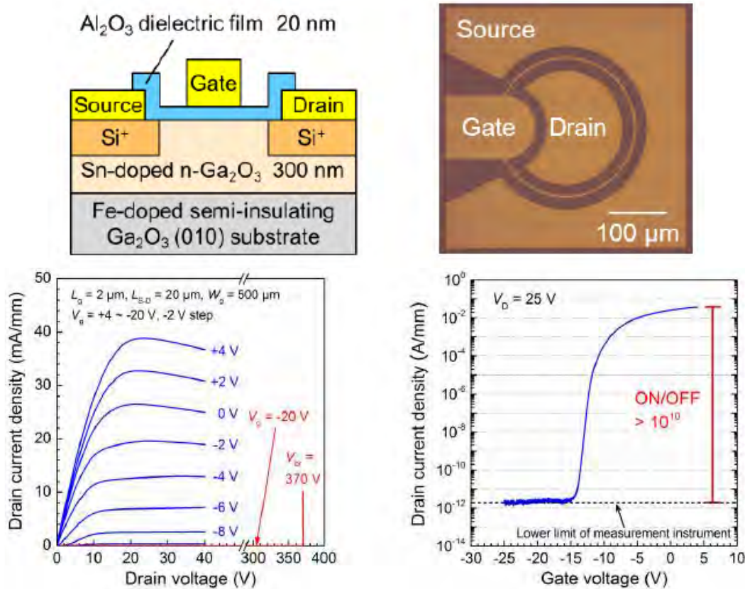
Fig. III.6.3 MOSFET \text{Ga}_2\text{O}_3 : structure en coupe et vue de dessus (en haut), caractéristiques électriques (en bas) [NICT'13].
