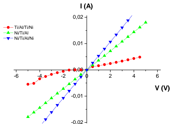
Figure II.3.69. Caractéristiques I-V typiques obtenues entre les plots TLM pour les trois familles de métallisations.
