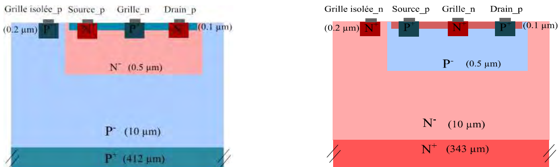
Fig II.4.9 : Vue en coupe des transistors JFET 600V complémentaires de l'étage de puissance du bras d'onduleur à canal n (à gauche) et à canal p (à droite).
