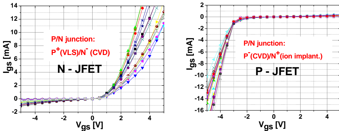
Fig. II.4.19. Caractéristiques I_{gs} - V_{gs} des transistors N-JFET et P JFET
