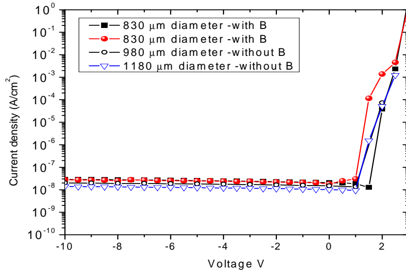
Fig.II.5.8 Caractéristiques I-V en inverse des diodes avant et après implantation de ^{10}\text{B} dans la couche de métallisation de l'anode
