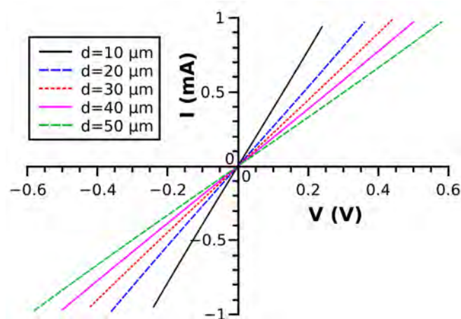
Figure II.3.79. Caractéristiques I-V linéaires obtenues entre les plots TLM créés sur une des couches VLS. Les couches Ni/Ti/Al/Ni pour former les contacts ont été déposées sans recuit.
