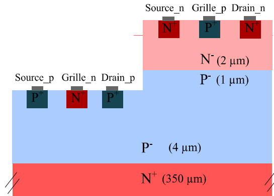
Fig.II.4.13 : Vue en coupe du bras d'onduleur fabriqué pour l'étage commande avec les structures des JFET basse tension à canal N et P intégrées monolithiquement.
