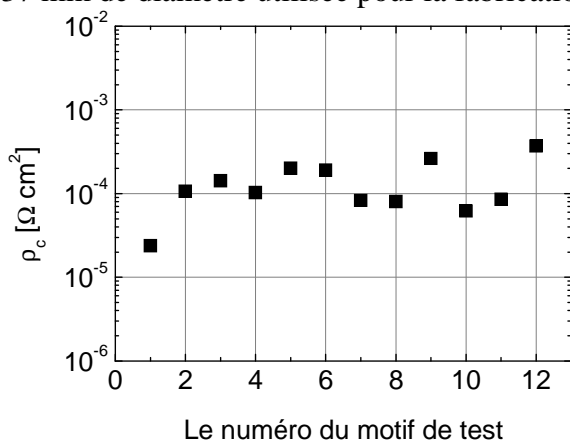
Figure II.3.59 : Résistances de contacts spécifiques mesurées sur les motifs de test des contacts Al/Ti réalisés sur une plaque SiC-4H avec des diodes PiN 5 kV
