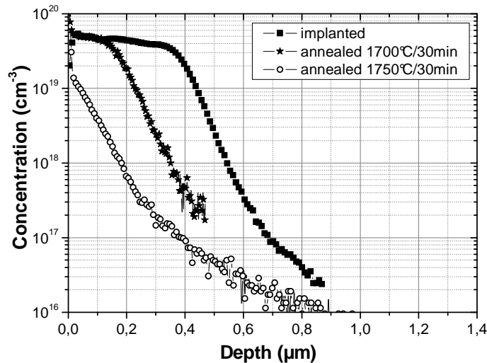
Fig. II.3.7 : Pertes des dopants Al identifiées par des mesures SIMS des surfaces SiC implantées avant et après recuit post-implantation.
