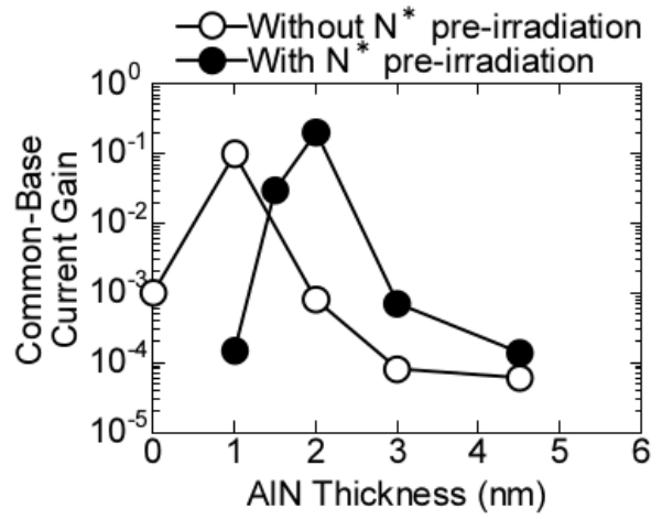
Fig. III.6.6. HBT GaN/SiC fabriqué par Miyake et al. en 2012, ainsi que les caractéristiques électriques obtenues. Influence de la couche tampon d'AlN présente entre le GaN et le SiC.
