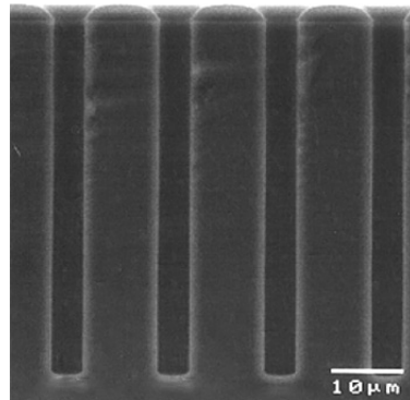
Fig. III.1.4. Des trous via créés dans le Si par gravure DRIE cryogénique ou procédé Bosch
