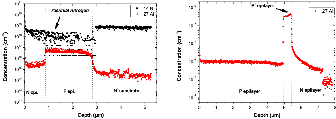
Fig.II.4.14. Profils des dopages aluminium et azote mesurés par SIMS pour les couches épitaxiales CVD utilisées dans les structures de l'étage de puissance (à gauche) et de commande (à droite).
