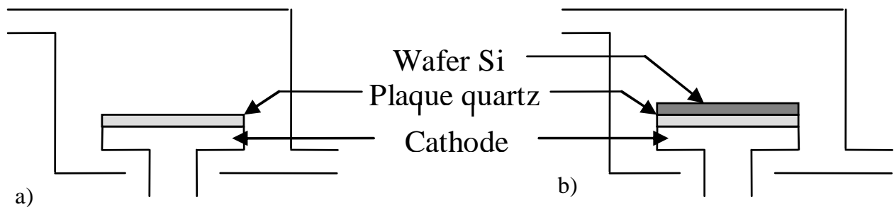
Fig. II.3.32 Configuration du réacteur RIE avec une cathode en quartz (a) et recouverte d'un wafer de silicium (b) [CN6]
