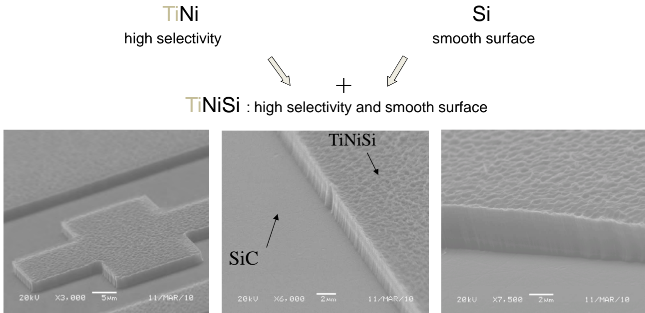
Fig. II.3.43. Schéma du concept des masques TiNiSi (en haut). Analyses MEB avant retrait des masques TiNiSi montrant l'état des surfaces de SiC-4H gravées (en bas).
