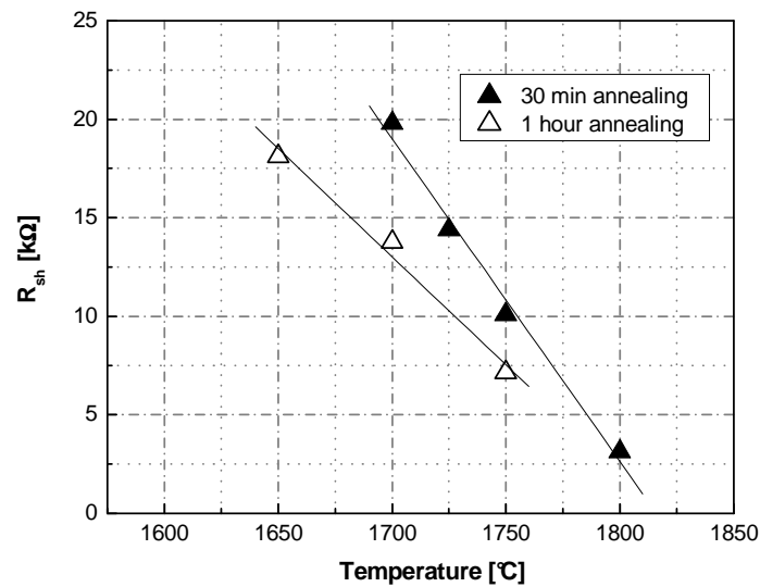
Fig. II.3.5 : Variation des résistances carrées des couches type p créées par implantation ionique d'aluminium avec la température et la durée du recuit post-implantation [RI9].
