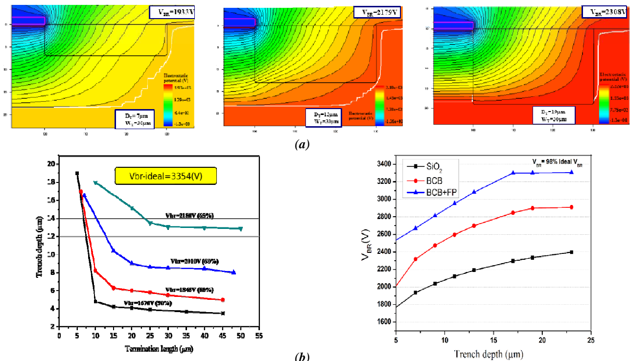
Fig II.3.48 : Résultats des simulations TCAD : répartition des équipotentielles sous polarisation inverse pour 3 profondeurs des tranchées gravées : 7, 13 et 19 \mu\text{m} (a) et tenue en tension estimée en faisant varier différents paramètres technologiques : profondeur et largeur des tranchées gravées, remplissage avec différents isolants, utilisation d'une plaque de champ (b).
