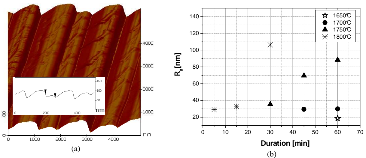
Fig. II.3.6 : Marches mesurées en AFM dues à une rugosification de la surface du SiC après recuit post-implantation (a) évolution en fonction de la température et du temps de recuit des valeurs des rugosités moyennes ( R_a ) quantifiées par des mesures de profilométrie avec un alpha-step stylus Dektak Veeco (b)
