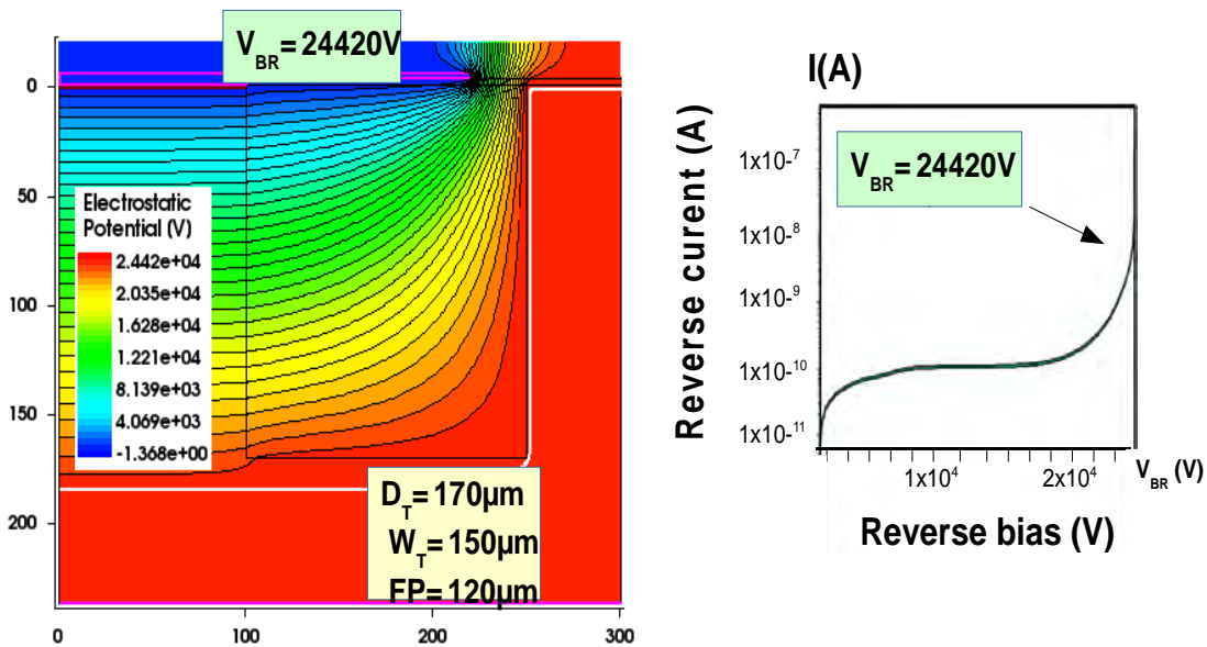
Fig II.3.52 : Simulation TCAD Sentaurus d'une structure d'un composant SiC 25 kV avec une protection périphérique verticale DT 2 nécessitant une gravure de plus de 170µm.
