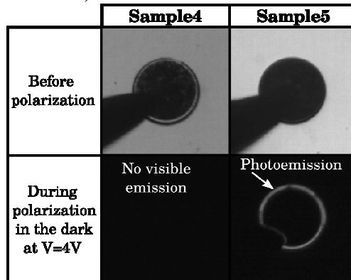
Fig. II.3.22. Effet du recuit à 1700 °C sur l'électroluminescence des diodes p + /n dont la couche p + a été réalisée par croissance VLS. Uniquement l'échantillon n°5 a subi le recuit à 1700 °C post croissance VLS.
