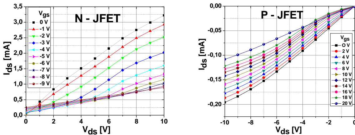
Fig. II.4.18. Caractéristiques électriques typiques des transistors N-JFET et P-JFET avec des caissons P + réalisés par VLS.
