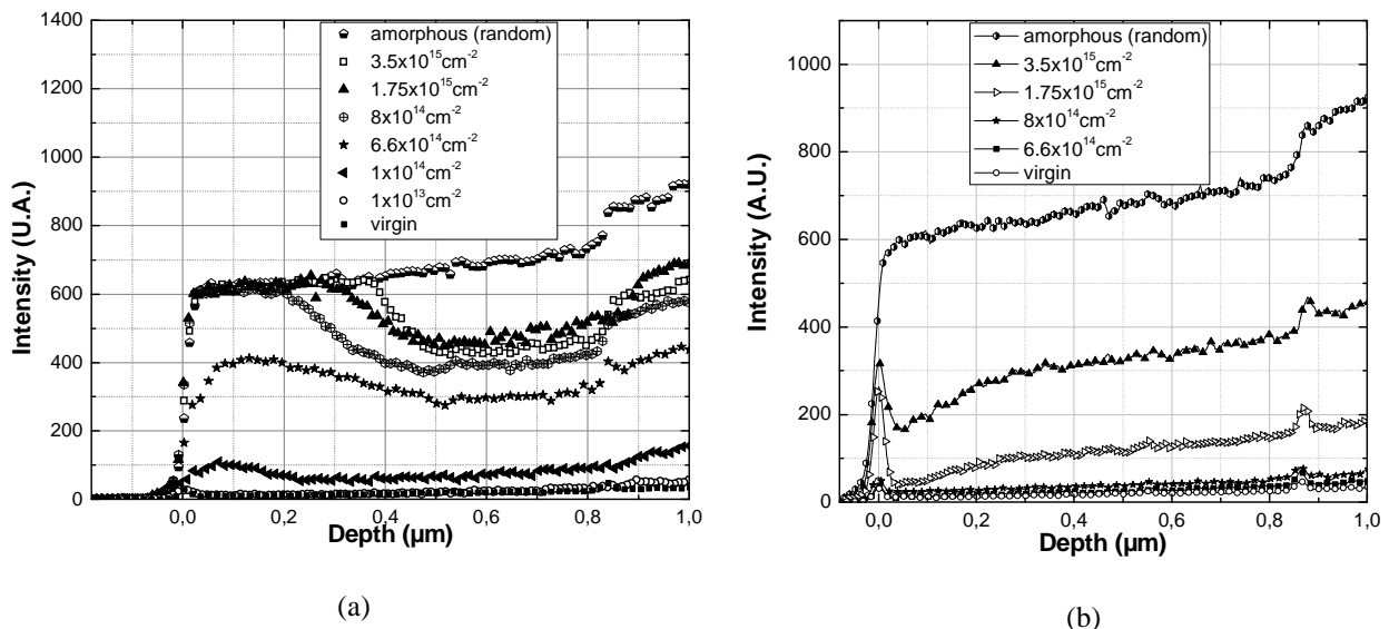
Fig. II.3.10 Analyses RBS/C de couches implantées Al à différentes doses juste après implantation (a) et après recuit post-implantation 1700°C/30 min (b)
