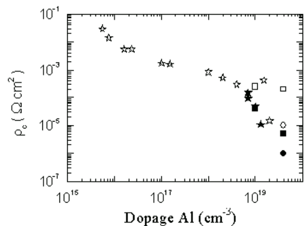
Figure II.3.60 : Résistances spécifiques de contact sur SiC-4H (ronds) et SiC-6H (carrés) mesurées à température ambiante (ouverts) et à 290°C (pleins) comparées à [Crof'02] (étoile)
