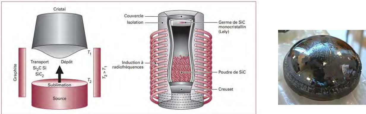
Fig. II.2.4 : Schéma d'un bâti de croissance du SiC par la méthode de Lely modifiée (à gauche). Image d'une boule de SiC obtenue (à droite).
