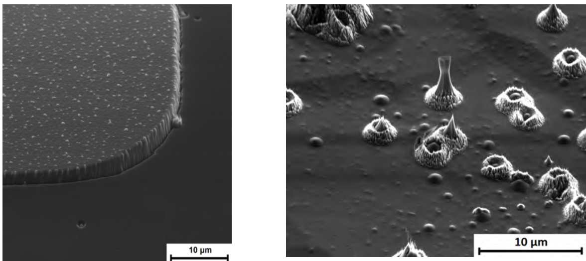
Fig. II.3.57. Images MEB présentant des surfaces de diamant gravées par plasma jusqu'à 2,5 µm à gauche (masque Al encore présent) et jusqu'à 9 µm à droite avec un zoom sur les défauts en fond de gravure.
