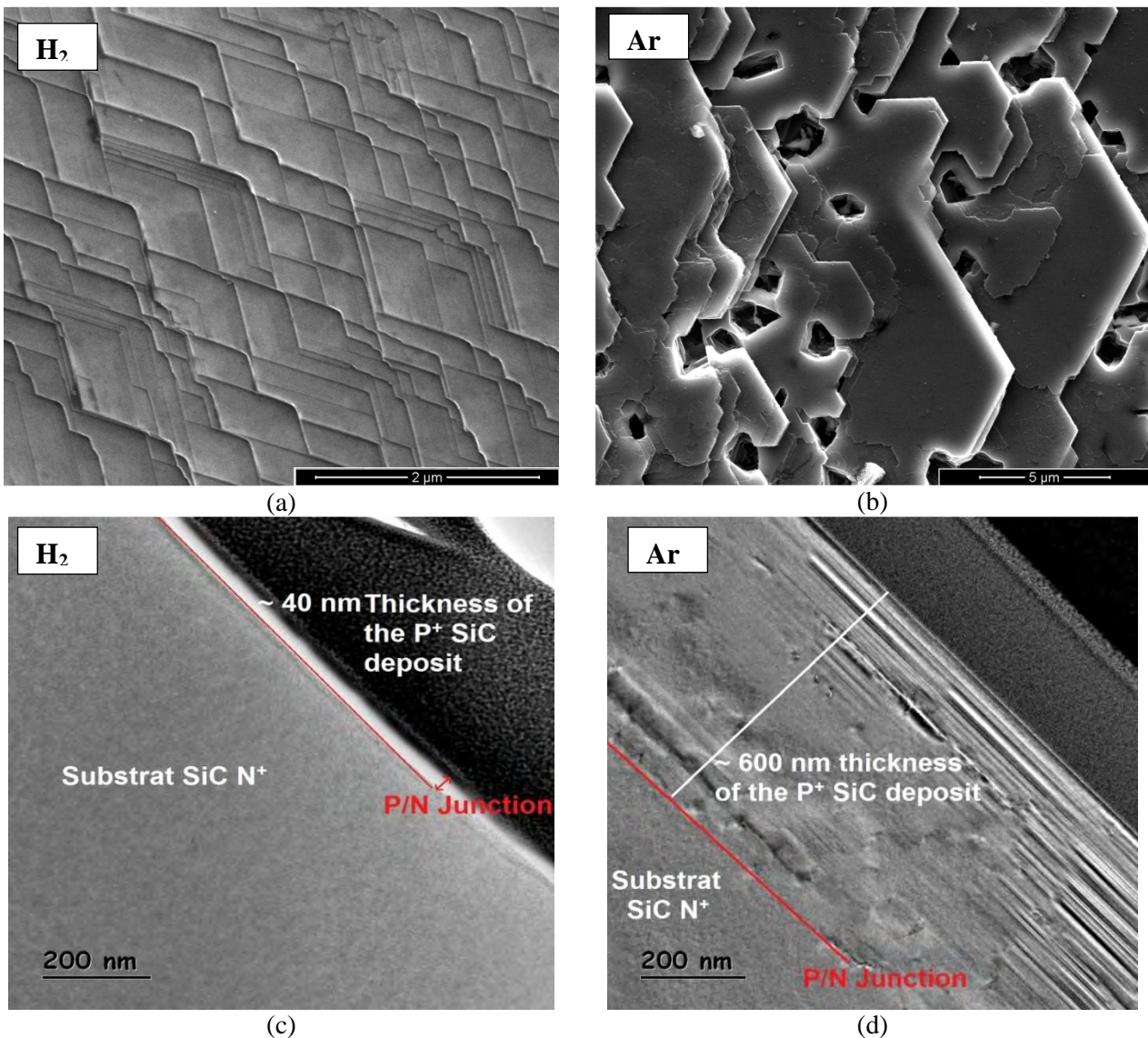
Fig. II.3.25. Clichés MEB (a et b) et MET (c et d) montrant la morphologie de surface et volumique de couches VLS obtenues avec un gaz vecteur H_2 (a et c) ou argon (b et d) [RI79].
