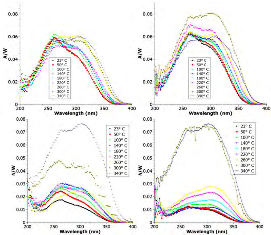
Fig. II.5.3 Réponses spectrales des photodétecteurs UV réalisés par dopage aluminium (en haut) et bore (en bas) et mesurées en températures croissantes et décroissantes
