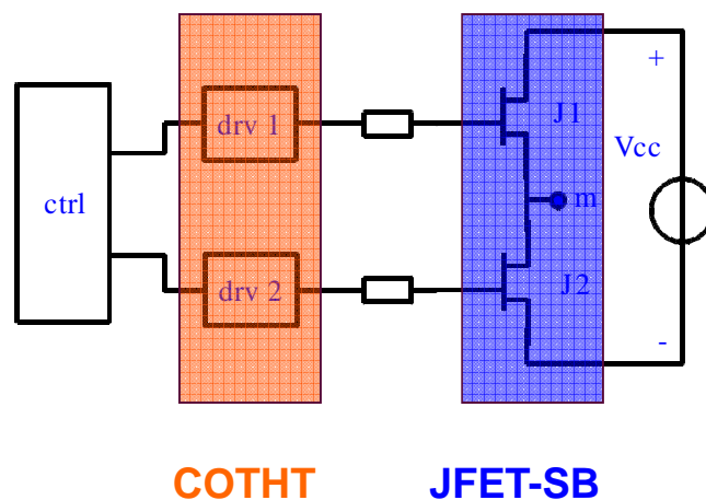
Fig II.4.1 : Schéma d'un onduleur avec les deux étages commande (COTHT) et puissance (JFET-SB)
