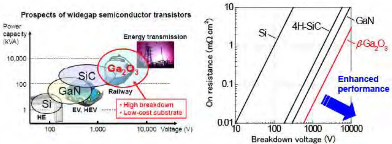
Fig.III.6.1: Applications potentielles pour l'électronique de puissance (à gauche) et limites de performances théoriques (à droite) du \text{Ga}_2\text{O}_3 comparés aux SiC, GaN et silicium [NICT'13].
