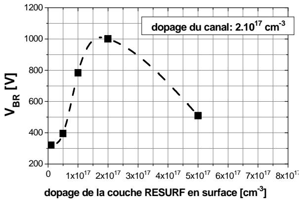
Fig. II.4.6 Variation de la tenue en tension avec le dopage de la couche RESURF en surface
