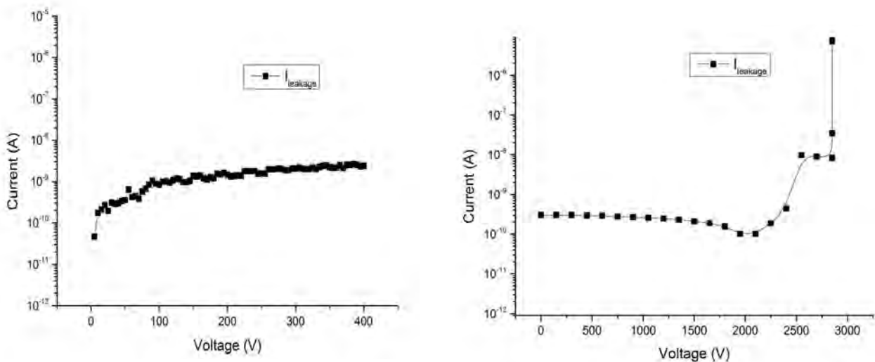
Fig. II.3.5 Mesures électriques montrant un faible courant de fuite et validant la tenue en tension des diodes avec la protection DT 2 . A gauche sans remplissage des tranchées, à droite après remplissage avec une couche diélectrique en parylène. La largeur de la tranchée est de 200 μm et la taille d'une diode 400 μm.
