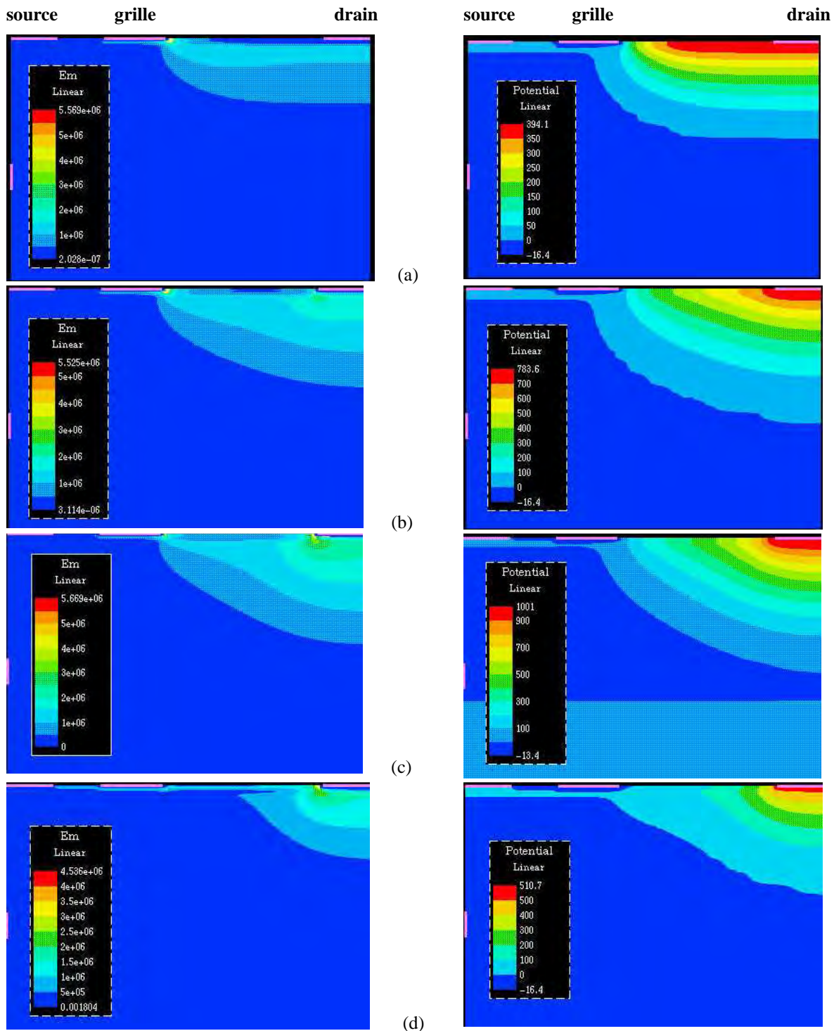
Fig. II.4.5: Répartition du champ électrique (à gauche) et des équipotentielles (à droite) dans le JFET à canal N pour 4 différents dopages de la couche RESURF en surface de type p: 5 \times 10^{16} \text{ cm}^{-3} (a), 1 \times 10^{17} \text{ cm}^{-3} (b), 2 \times 10^{17} \text{ cm}^{-3} (c) et 5 \times 10^{17} \text{ cm}^{-3} (d).
