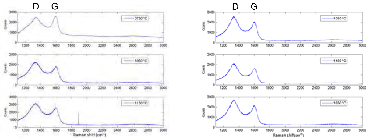
Fig. II.5.15. Analyses \mu -Raman des couches PPF en fonction de la température de recuit.
