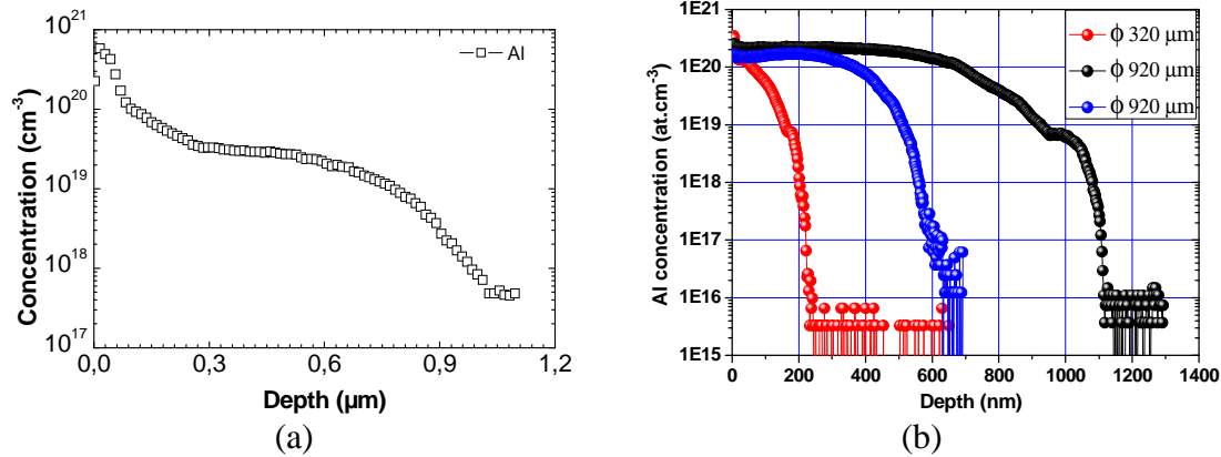
Fig. II.3.18 Profils d'Al obtenus par analyses SIMS de couches SiC type p réalisées par croissance VLS localisée en configuration sans caissons gravés (a) et avec caissons gravés (b) à la surface du SiC.
