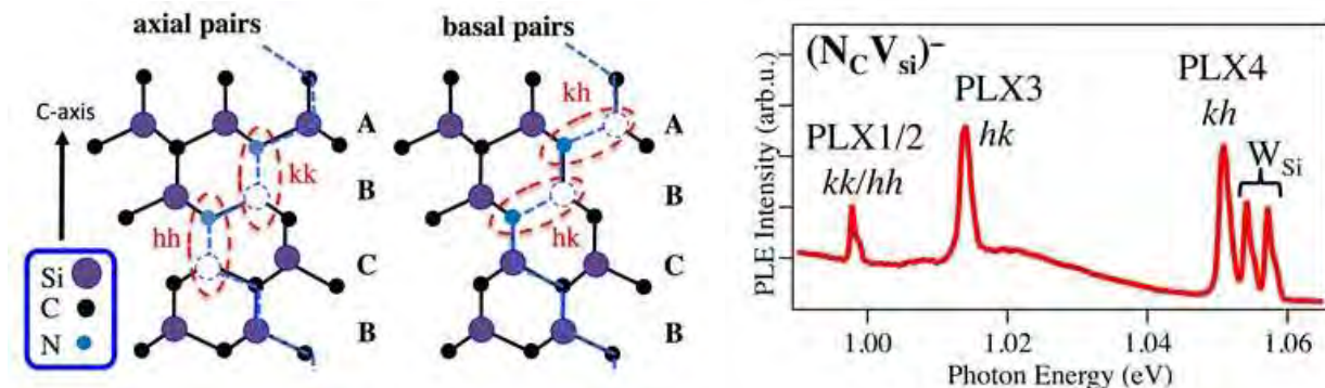
Fig.III.5.1 : Défaut N_C V_{Si} dans le réseau hexagonal du 4H-SiC (à gauche) et photoluminescence de ce défaut (à droite) [Zarg'16].
