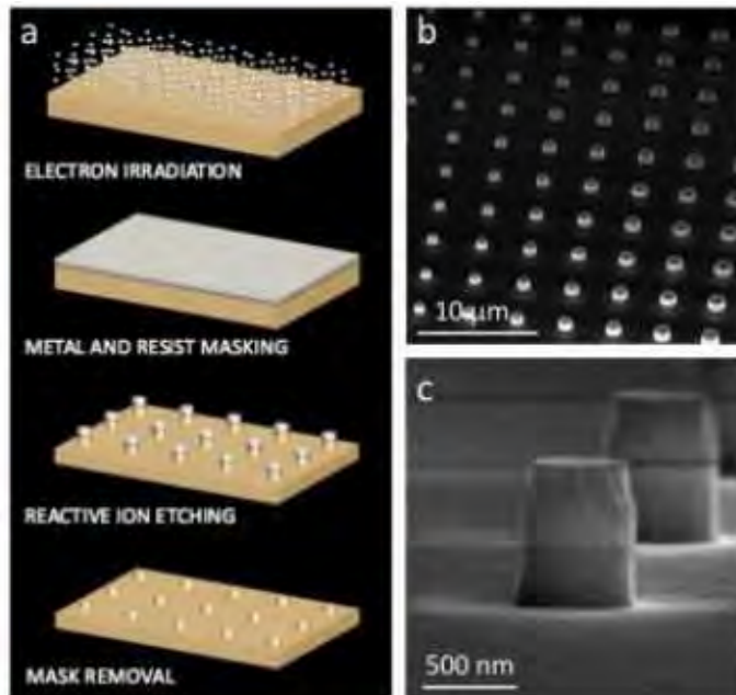
Fig.III.5.3 : Procédé technologique des structures de nanopiliers dans une surface SiC ou des centres colorés ont été créés préalablement par irradiation électronique. Images MEB des piliers formés [Radu'17].
