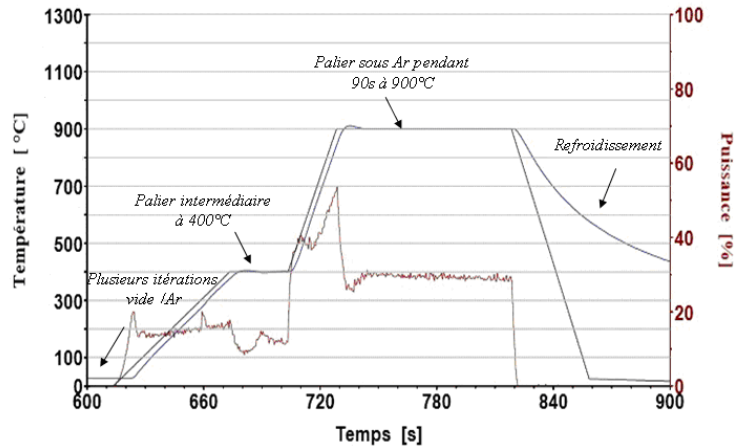
Figure II.3.68. Profil typique d'un recuit de métallisation à 900 °C pendant 90 s avec 2 paliers.
