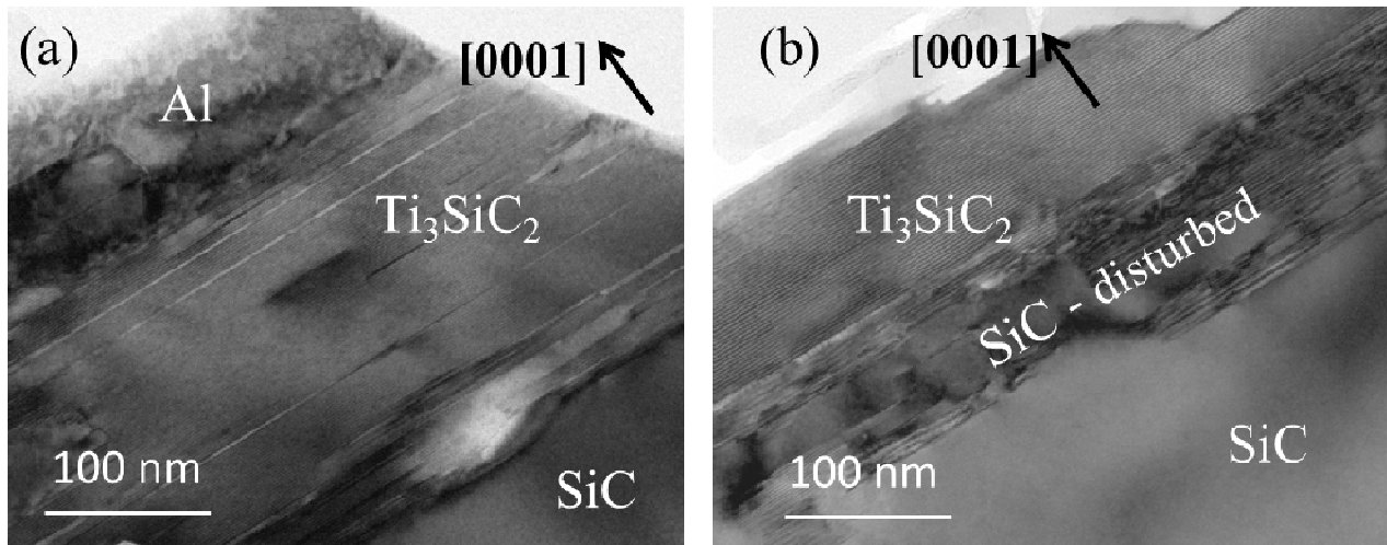
Figure II.3.76. Clichés XTEM-BF des contacts obtenus avec des alliages Ti_{30}Al_{70} sur SiC montrant la formation du Ti_3SiC_2 épitaxial après un recuit à 1000^\circ C (a) et 1200^\circ C (b)
