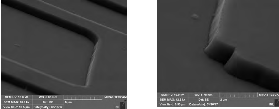
Fig. II.3.23 Images MEB montrant l'aspect des flancs et les surfaces de SiC après gravure ICP
