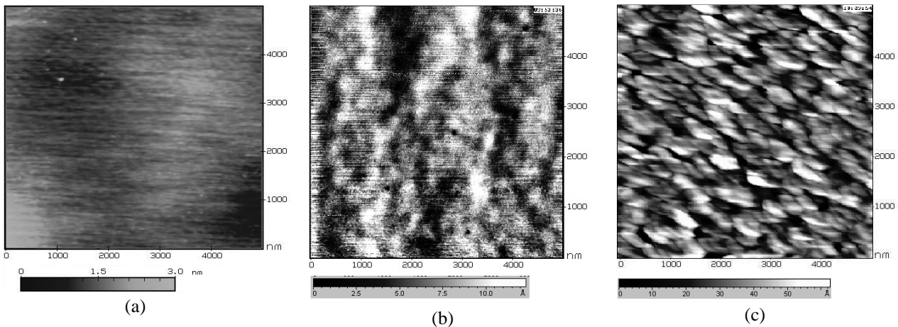
Fig. II.3.9 Images AFM 5 \times 5 \mu\text{m}^2 pour un échantillon vierge (a), implanté aluminium avec une dose de 1,75 \times 10^{15} \text{cm}^{-2} et recuit à 1800°C/30 min avec C-cap (b), implanté aluminium avec une dose de 3,5 \times 10^{15} \text{cm}^{-2} après un recuit à 1800°C/30 min avec C cap (c).
