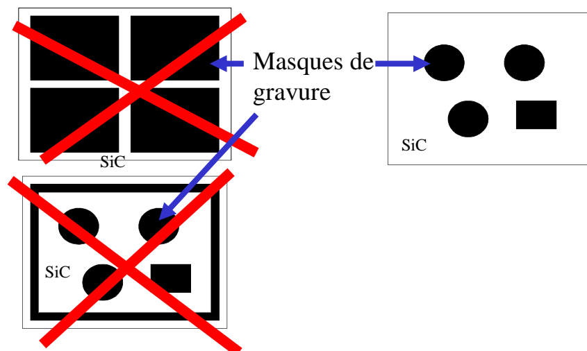
Fig. II.3.41 Design des masques pour éviter le phénomène de micromasking [CN6]
