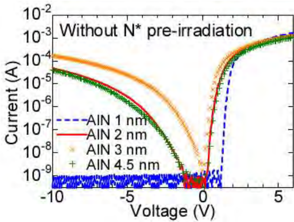
Fig. III.6.6. HBT GaN/SiC fabriqué par Miyake et al. en 2012, ainsi que les caractéristiques électriques obtenues. Influence de la couche tampon d'AlN présente entre le GaN et le SiC.
