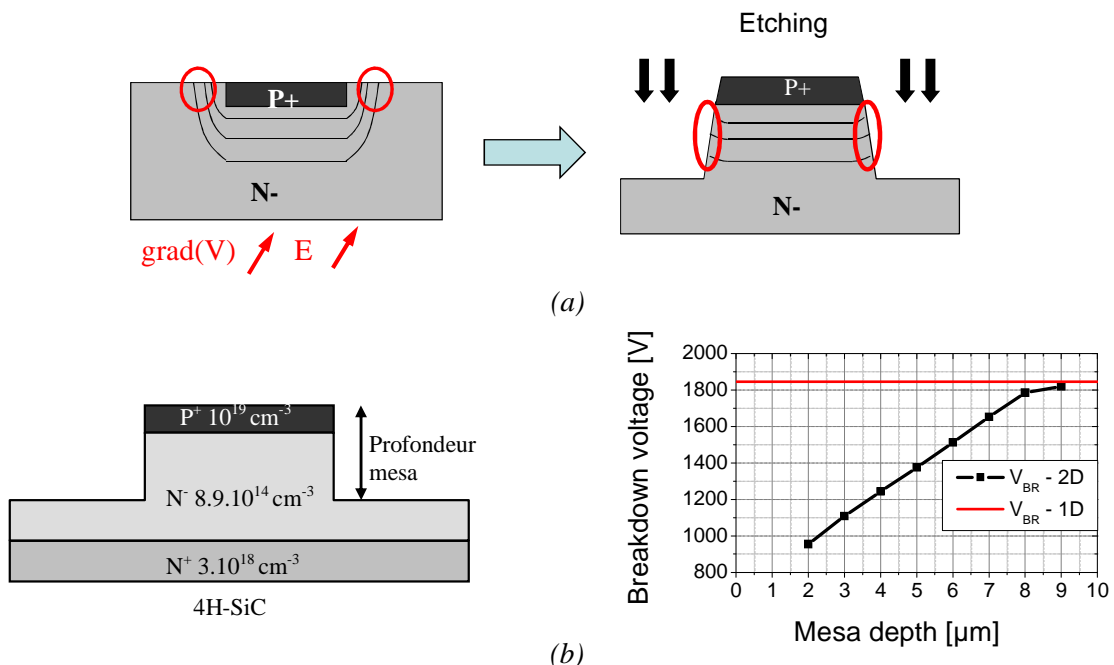
Fig. II.3.30 Protection périphérique mesa d'un composant de puissance vertical. Retrait par gravure des zones à fort champ ou resserrement des équipotentielles (a). Tenue en tension en fonction de la profondeur de gravure pour une diode SiC, résultats obtenus avec le simulateur par éléments finis MEDICI (b) [CN6].
