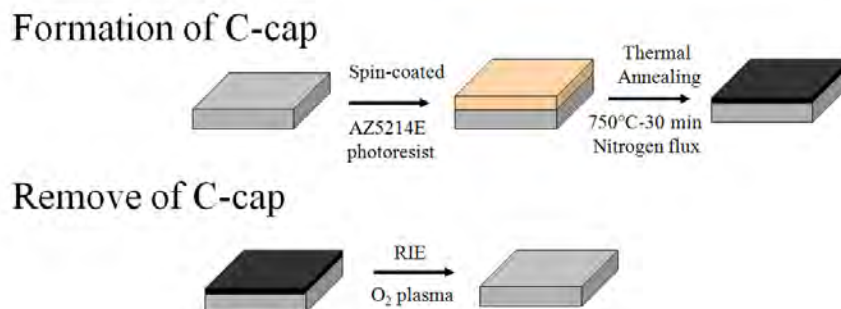
Fig. II.3.8 : Procédé d'encapsulation de la surface des plaquettes SiC avec de la résine pyrolysée et son retrait après le recuit post-implantation.
