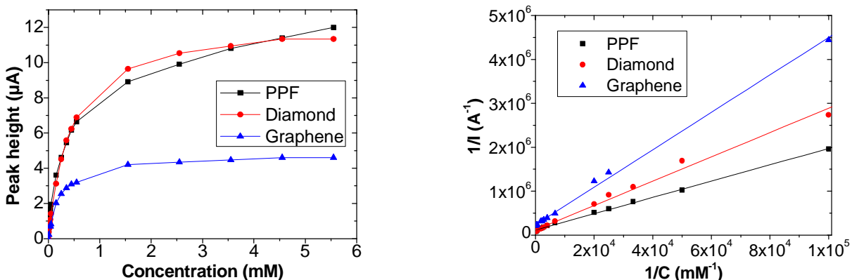
Fig. II.5.16 Courbes de calibration Michaelis-Menten (à gauche) et Lineweaver Burk (à droite) pour nos électrodes carbonées utilisées comme biocapteurs pour la détection de l'acetylthiocholine.
