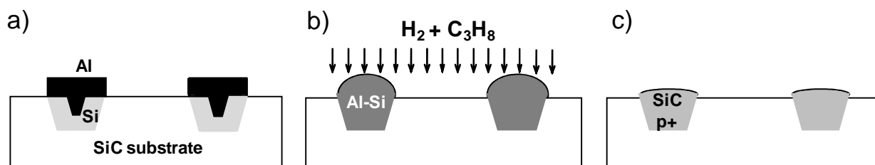
Fig. II.3.15 Schéma représentant les trois étapes de la croissance localisée de SiC dopé aluminium de type p par transport VLS: dépôt de couches de silicium et aluminium dans les tranchées formées par gravure plasma RIE ou ICP du SiC (a), fusion de l'alliage Al-Si à 1000-1100°C et ajout de propane dans la phase gazeuse (b), formation d'un dépôt épitaxial de SiC dopé aluminium et de type p (c)
