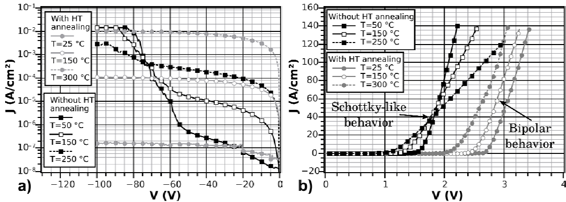
Fig. II.3.21 Effet du recuit à 1700 °C sur le comportement électrique J-V en température des diodes p + /n dont la couche p + a été réalisée par croissance VLS: sous polarisation en inverse (a) et en direct (b).
