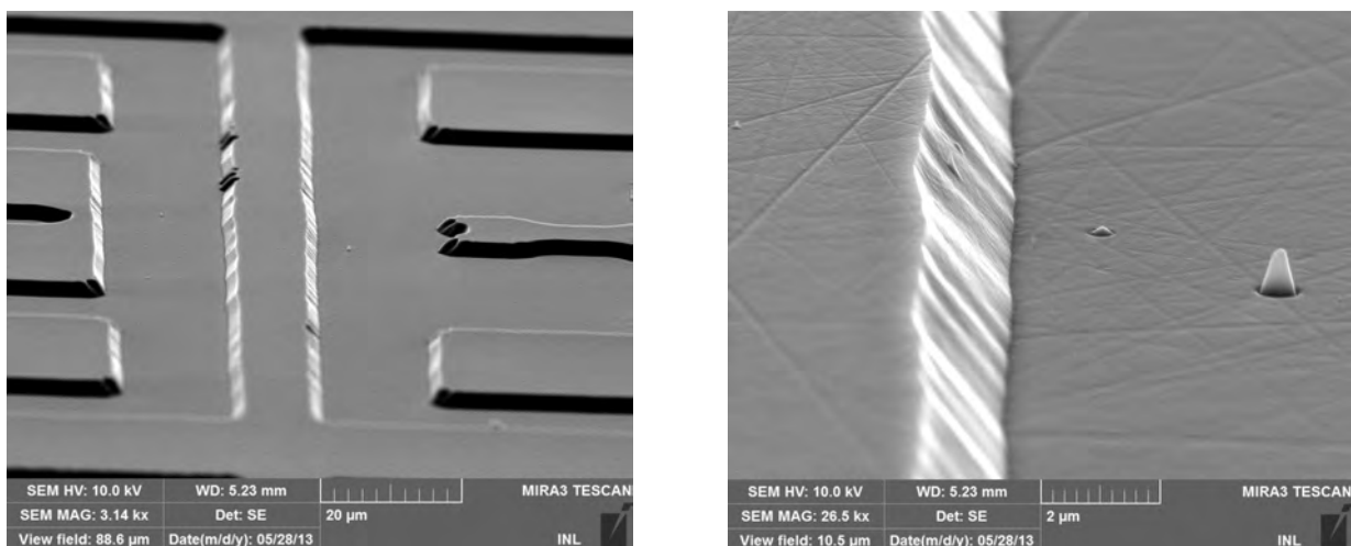
Fig. II.3.44. Images MEB de surfaces SiC gravées avec une chimie SF 6 en utilisant le bâti Oxford NGP80 et des masques en résines MAP1240 et LOR 30B
