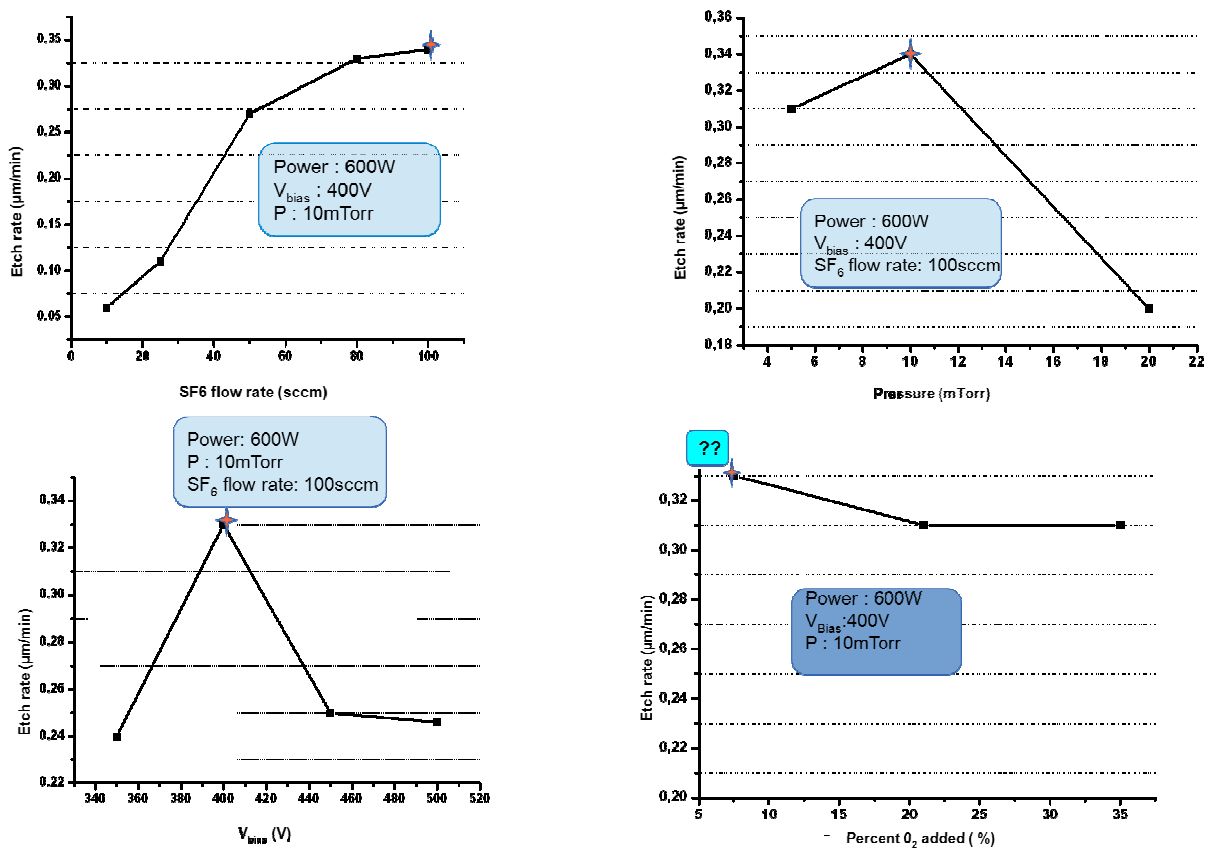
Fig II.3.49 : Optimisation des paramètres de gravure ICP plasma \text{SF}_6 (débit, pression, bias, pourcentage \text{O}_2 ) pour la réalisation de tranchées profondes et étroites de la protection DT^2 en SiC.
