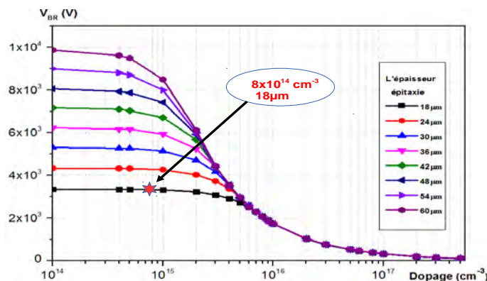
Fig. II.3.46 Tenue en tension 1D estimée en utilisant les coefficients d'ionisation de Konstantinov [Kons'98] pour des couches N de drift SiC en fonction de leurs dopages et épaisseurs.
