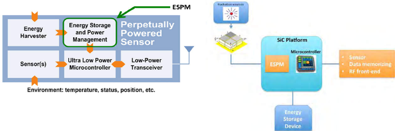
Fig. II.5.6 Intégration du capteur SiC multipixels dans un système autoalimenté
