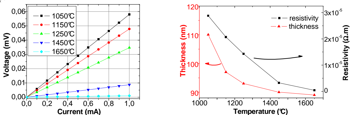
Fig. II.5.14. I-V par mesures 4-pointes sur les couches PPF recuites à différentes températures (à gauche). Résistivité extraite et épaisseur des couches vs température (à droite).
