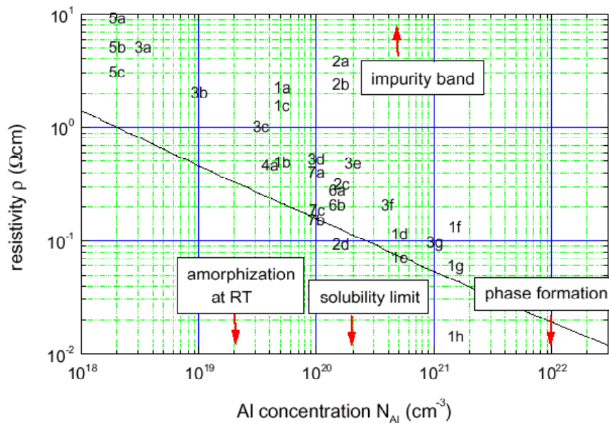
Fig. II.3.3 : Les résistivités obtenues par implantation ionique d'aluminium pour des fortes concentrations avec des limites physiques: amorphisation, solubilité et dégénérescence [Heer'01].
