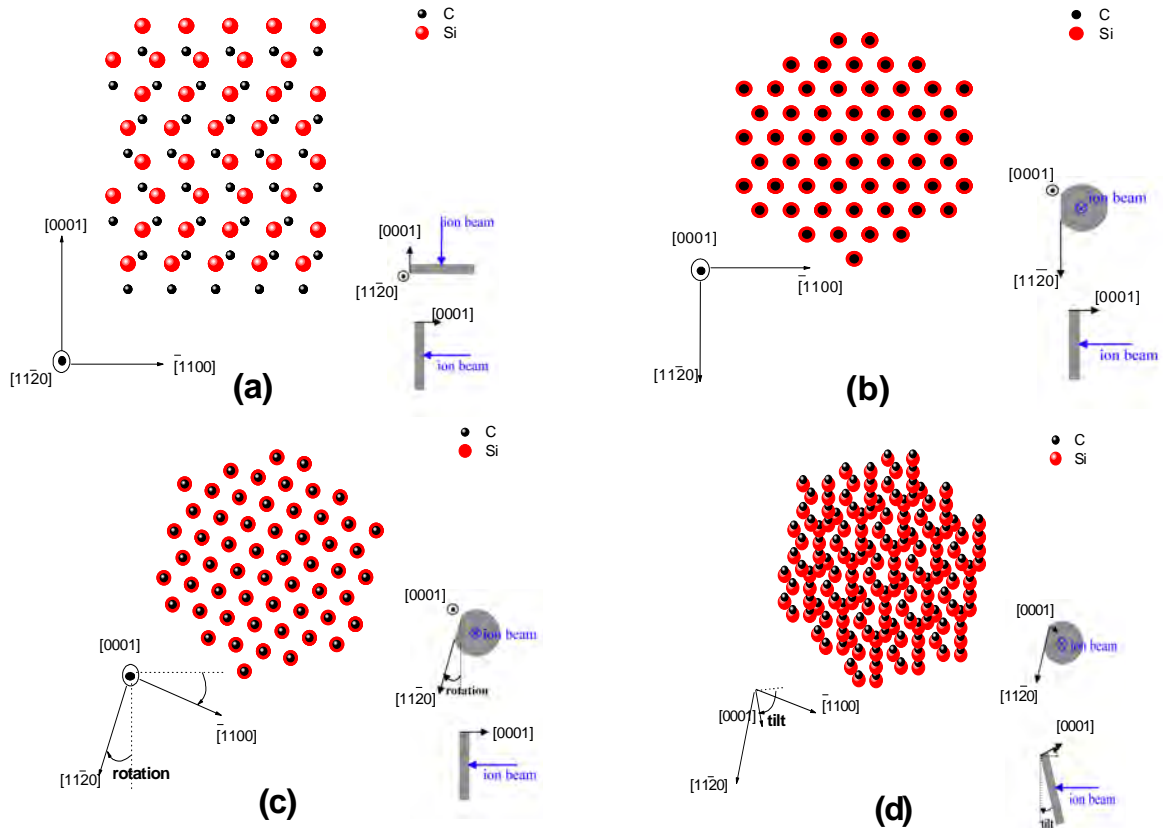
Fig. II.3.13. Structure cristalline SiC-4H en coupe (a) et vue par le faisceau ionique sans désorientation (b), après une rotation suivant l'axe [0001] (c) et après un tilt supplémentaire (d).
