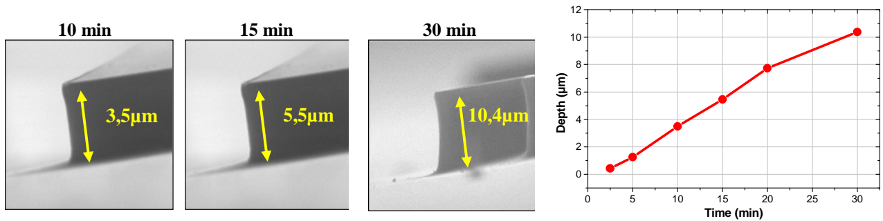
Fig. II.3.35 Trois clichés MEB montrant des flancs SiC obtenus après 10, 15 et 30 min de gravure RIE SF 6 /O 2 (25sccm/6,7sccm) à 250W et 60mTorr. A droite: courbe expérimentale profondeur vs temps gravure [RI25].
