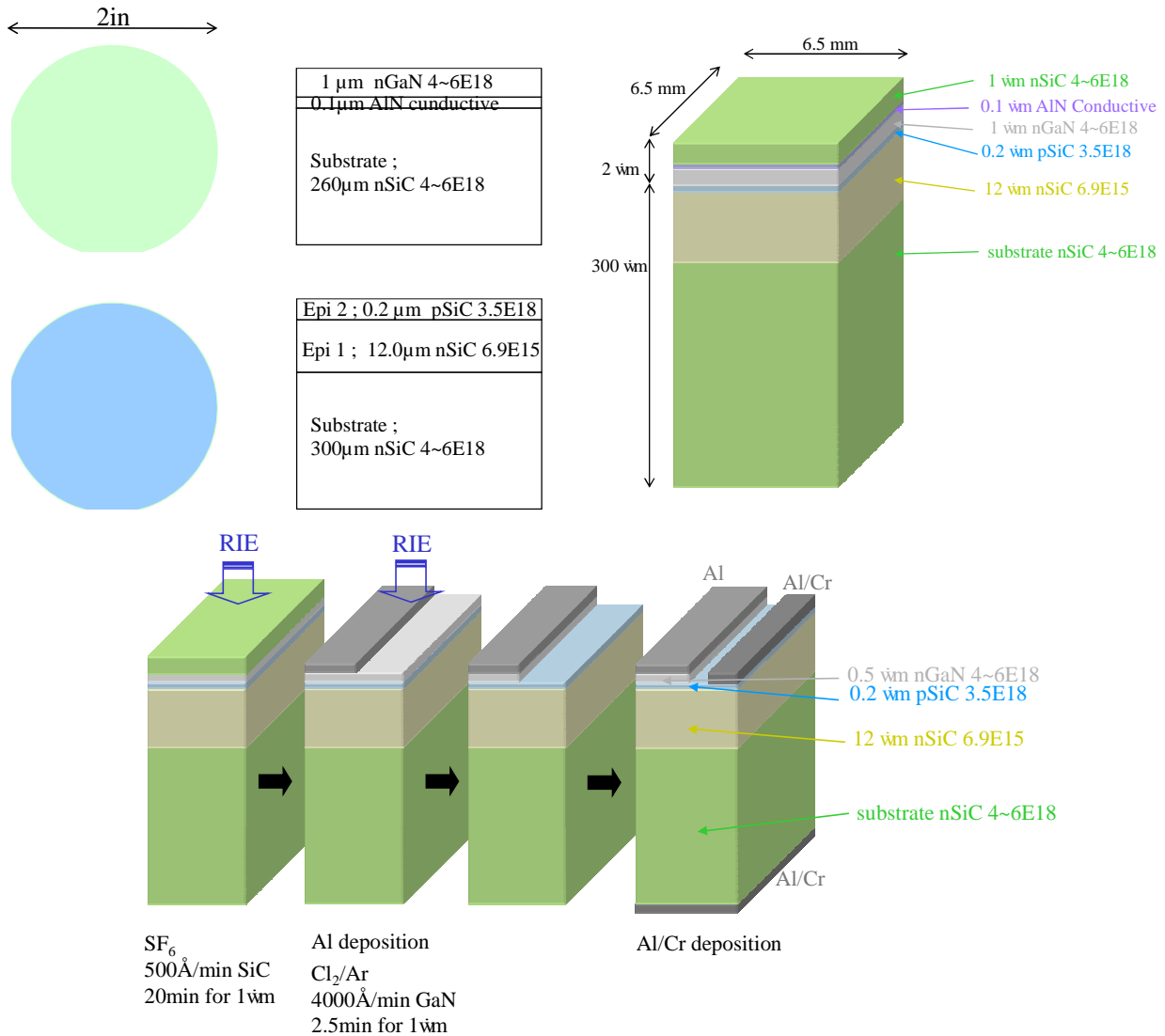
Fig. III.6.5. HBT GaN/SiC fabriqué par Lee et al. en 2002 montrant la structure obtenue par collage (bonding) moléculaire et polissage des substrats SiC utilisés (en haut) et la structure finale ou des gravures RIE ont été utilisées pour l'ouverture des prises de contact (en bas).
