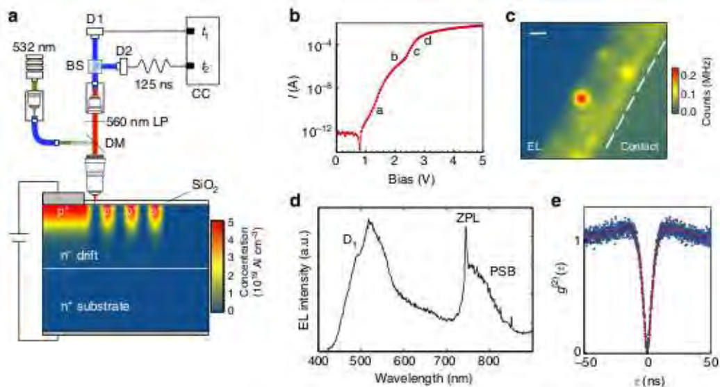
Fig.III.5.2 : Sources de photon unique dans une diode PiN 4H-SiC: (a) banc expérimental confocale (b) caractéristique I-V de la diode avec différents régimes (c) cartographie par électroluminescence (EL) de la périphérie sous polarisation directe 10V. Le spot brillant central est un défaut SPS (d) spectre EL du défaut SPS avec un ZPL (zero phonon line) à 745 nm [Lhor'15].
