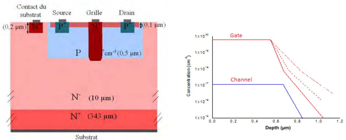
Fig. II.3.14 Structure (à gauche) des composants JFET latéraux que nous avons fabriqués dans le cadre du projet ANR JFET-SB, présentant un canal latéral bloqué à cause du manque de contrôle de la queue du profil d'implantation de la grille, représentée schématiquement (à droite)
