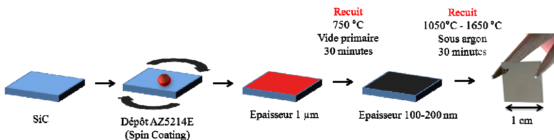
Fig. II.5.13 Synthèse et recuit de couches PPF par pyrolyse de résines AZ5214E déposées sur SiC.
