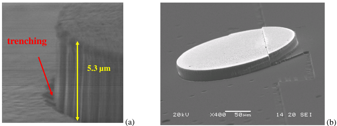
Fig. II.3.39 : Impact de l'état de surface initial sur la formation du trenching: gravure RIE d'une surface implantée (a), gravure ICP d'une surface qui a déjà subi partiellement une autre étape de gravure.
