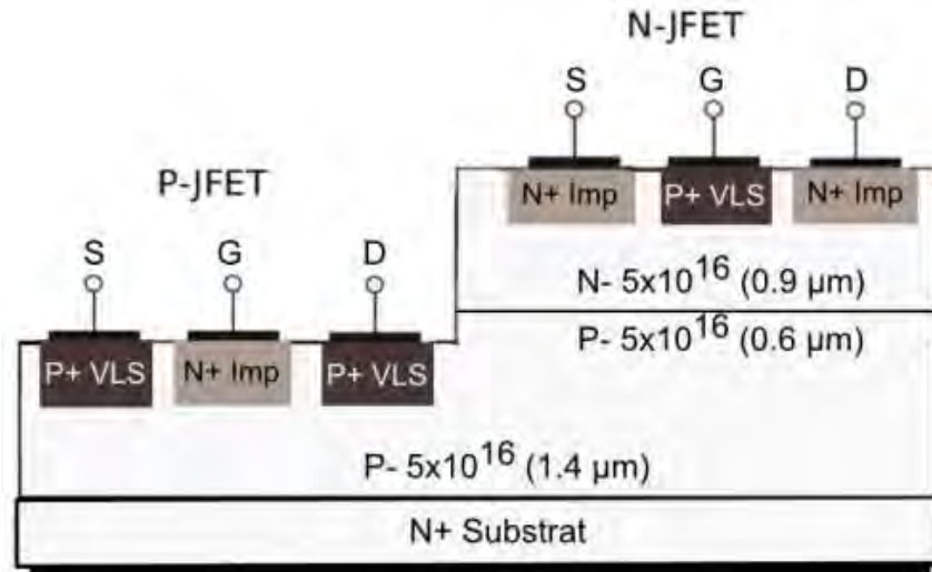
Fig. II.4.17: Présentation schématique des JFETs latéraux N et P intégrés monolithiquement avec des caissons P + réalisés par croissance VLS.
