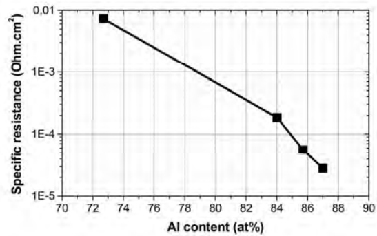
Figure II.3.63 Résistances spécifiques des contacts Ni/Al en fonction du taux d'aluminium présent dans la métallisation [RI24].
