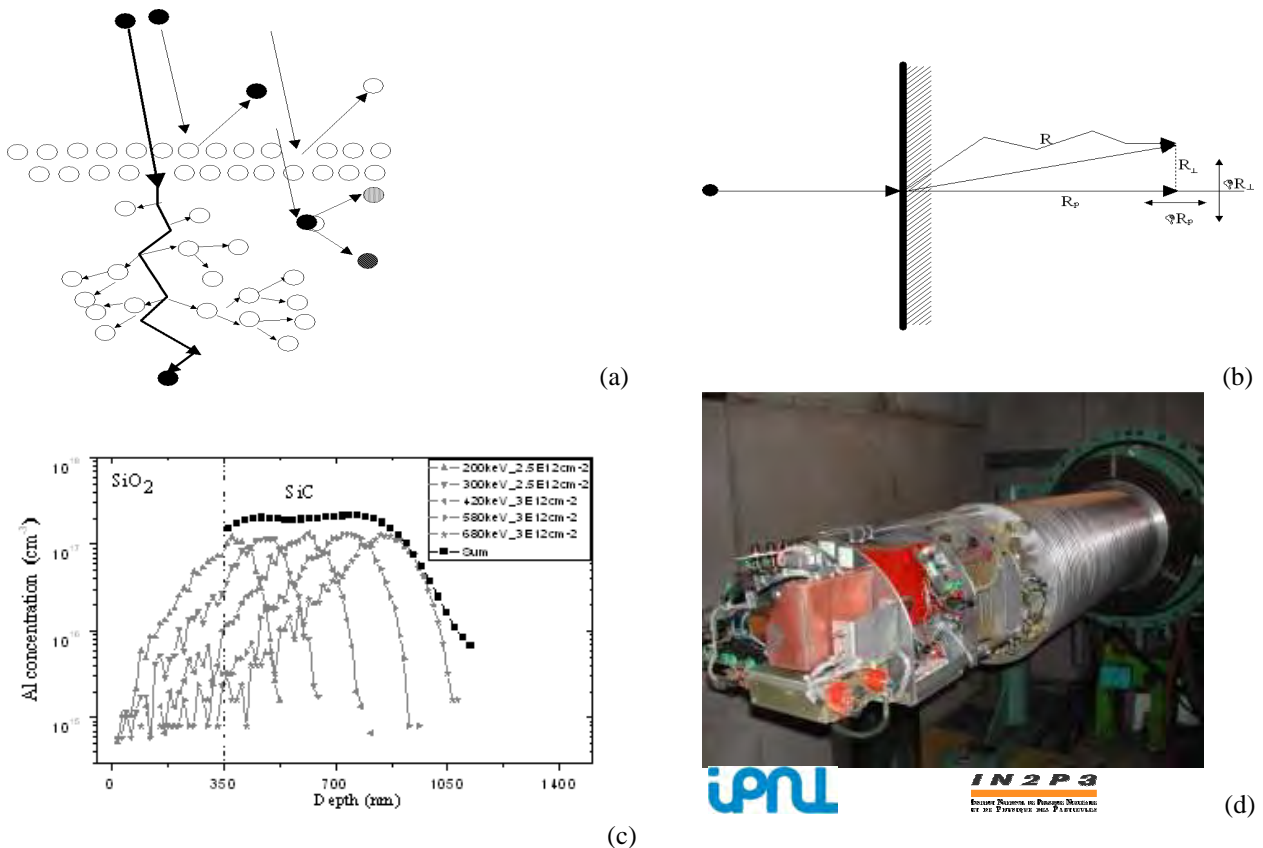
Fig. II.3.2 : Schéma d'une implantation ionique dans un semiconducteur cristallin (a); parcours projeté d'un ion (b); profil d'implantation aluminium typique dans le SiC pour une JTE (c); image de l'accélérateur 100-400 kV de l'implanteur "classique" de l'IPNL, fabriqué maison et utilisé dans nos travaux (d).
