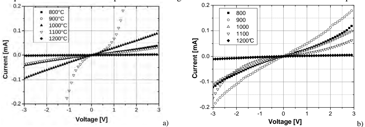
Figure II.3.64 La formation des contacts ohmiques a lieu à 1000°C pour l'alliage où l'épaisseur de la couche initiale de titane est de 25 nm (a) et à 900°C dans le cas où celle-ci était de 48 nm (b). Dans les deux cas, l'épaisseur de la couche de nickel était de 100 nm.
