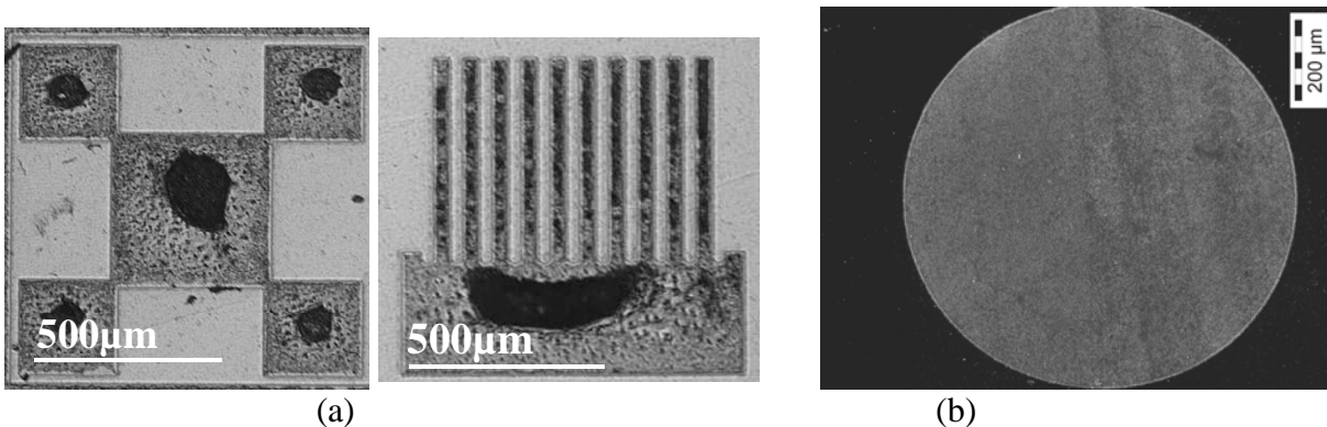
Fig. II.3.17 Images de couches SiC type p réalisées par croissance VLS localisée en configuration sans caissons gravés (a) et avec caissons gravés (b) à la surface du SiC.
