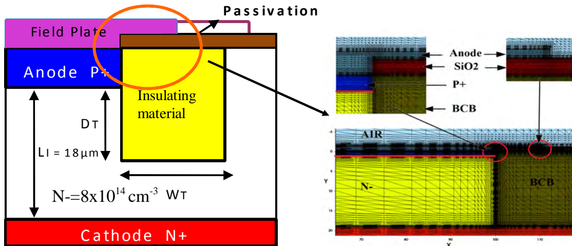
Fig II.3.47 : Design et présentation schématique de la structure de nos composants 3 kV obtenue par simulation TCAD Sentaurus
