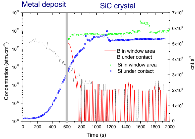
Fig. II.5.2 Analyses SIMS du contact métallique au-dessus des zones P + créées par immersion plasma
