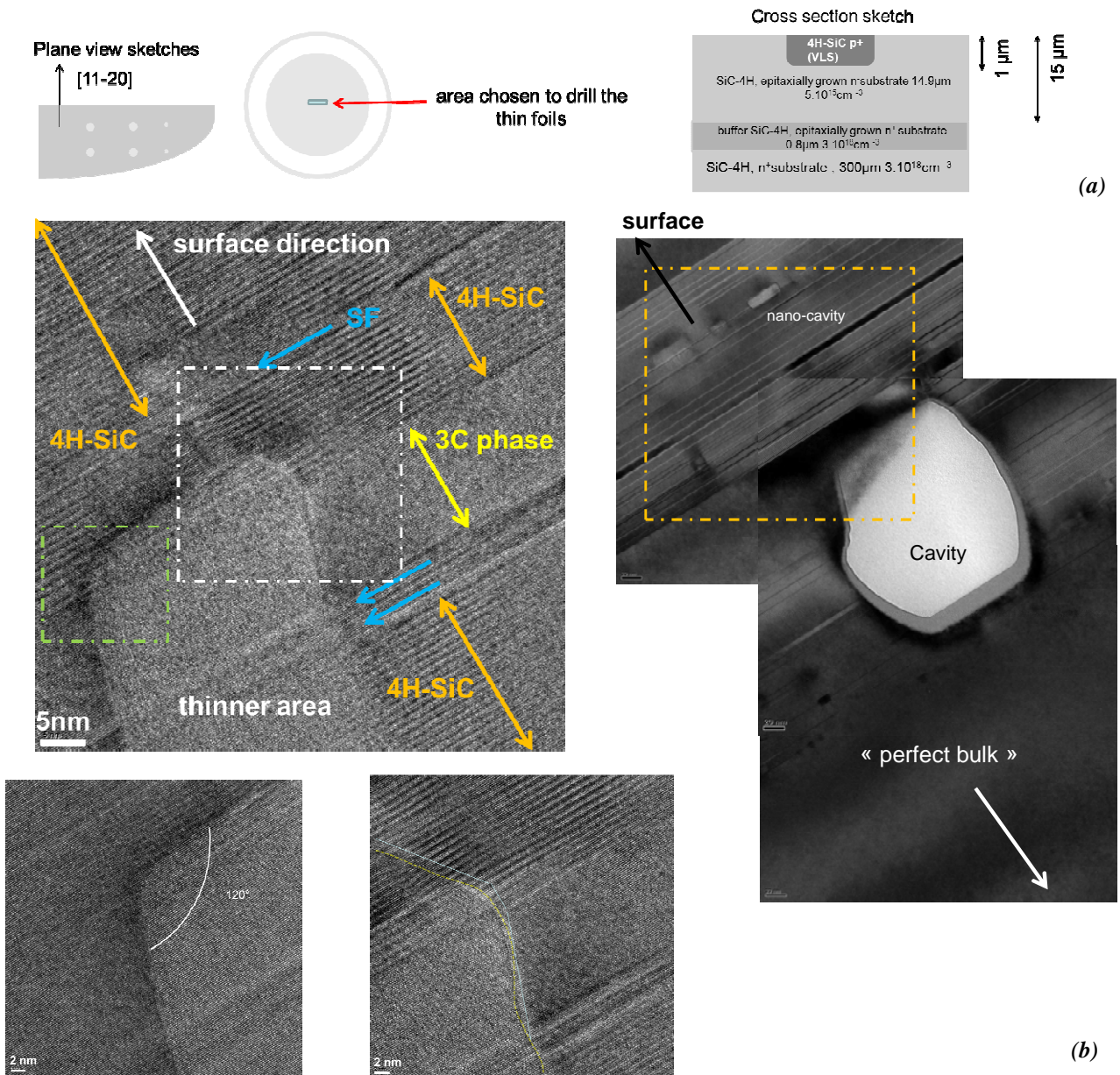
Fig. II.3.20 Présentation schématique des échantillons (a) et résultats des analyses HR-TEM (b) mettant en évidence les défauts structuraux dans la couche VLS et à l'interface avec la surface initiale de SiC
