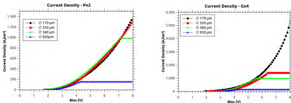
Fig. II.2.28. Caractéristiques J-V en direct de deux lots de diodes verticales VLS
