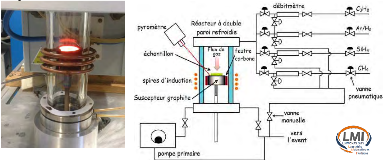
Fig. II.3.16 Réacteur vertical à parois froides du LMI dédié aux croissances VLS du SiC
