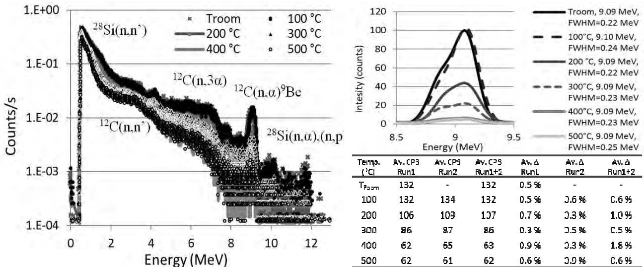
Fig.II.5.11 Mesures réalisées jusqu'à 500 °C avec un générateur de neutrons rapides de l'Université Technique de Dresde à 14 MeV sous un flux de 2,4 à 3,1 \times 10^7 n/cm 2 s.
