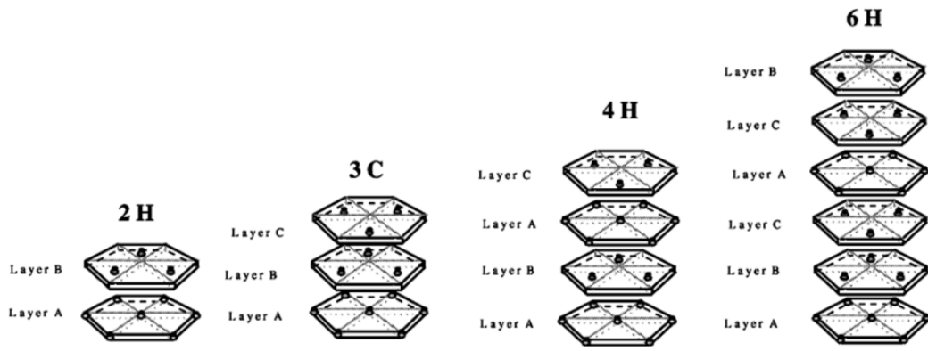
Fig. II.2.2: Présentation des structures cristallographiques compactes de quatre polytypes de SiC en notation de Ramsdell
