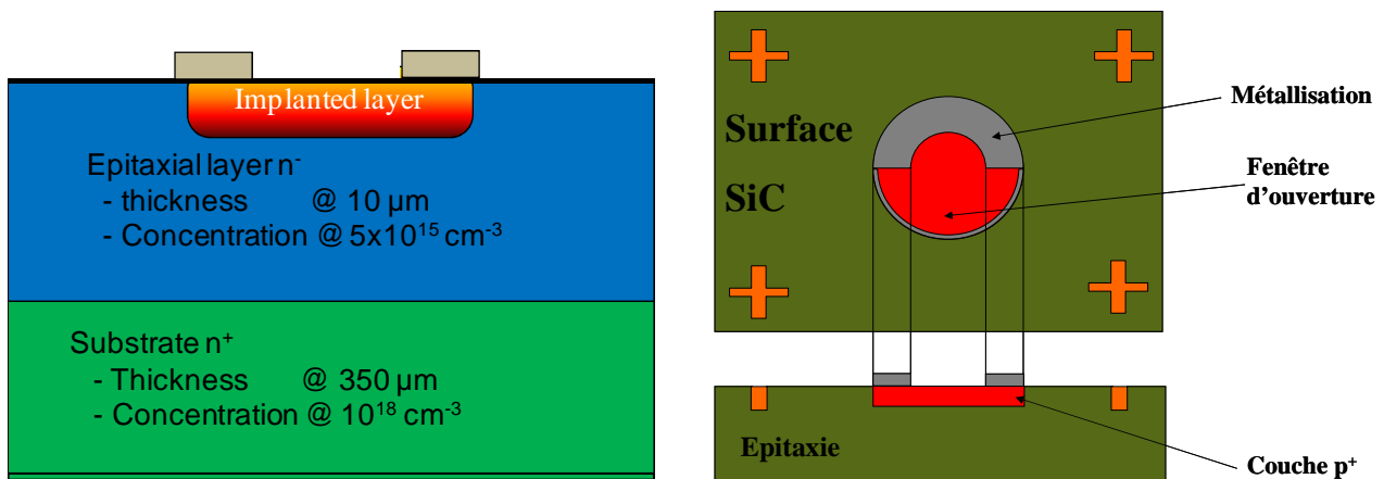
Fig. II.5.1 Structures des photodétecteurs UV en SiC, vue en coupe à gauche et vue mixte de dessus et en coupe à droite
