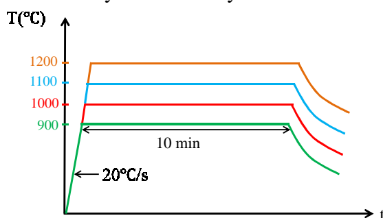
Figure II.3.74. Profil typique du recuit des alliages Ti_xAl_{100-x} sur SiC pour la formation du Ti_3SiC_2 .
