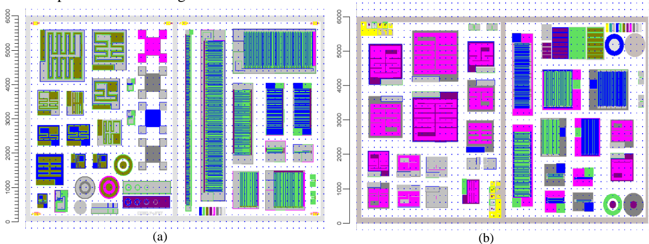
Figure II.4.8 Superposition des niveaux de masques pour des structures planaires (a) et gravées (b). L'échelle de l'ordonnée est graduée en µm.
