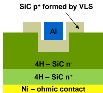
Fig. II.3.27. Structure d'une diode verticale VLS
