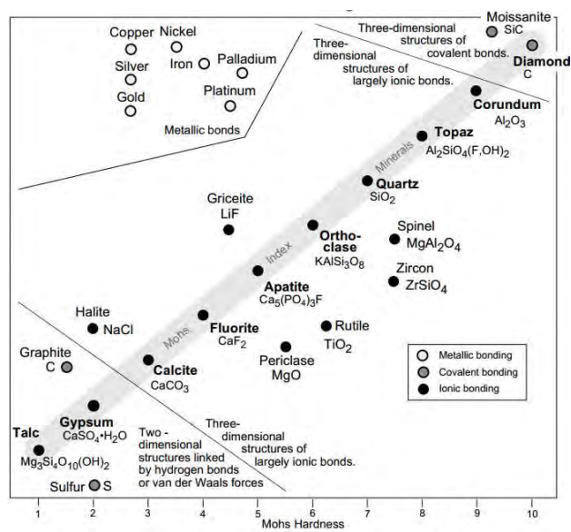
Fig. II.2.3: La dureté de différents matériaux dont SiC et diamant, sur l'échelle de Mohs.
