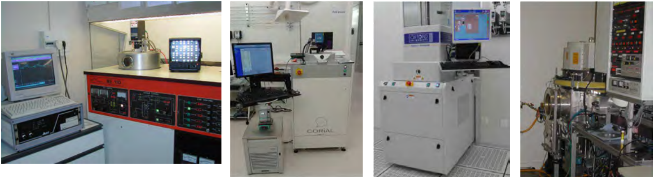
Fig. II.3.31 Bâtis de gravure plasma utilisés sur la plateforme Nanolyon, de gauche à droite: RIE Nextral NEE110, Corial 200S, Oxford NGP80 et l'ICP ETREM.
