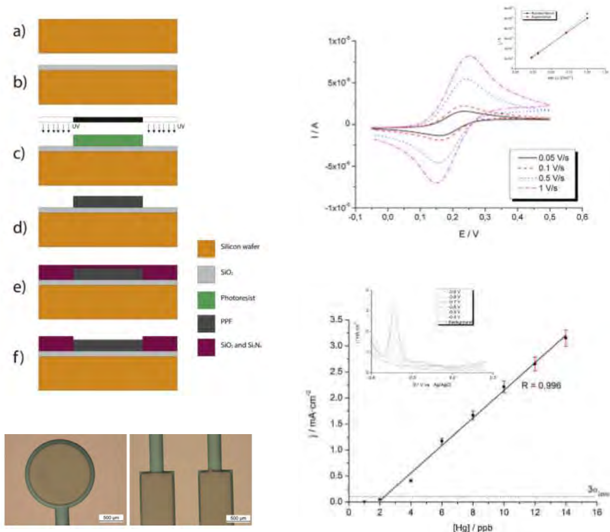
Fig. III.4.1. Détecteur de mercure (Hg) en silicium avec des électrodes en PPF [Sanc'13]. A gauche la réalisation technologique et à droite les caractéristiques électrochimiques y compris courbe d'étalonnage pour la détection.
