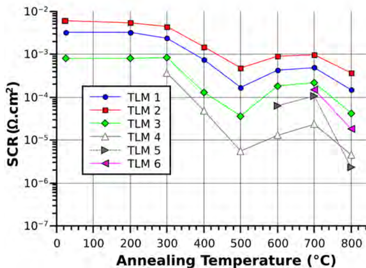
Figure II.3.78. Résistances spécifiques de contact sur les couches VLS en fonction de la température de recuit.
