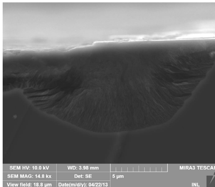
Fig. II.3.55. Cliché MEB d'une coupe verticale sur un substrat SiC après gravure électrochimique.
