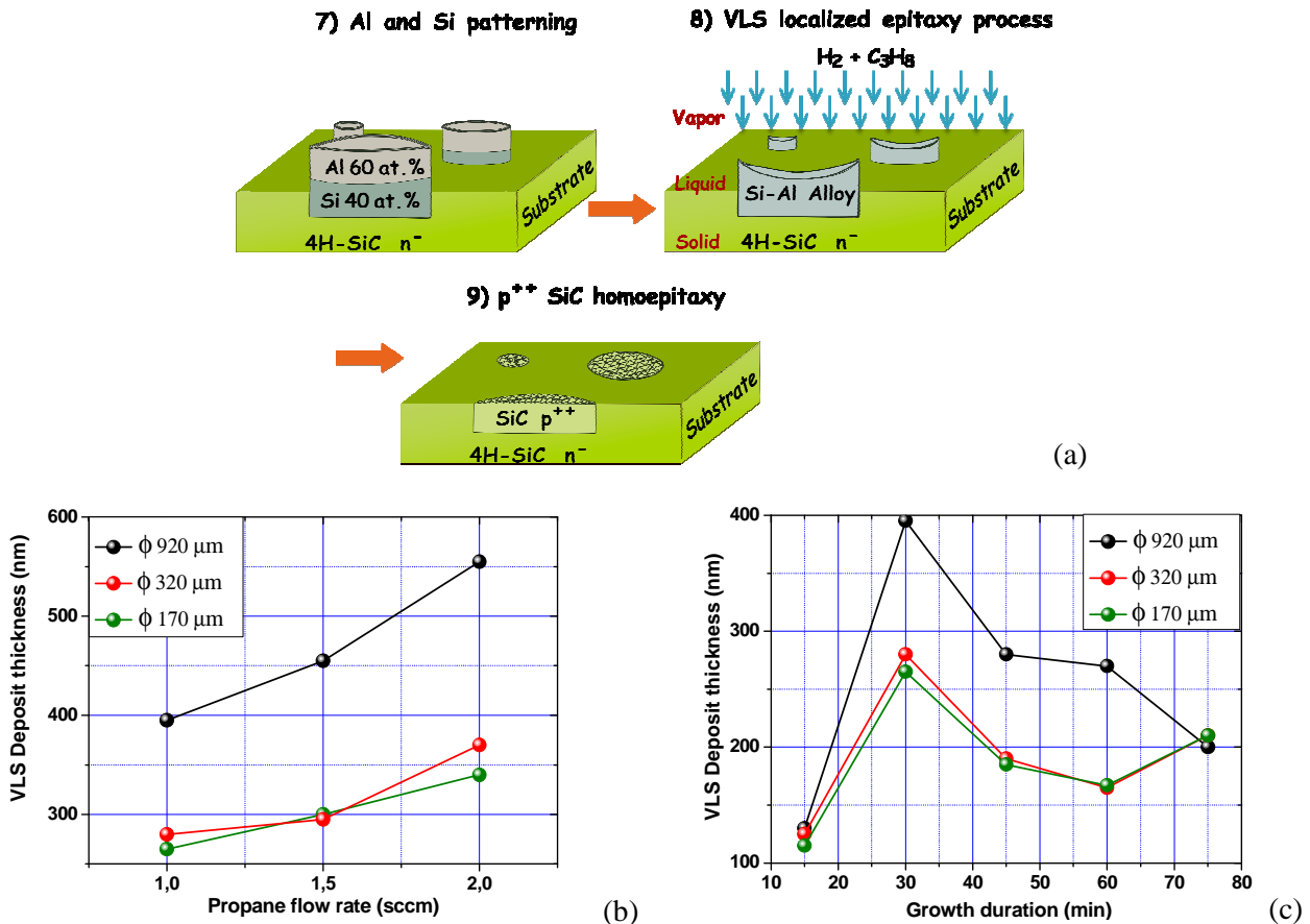
Fig. II.3.26. Représentation schématique de la configuration VLS retenue, H 2 - C 3 H 8 (a) et variation de l'épaisseur des couches obtenues avec le flux de propane (b) et avec durée de croissance (c). Dans les deux cas, la croissance a eu lieu à 1100 °C [RI84].
