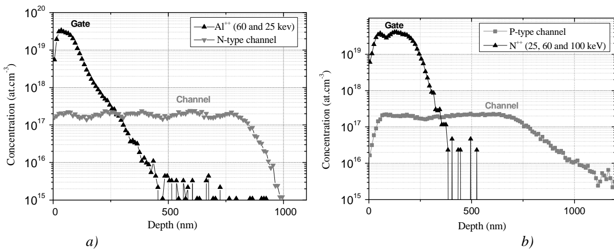
Fig.II.4.15. Paramètres des implantations ioniques et profils de dopages des grilles et des canaux optimisés par simulation MC I 2 SiC pour les N-JFET (a) et les P-JFET (b) de l'étage de puissance.
