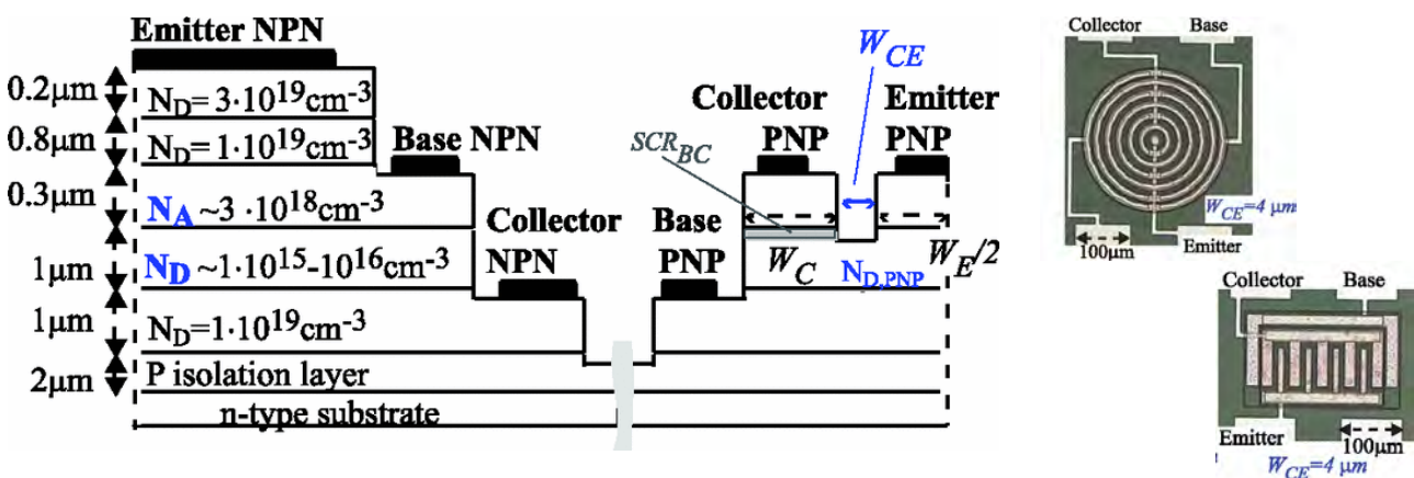
Fig. II.4.2 Technologie bipolaire pour l'intégration d'un transistor vertical NPN et un latéral PNP pour la réalisation de circuits intégrés analogiques [Lann'14].
