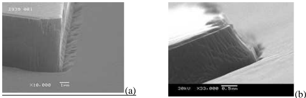
Fig. II.3.37. Micrographies MEB sur des échantillons SiC-4H gravés avec un plasma 25 sccm SF_6 et 6,7 sccm O_2 à (a) 100 W, 30 mTorr, 30 min et (b) 100 W, 60 mTorr, 10 min.
