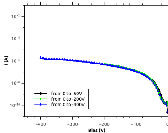
Fig. II.3.29 Caractéristiques I-V en inverse typique et tenue en tension des diodes verticales VLS
