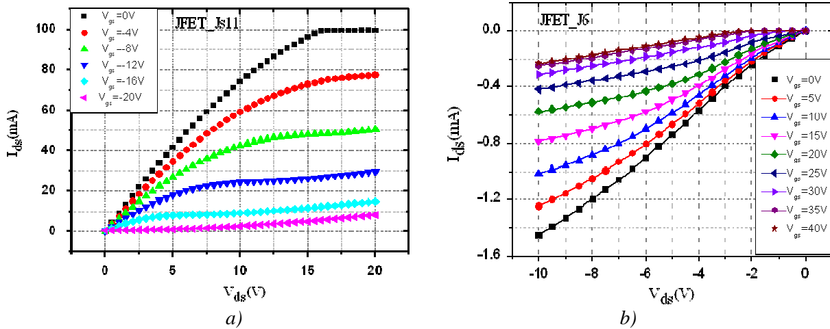
Fig. II.4.16. Des caractéristiques électriques typiques I_{ds} - V_{ds} versus V_{gs} pour les N-JFET (a) de l'étage de puissance et les P-JFET (b) de l'étage de commande.
