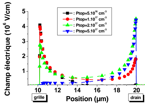
Fig. II.4.7 Distribution du champ électrique dans le JFET latéral
