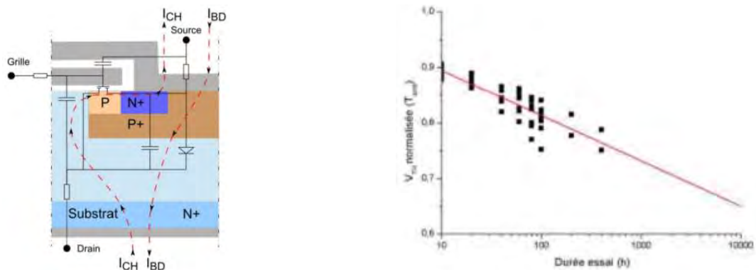
Fig. III.2.2 A gauche: schéma d'un MOSFET vertical SiC, canal et diode bipolaire interne. A droite : dérive du V_{TH} [Salv'16].
