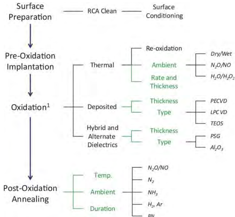
Fig. III.3.1 Présentation schématique des étapes technologiques envisagées pour réaliser l'oxydation du SiC et améliorer la qualité de l'interface SiC/diélectrique [Sidd'16].
