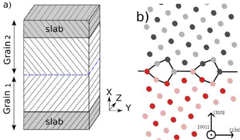
Figure B.11: a) Schéma de la cellule de simulation. b) Configuration du joint de grain de \Sigma 13(320) projeté dans le plan (x, y) : les atomes noir (gris) et rouge (rose) appartiennent aux différents grains.
