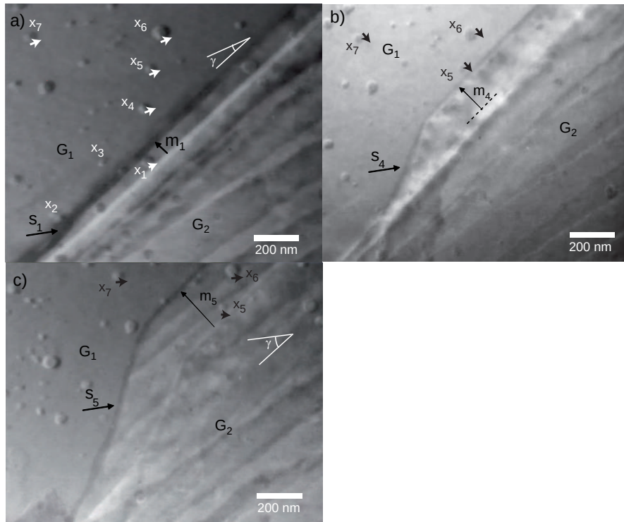
Figure B.6: Différence d'image obtenue par soustraction de contraste des images prises avant et après le mouvement de la marche s_1 (a), s_4 (b) et s_5 (c). En superposant les marqueurs dans G_2 , un décalage dans la position des marqueurs dans G_2 est observé indiquant la déformation produite due à la migration. Le facteur de couplage possède à la fois une composante parallèle et perpendiculaire au joint de grains.
