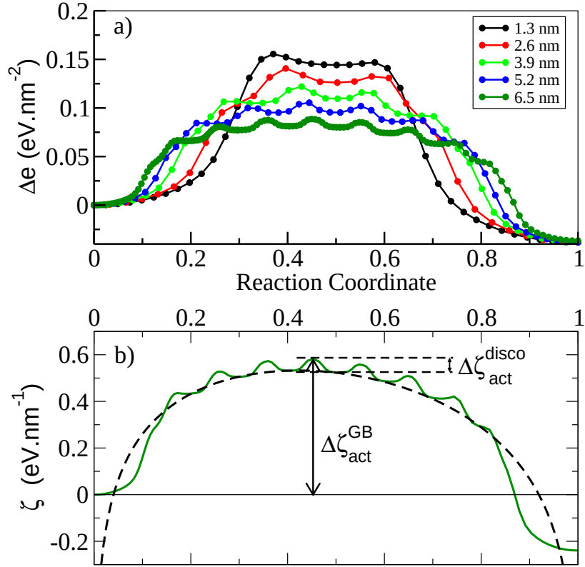
Figure B.14: a) Chemin d'énergie minimum -MEP- (ligne pleine) par unité de surface en fonction de RC pour d = 0.066 nm pour 5 cellules de tailles différentes selon y , allant de 1 à 5 périodes de joint de grain (la taille selon z est de 1.4 nm). b) Chemin d'énergie minimum -MEP- par unité de longueur de disconnection en fonction de RC pour d = 0.066 nm (cellule de 6.5 nm et 1.4 nm de long selon y et z ) et variation de l'énergie (ligne en pointillés) selon la théorie de l'élasticité et Eq. (4.27).
