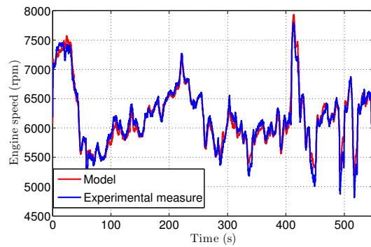
(d) Engine model identification
