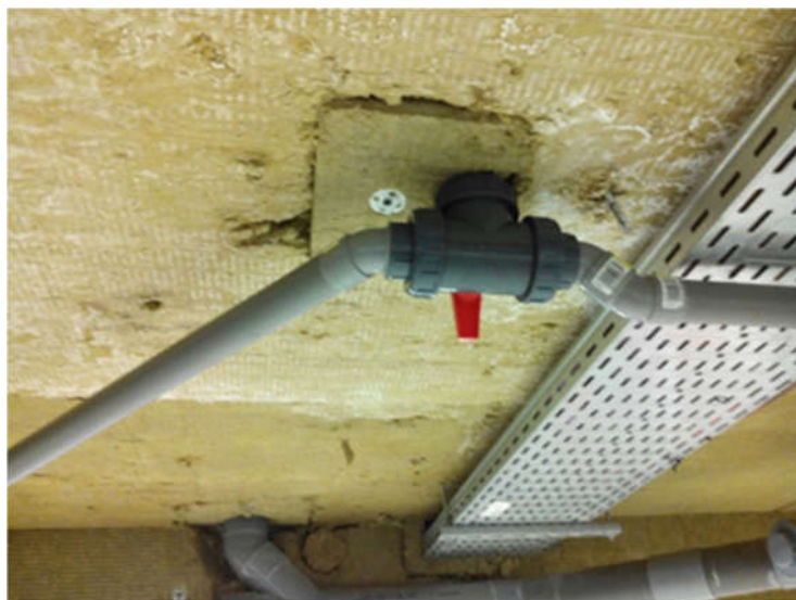
Figure 4.24 : « Vanne de transition socio-écologique » du projet Azuris.
