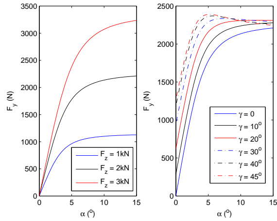
FIGURE 2.17 – Influence de la charge et de l’angle de carrossage sur la force latérale
