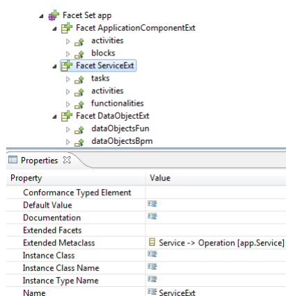
FIGURE 4.26 – Capture d'écran de la Facet ServiceExt
