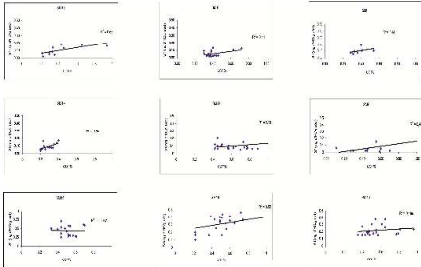
Figure 47b : Valeurs des paramètres liés (Y) en fonction de COT.
