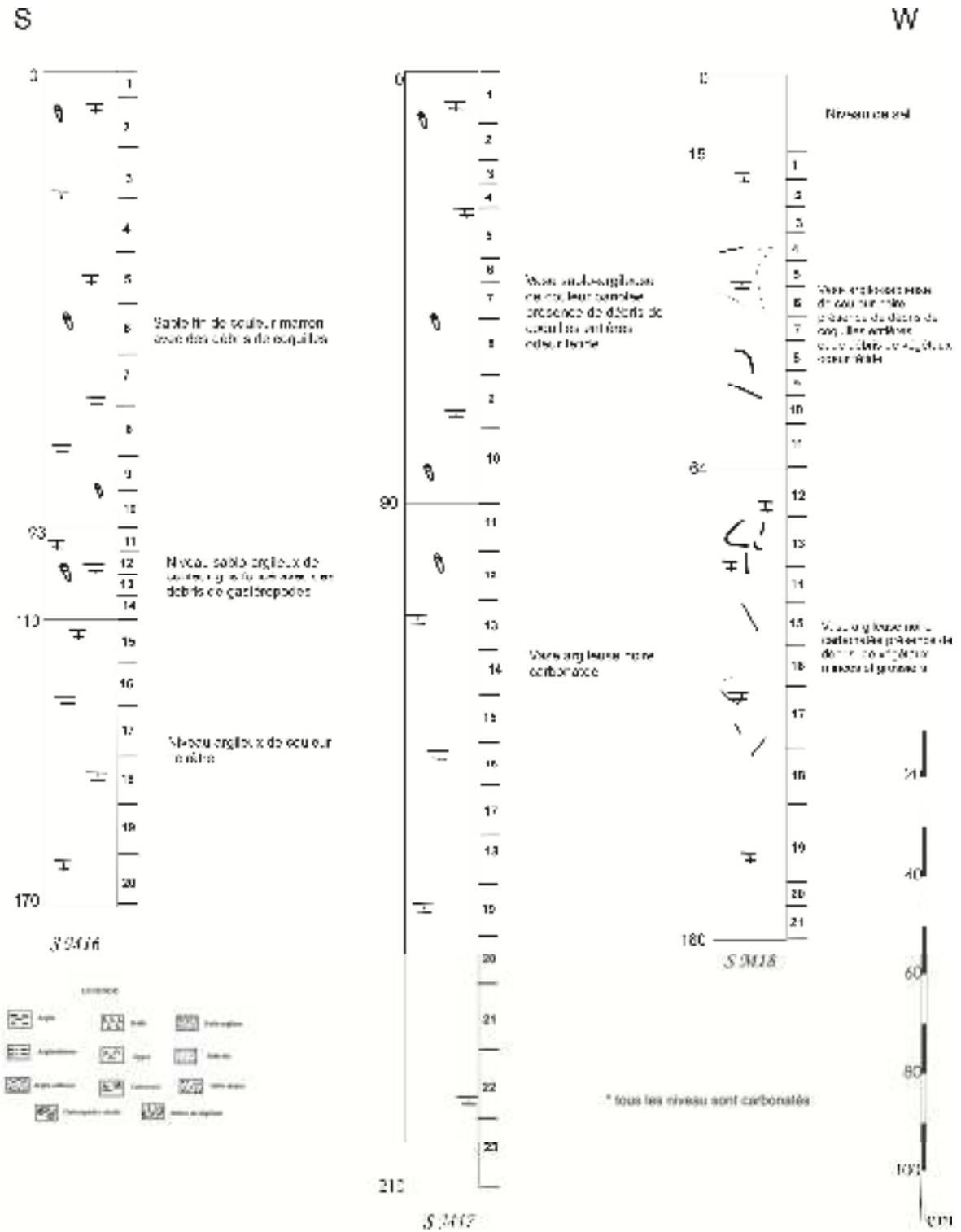
Figure 17 : Corrélation stratigraphique des profils réalisés au Vu-Chest de la sablière de Moknine.
