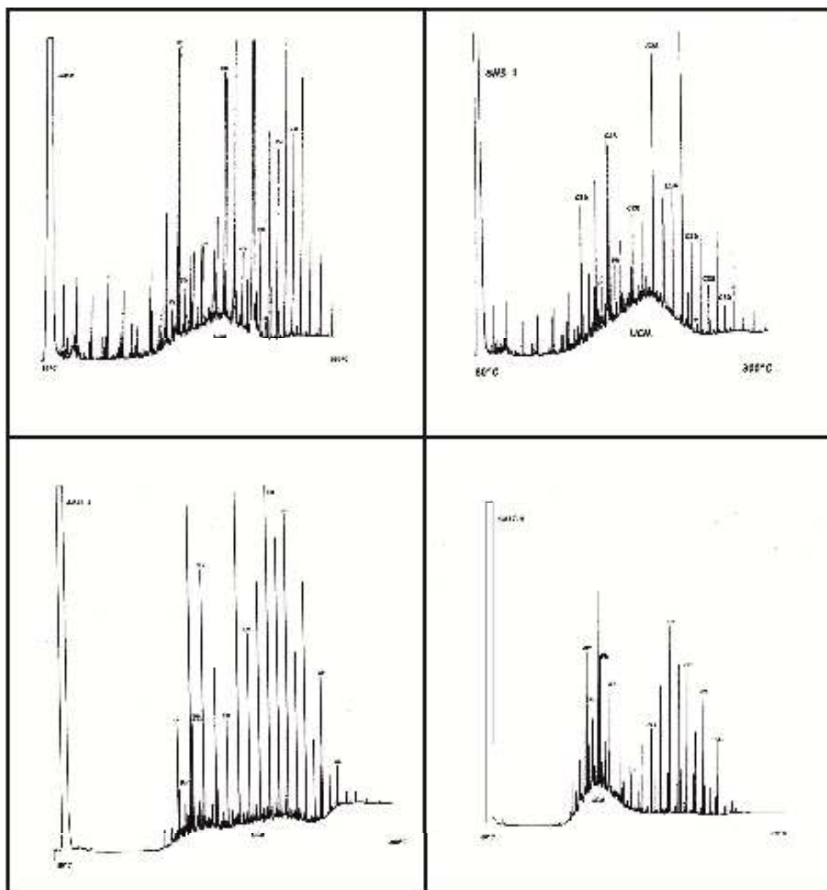
Figure 3.3b : chromatogrammes des hydrocarbures saturés et insaturés non aromatiques des sédiments (en sub-surface) prélevés dans la zone médiane de la sébkha de Moknine. (UCM : composé non résolu, Pr: pristane, Ph: phytane, *: squalène)
