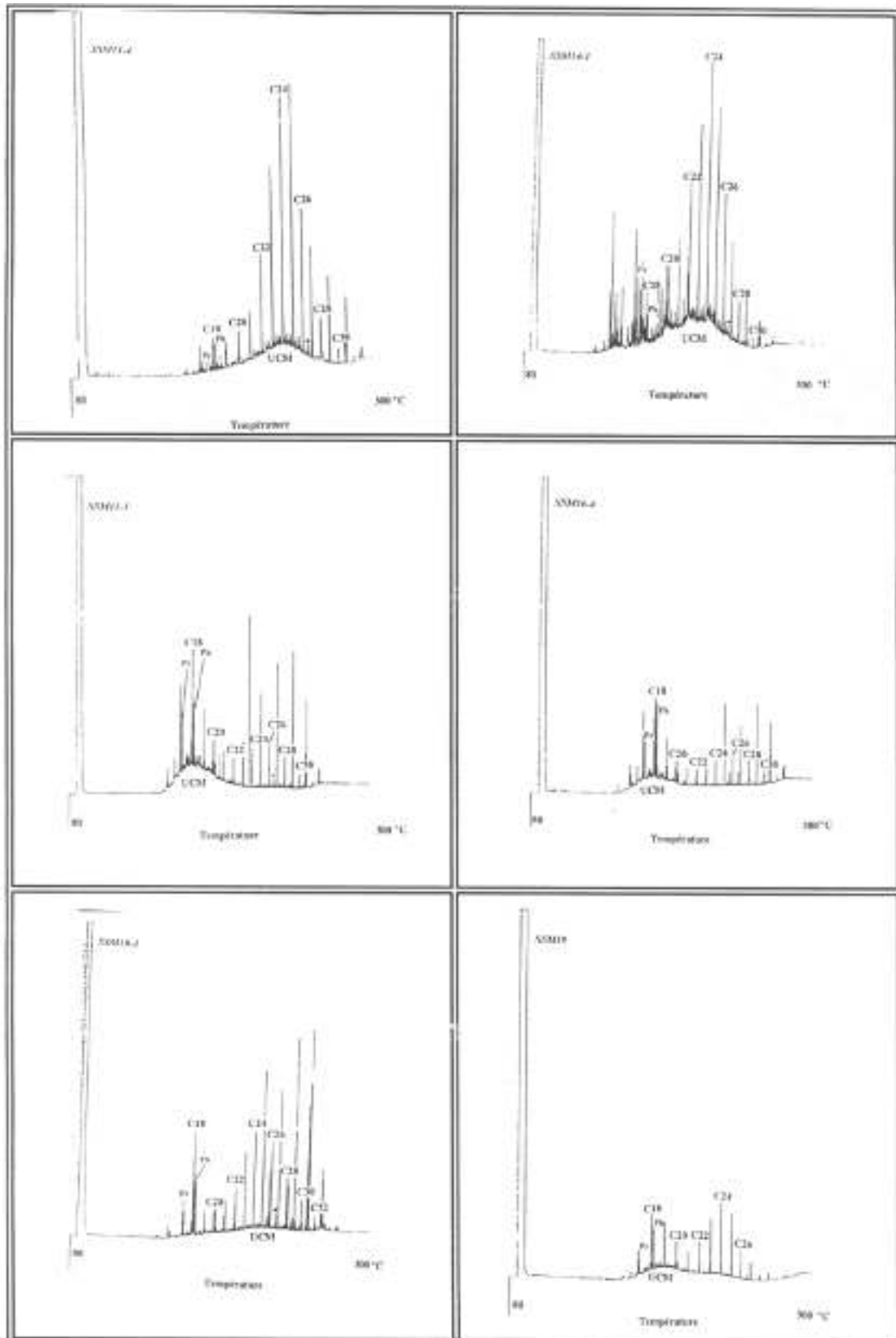
Figure 45 : Chromatogrammes des hydrocarbures saturés et insaturés non aromatiques des sédiments de surface de la partie émergée. (UCM : composés non résolus, Pr : pristane, Ph : phytane, * squalane)
