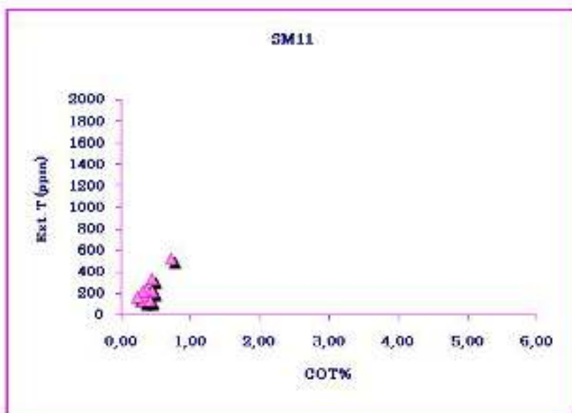
Figure 5.1g : Variation de l'extrait chloroformique total (Ext. T) en fonction du COT Radiuse 344
