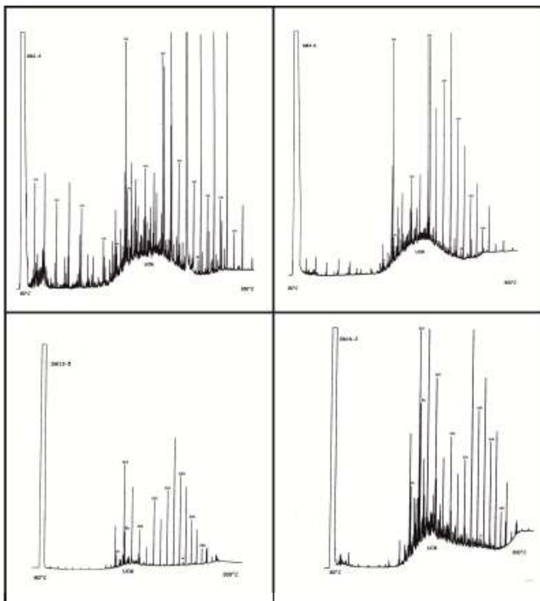
Figure 55a : chromatogrammes des hydrocarbures saturés et insaturés non aromatiques des sédiments (à sécheresse) prélevés à la périphérie de la sébja de Moknine. (100°C : composés non tétra, 120°C : pristane, 140°C : phytane, 170°C : squalène)
