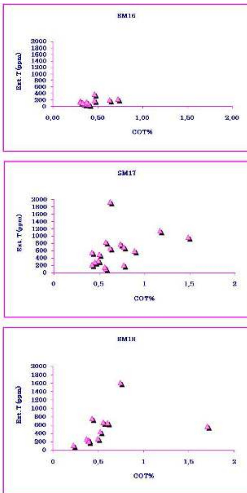
Figure 51e : Variation de l'extrait chloroformique total (Ext. T) en fonction du COT. Radiale 54V
