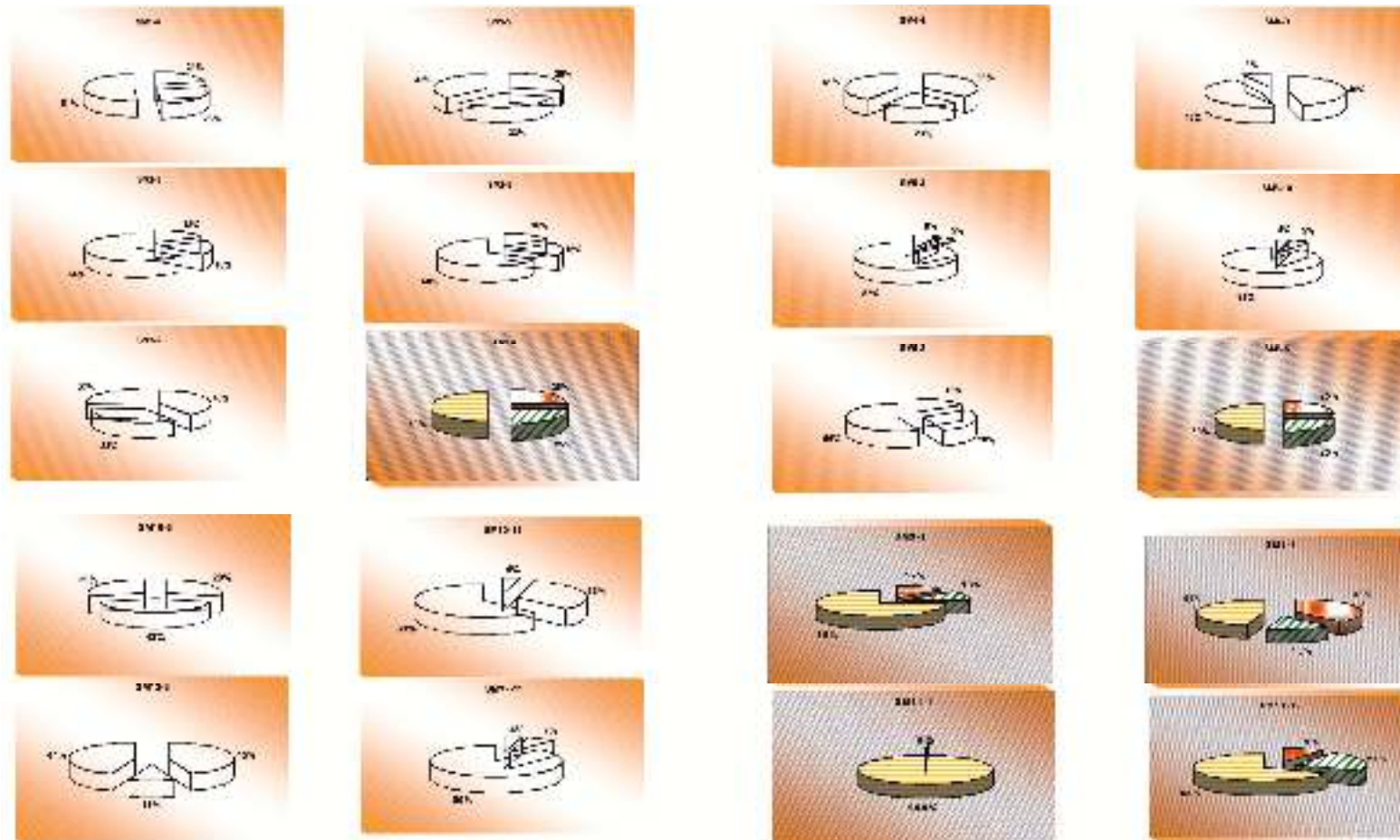
Figure 5.2a : Pourcentages des fractions de l'extrait chloroformique total
