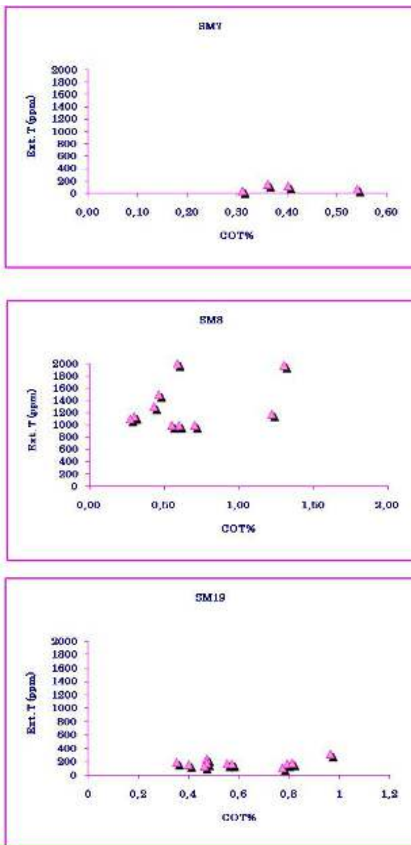
Figure 51f: Variation de l'extrait chloroformique total (Ext. T) en fonction du COT. SM7-SM8-SM19
