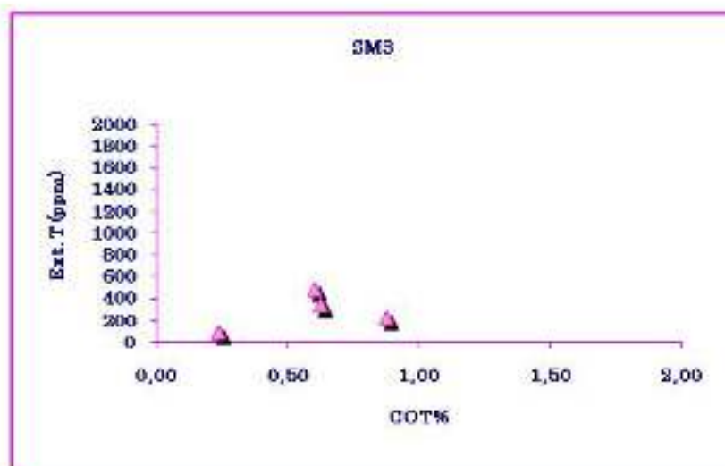
Figure 5 1a : Variation de l'extrait chloroformique total (Ext. T) en fonction du COT. Réduite NE
