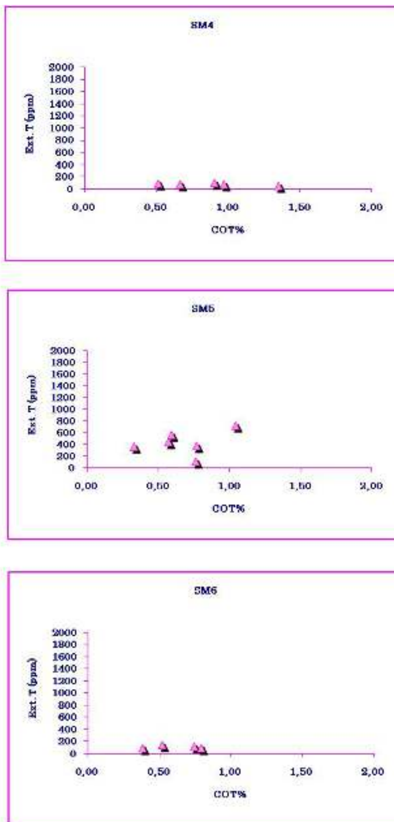
Figure 5.1b : Variation de l'extrait chloroformique total (Ext. T) en fonction du COT Résultats SE
