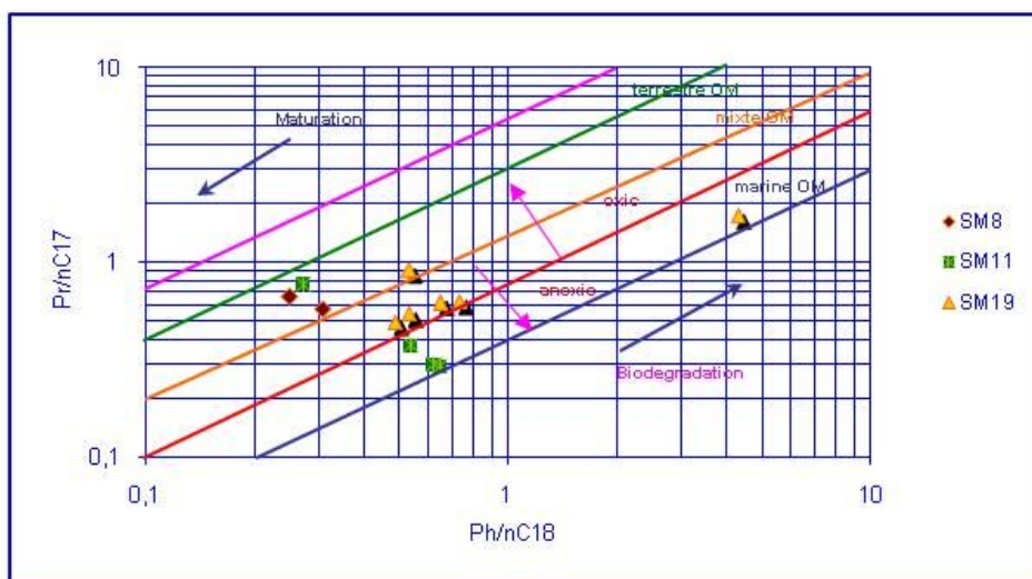
Figure 5 46 : diagramme de wapels : Type de matière organique, environnement de dépôt et degrés de maturité.
