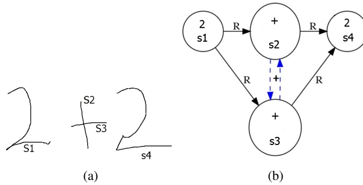
Figure 8.2 – (a) « 2 + 2 » écrit en quatre traits ; (b) le graphe SLG de « 2 + 2 ». Les quatre traits sont repérés s1, s2, s3 et s4, respectant l'ordre chronologique. (ver.) et (hor.) ont été ajoutés pour distinguer le trait horizontal et vertical du '+'. 'R' représente la relation Droite.
