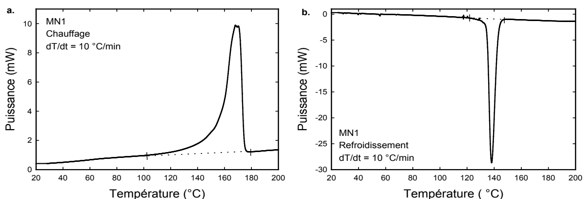
Figure II.9: Thermogrammes a. de fusion et b. de cristallisation du iPP obtenus par DSC.
