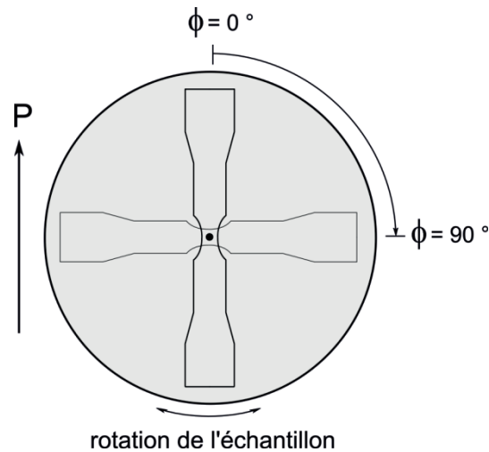
Figure IV.4: Protocole des mesures de diffusion Raman sur le iPP déformé en traction en fonction de l'angle \phi entre la direction de traction z et celle de la polarisation P .
