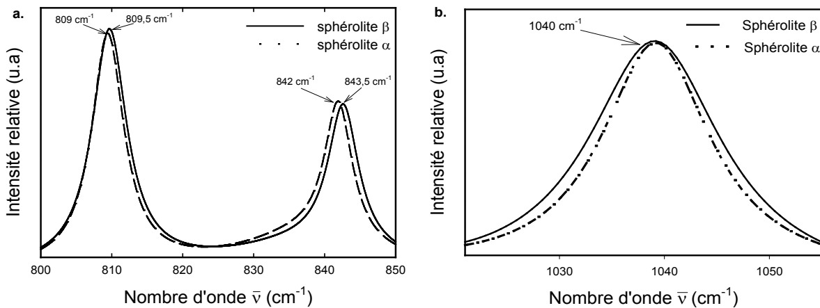
Figure III.13: Spectres de diffusion Raman enregistrés sur un sphérolite \alpha et \beta du iPP a. de 800 à 850 \text{cm}^{-1} et b. de 1020 à 1060 \text{cm}^{-1} .
