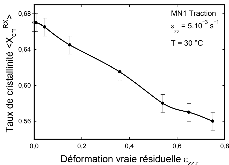
Figure III.7: Evolution du taux de cristallinité moyen en masse \langle X_{cm}^{RX} \rangle , déterminé par diffraction des rayons X, en fonction de la déformation vraie résiduelle \varepsilon_{zz,r} du iPP.
