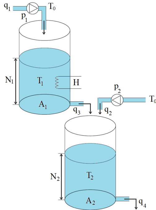
FIGURE 2.1 – Système hydraulique
