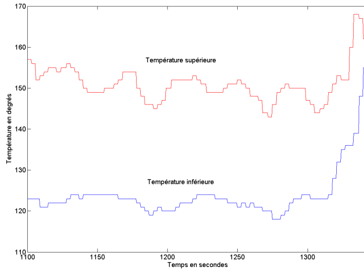
FIGURE 5.13 – Températures des thermocouples de la colonne 4
