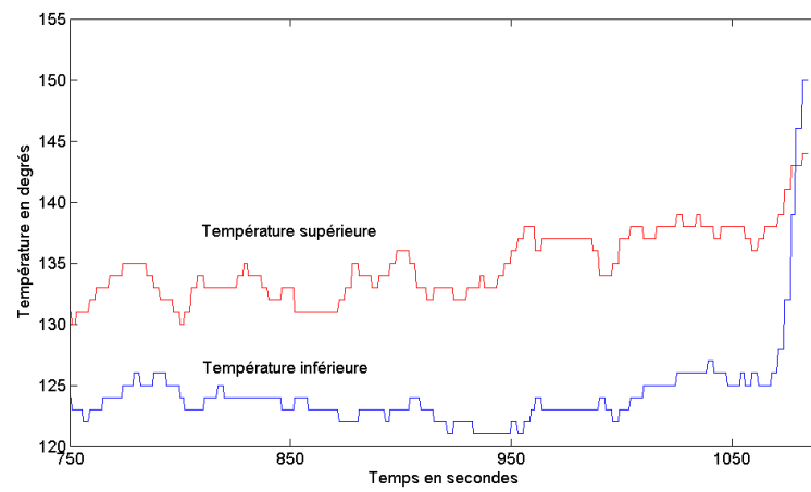
FIGURE 5.18 – Températures des thermocouples de la colonne 5
