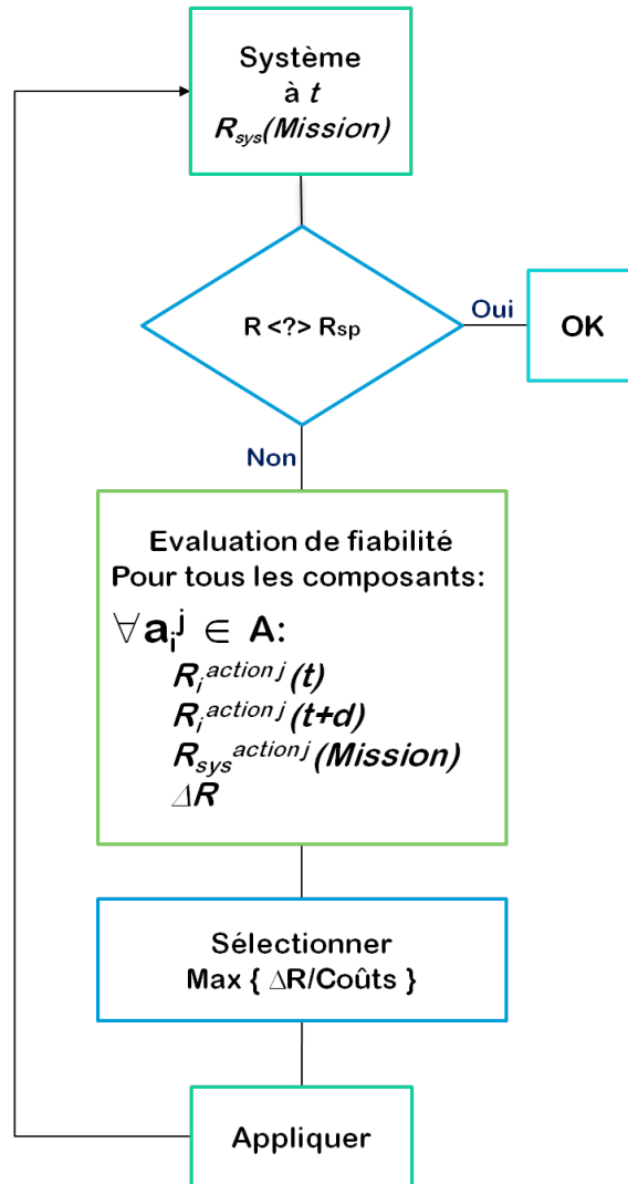
FIGURE 3.15 – Démarche d'optimisation
