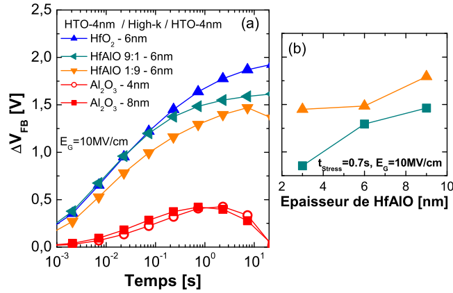
FIG. 3.26: a) Caractéristiques de programmation \Delta V_{FB} - Temps_{Stress} d'empilements HfO-4nm / High-κ / HfO-4nm pour différents types de High-κ . b) Décalage de la tension de bande plate pour différentes concentrations de HfAlO pour V_G/EOT = 10 MV/cm et t_{Stress} = 0,7 s.
