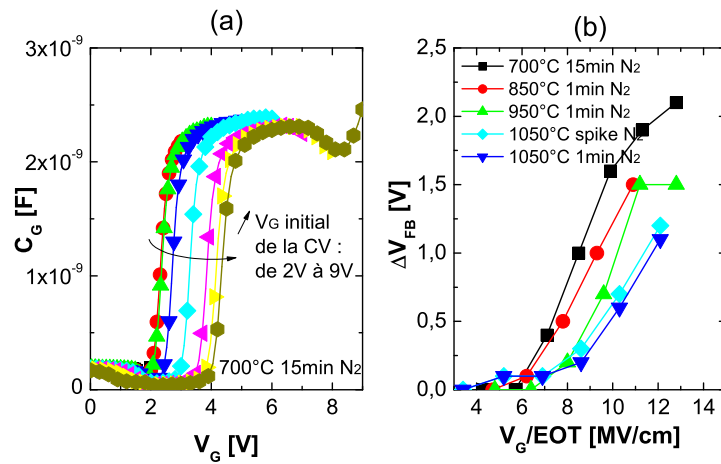
FIG. 3.47: (a) Caractéristiques C_G - V_G permettant d'effectuer des mesures de piégeage de l'alumine recuite à 700 ° C 15 min sous N_2 . Caractéristiques de piégeage de couches d'alumine \sim 15nm ayant subi différents recuits post-déposition (b) sous atmosphère N_2 .
