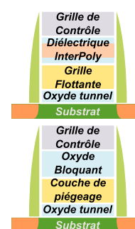
FIG. 3.10: Schémas de cellules mémoires à grille flottante et à couche de piégeage.
