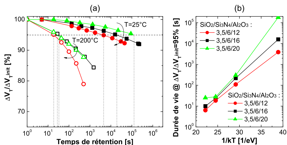
FIG. 4.35: (a) Caractéristiques de rétention normalisées \Delta V_T / \Delta V_{T_{init}} pour différentes épaisseurs d'alumine (12nm, 16nm et 20nm) à 25^\circ\text{C} et à 200^\circ\text{C} . (b) Tracés Arrhenius pour différentes épaisseurs d'alumine. V_{T_{prog}} \sim 6\text{V} et \Delta V_{T_{prog}} \sim 5\text{V} .
