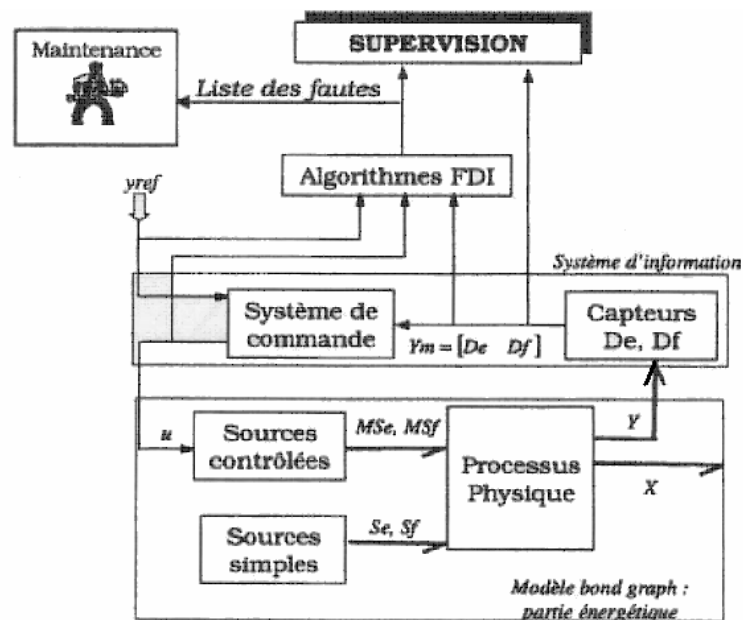
Figure 1.4. Représentation bond graph d'un système de surveillance.
