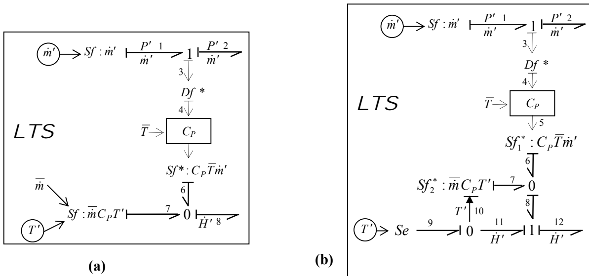
Figure 5.9. Modèles BG Linéarisés d'une Source Thermo fluide LTS.
