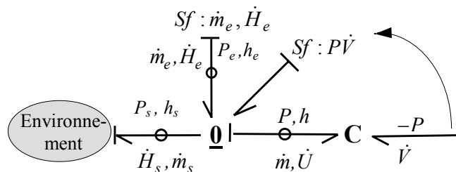
Figure 2.24. Modèle bond graph d'un accumulateur avec \dot{U} comme variable de flux
