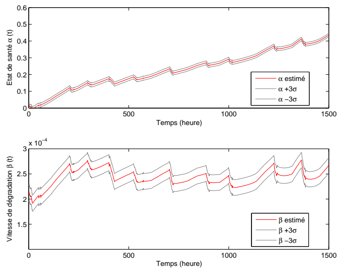
FIGURE 4.25 – Estimation de \alpha_k et de \beta_k à charge constante avec un interval de confiance de 99%
