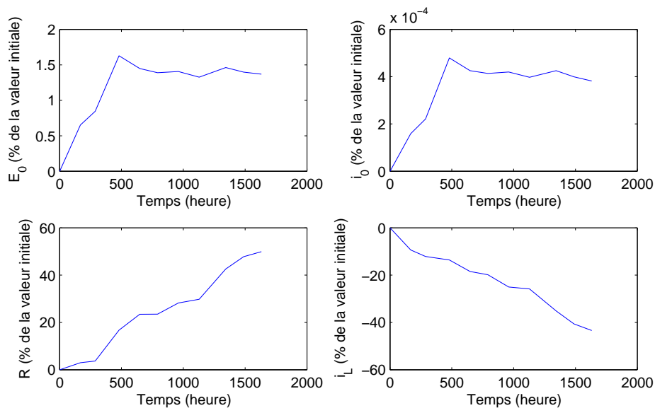
FIGURE 4.11 – Déviation des paramètres extraits des courbes de polarisation à charge constante
