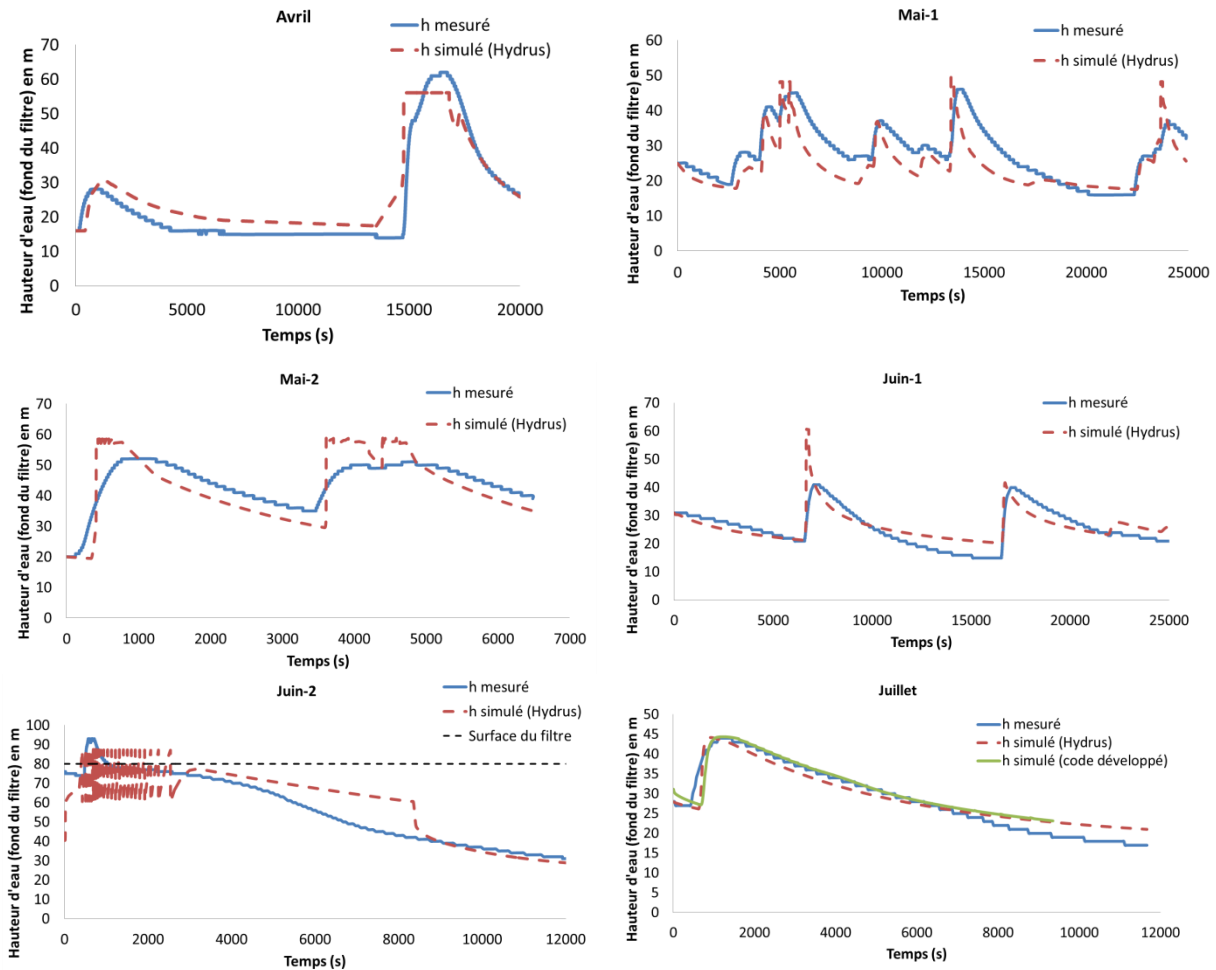
FIGURE 113:COMPARAISON ENTRE LES HAUTEURS D’EAU MESUREES IN SITU ET LES HAUTEURS SIMULEES POUR 5 EVENEMENTS PLUVIEUX AUX MOIS D’AVRIL, MAI, JUIN ET JUILLET 2013
