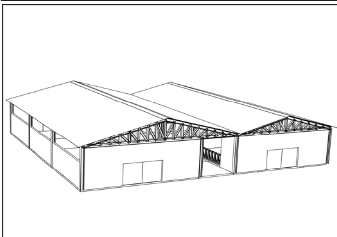
Photo n°10 : vue en perspective étable longitudinale pour 60 génisses (30 : moins de 1 an ; 30 : plus de 1 an).
