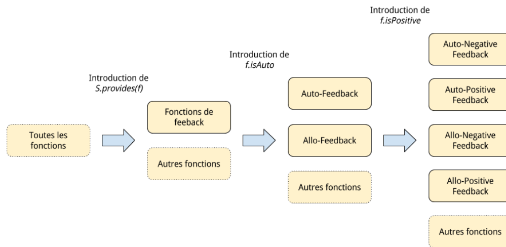
Fig. 4.2.: Processus d'extraction des traits primitifs pour les fonctions de feedback .
