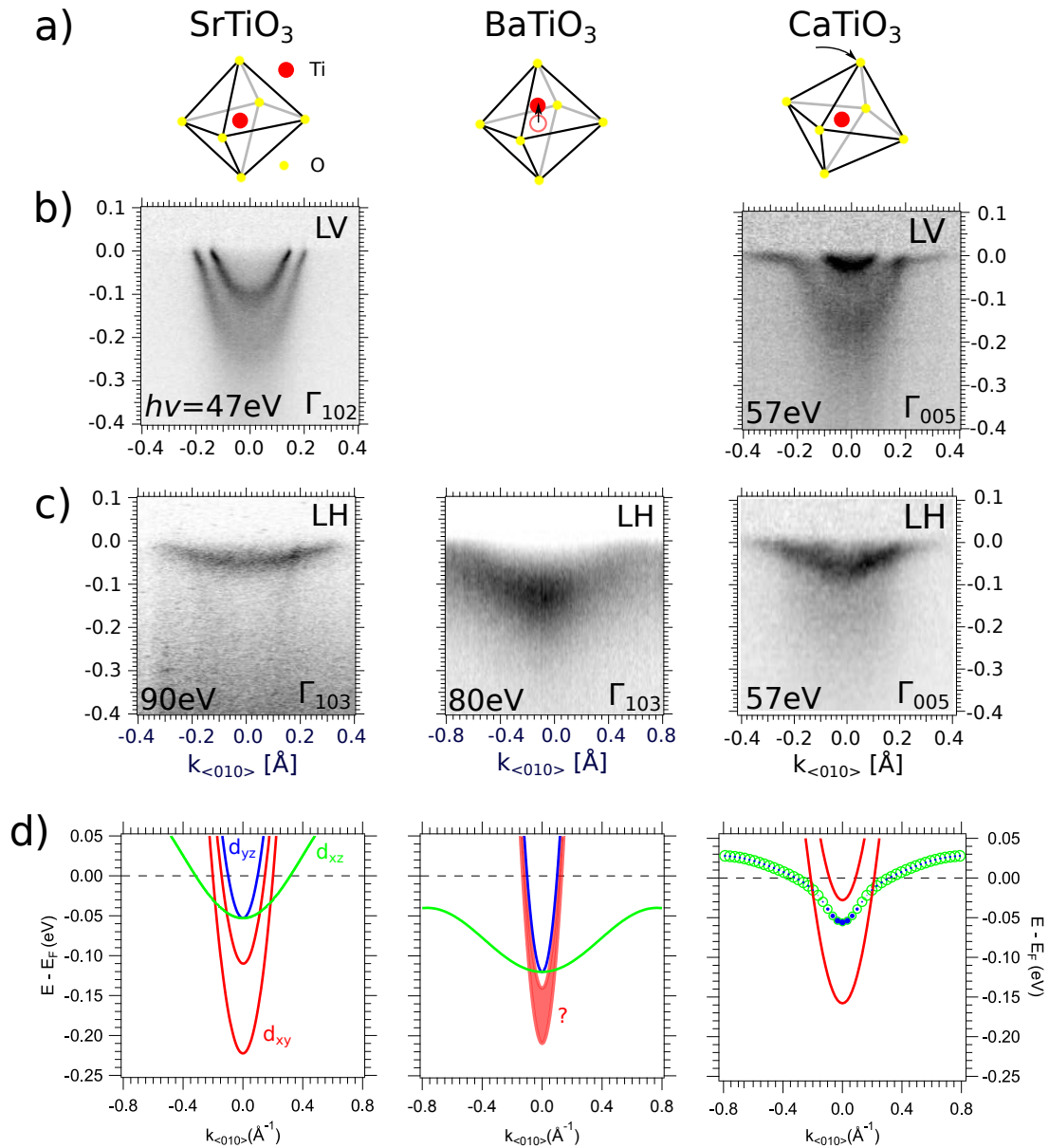
Figure 9.7: (a) Les octaèdres d'oxygènes dans des pérovskites ATiO_3 ( A = Sr, Ba, Ca ), (b,c) les cartes d'intensité ARPES E - k et (d) les schémas de dispersion des bandes observées dans le 2DEGs. (b,c) Des polarisations de lumière différentes ont été utilisées lors des mesures ARPES: (b) linéaire verticale (LV) et (c) linéaire horizontale (LH). Les énergies de photons utilisées pour les mesures et la position des mesures dans l'espace réciproque sont également indiquées sur les graphiques. (d) Car la dispersion de la bande d_{xy} n'a pas pu être déterminée précisément dans le cas de BaTiO_3 , une large bande rouge et un point d'interrogation indiquent la meilleure estimation. La taille des marqueurs pleins et vides dans le cas de CaTiO_3 représentent la fraction de d_{xz} (vert) et de d_{yz} (bleu) dans la dispersion de la bande qui a été obtenu en utilisant un modèle de liaisons fortes.
