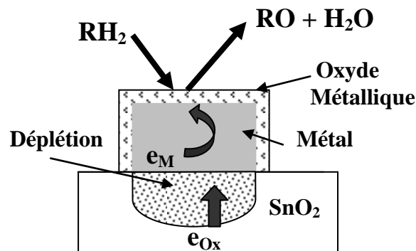
Figure 7 : Schématisation du mécanisme par effet électronique avec formation d'oxyde
