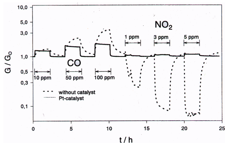
Figure 26 : Caractéristiques électriques sous CO et NO_2 du dispositif SnO_2 associé au Pt proposé par J. Wöllenstein [54].
