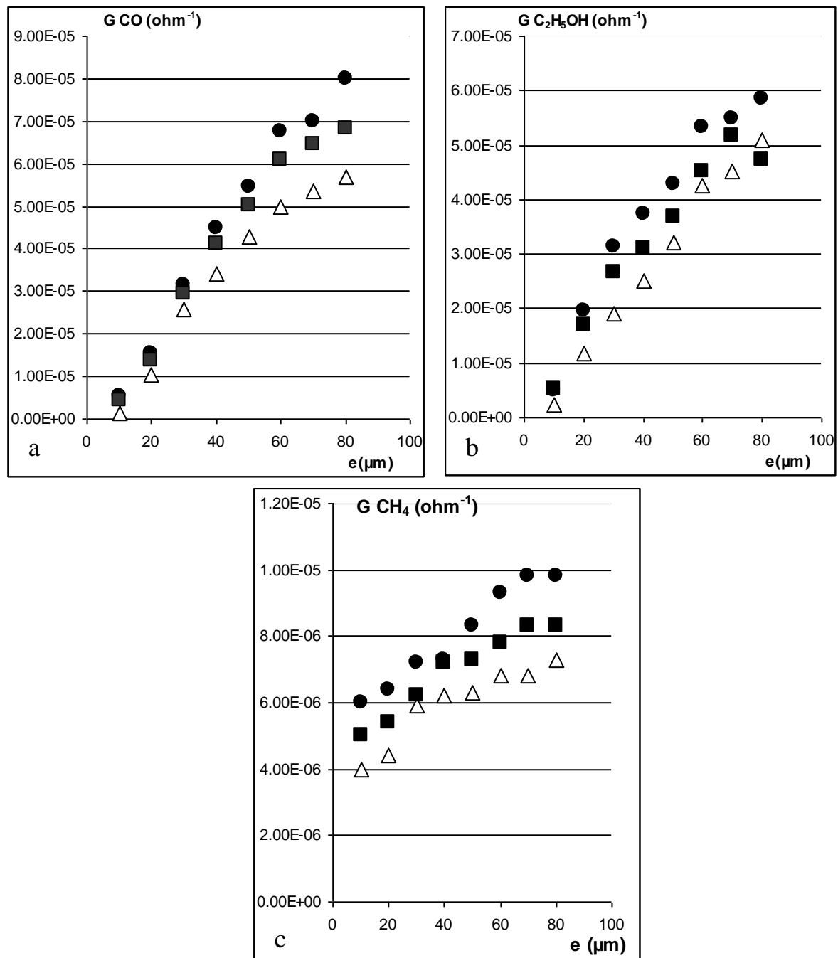
Figure 5: Influence de l'épaisseur des couches épaisses sur la conductance à 500^\circ\text{C} sous a : CO 300 ppm, b : C 2 H 5 OH 100 ppm et c : CH 4 1000 ppm pour 3 séries de 8 capteurs
