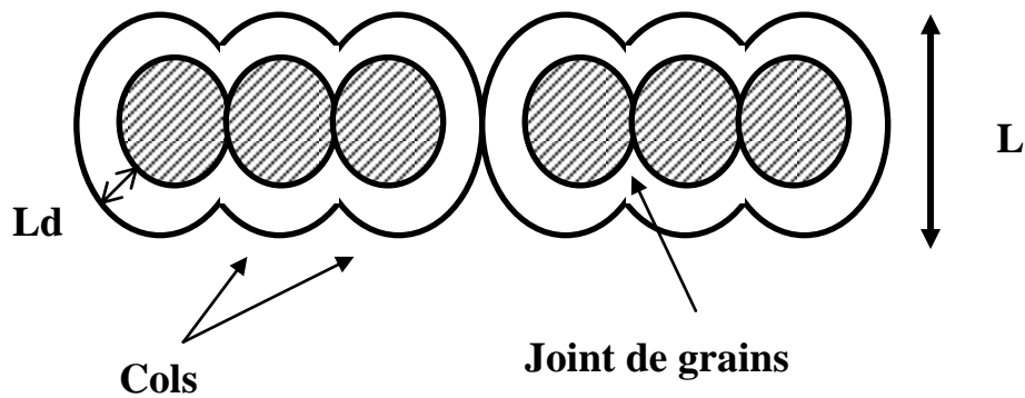
Figure 13 : Notions de cols et de joint de grain dans un matériau polycristallin
