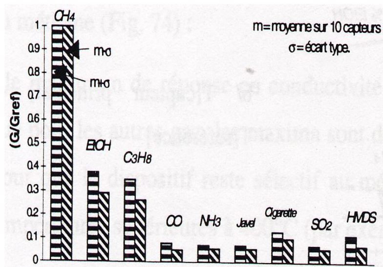
Figure 21 : Caractérisations électriques sous gaz du dispositif sélectif à CH 4 proposé par H. Débéda [48].
