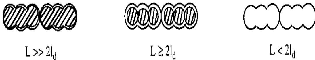
Figure 14 : Modèle de conduction dans \text{SnO}_2 d'après N. Yamazoe [37]. La zone hachurée et la zone non hachurée représentent respectivement la zone non déplétée et la zone déplétée.
