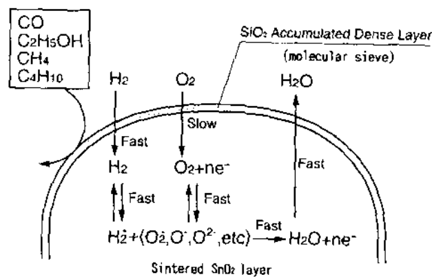
Figure 19 : Modélisation du dispositif proposé par A. Katsuki [44].
