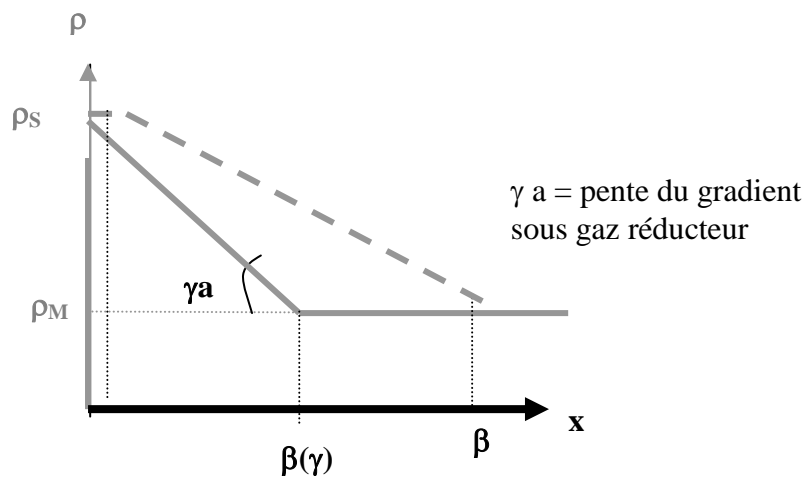
Figure 10 : Distribution de la résistivité dans la zone de déplétion liée au point triple en présence d'un gaz réducteur (trait plein) ou en présence d'air (points tillés).
