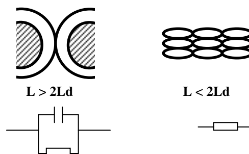
Figure 15 : Schémas électriques équivalents des grains et joints de grains selon la taille des grains proposés par W. Göpel [39].
