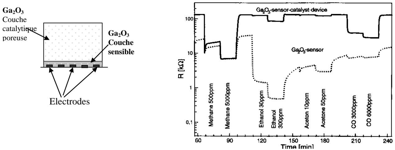
Figure 23 : Système de filtration à base d'oxyde de Gallium et caractérisations électriques sous gaz proposés par M. Fleisher [50].
