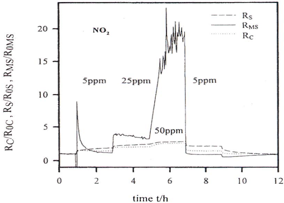
Figure 10 : Effets de NO_2 sur les valeurs de R_S (résistance du bulk), R_{MS} (résistance proche des électrodes) et R_C (résistance de contact) obtenus par TLM sur des capteurs SnO_2 selon U. Hoefler [31 ].
