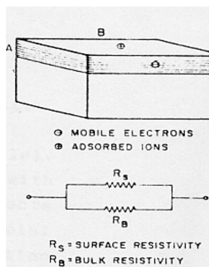
Figure 12 : Modèle macroscopique selon J. Gutierrez [35]
