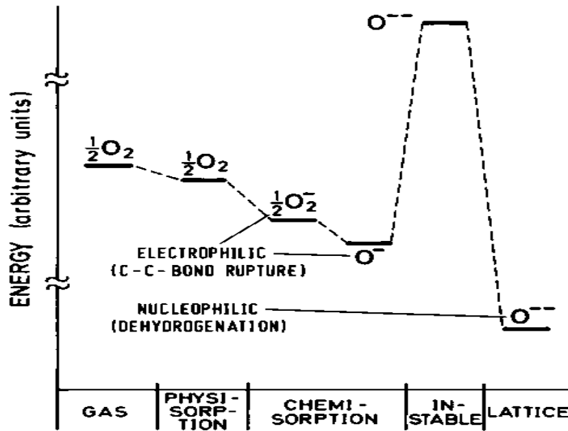
Figure 2 : Diagramme énergétique des divers oxygènes présents aux états gazeux, en phase adsorbée et liés à un élément du réseau selon A .Bielanski [8]
