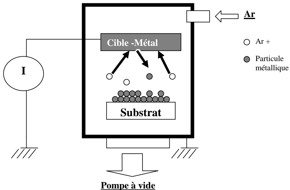
Figure 5 : Principe de la pulvérisation cathodique
