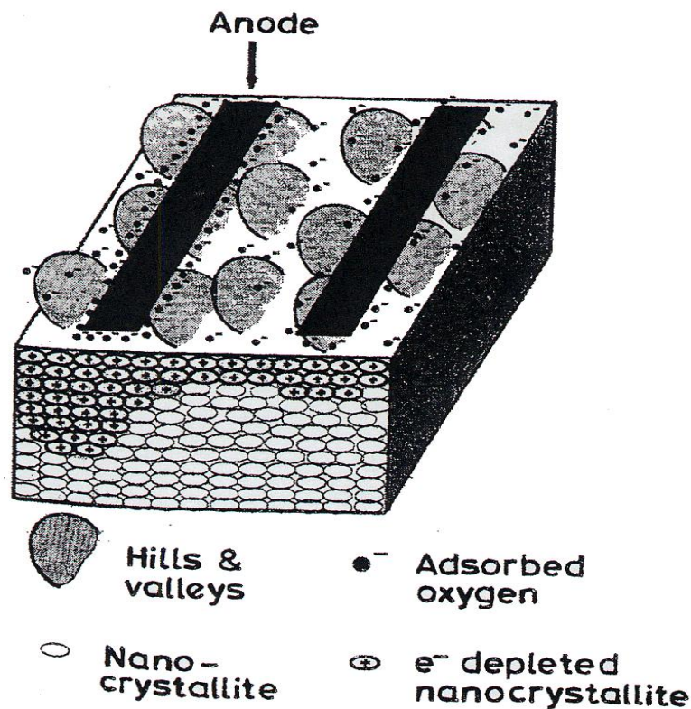
Figure 11 : Modélisation du rôle des électrodes proposée par K.Varghese [34].
