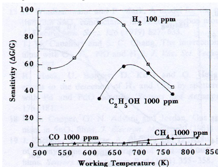
Figure 25 : Caractéristiques électriques sous gaz réducteur du dispositif SnO 2 associé au Pd proposé par G. Sberveglieri [53].
