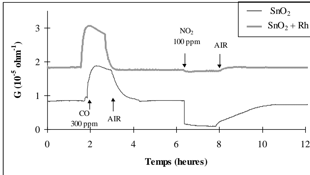
Figure 27 : Influence d'un film de rhodium sur les propriétés de détection d'une couche mince de dioxyde d'étain selon C. Pijolat [56]
