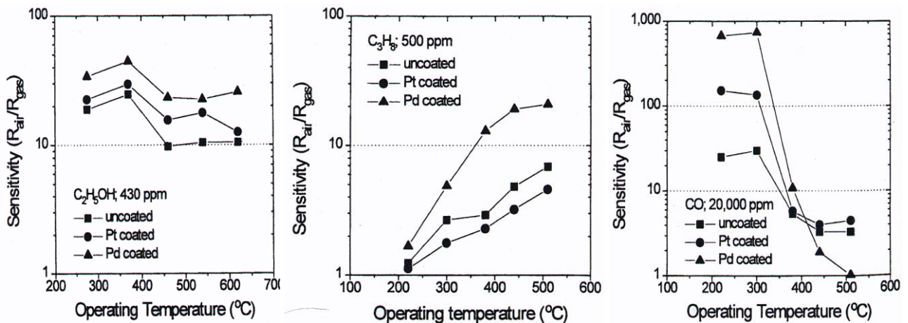
Figure 22 : Effets comparés du Pt et du Pd pour le dispositif proposé par Kwon [49].
