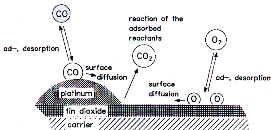
Figure 5 : Mécanisme de reverse spill-over concernant l'oxygène proposé par K. Grass [23]
