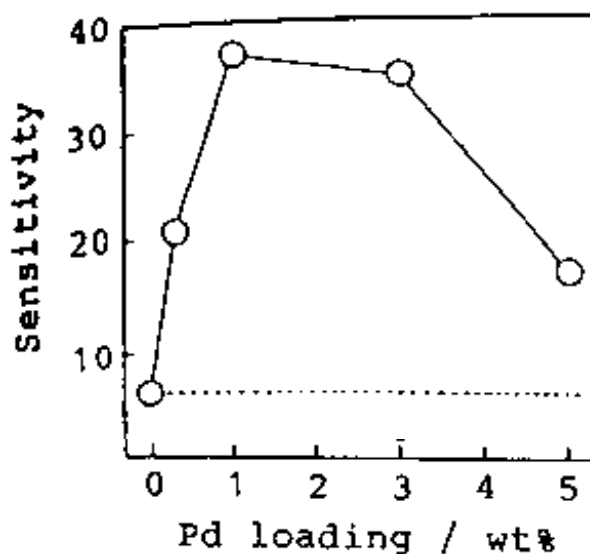
Figure 8 : Exemple de sensibilisation électronique obtenue par ajout de palladium dans \text{SnO}_2 selon Matsushima à 100 °C. La sensibilité est définie par G(\text{H}_2)/G(\text{air}) [26].
