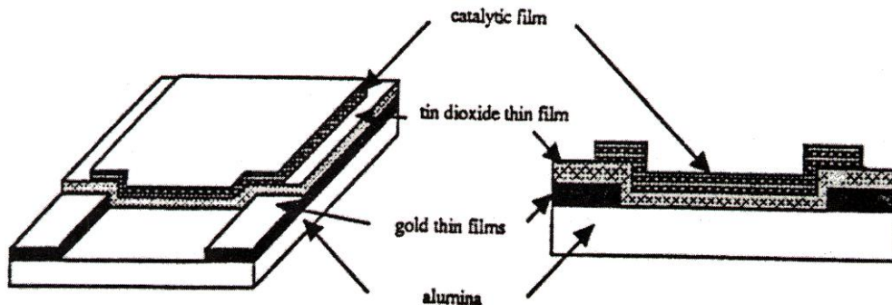
Figure 24 : Dispositif matériau sensible associé à un film métallique proposé en couches minces selon M. Sauvan [52].
