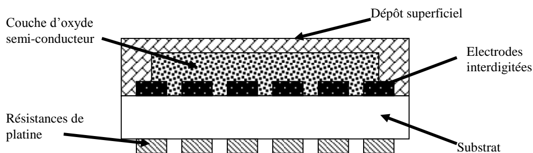
Figure 20 : Structure sérigraphiée matériau sensible associé à une membrane proposé par F. Ménil [46].
