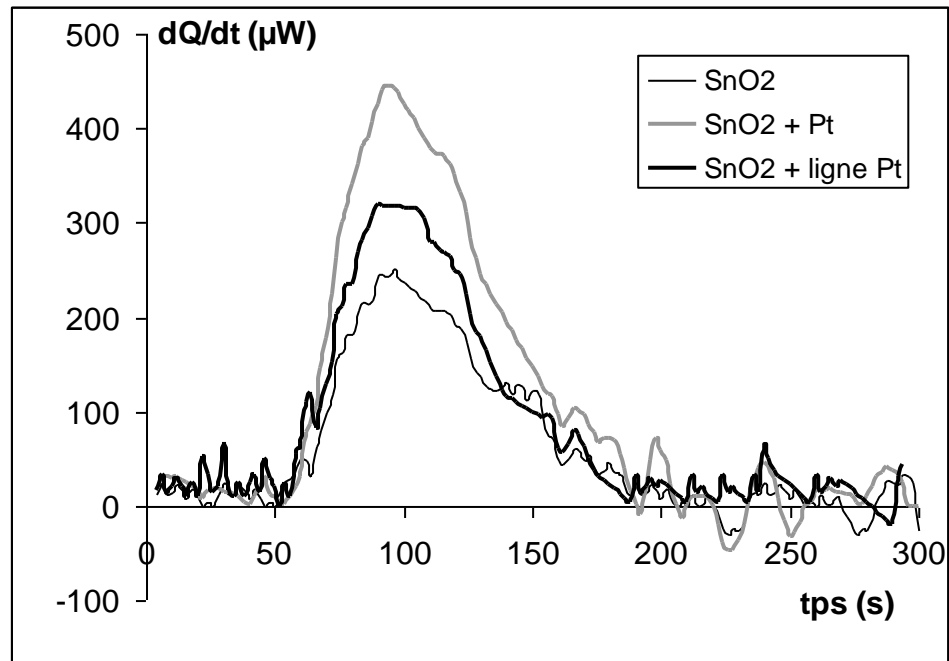
Figure 17 : Thermogrammes obtenus avec les différents types d'échantillons pour une température de 400°C et pour variations de pression d'oxygène de 2 mbar.
