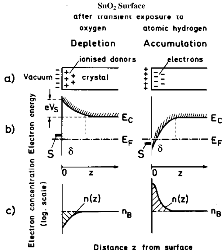
Figure 1 : Zone de charge d'espace à la surface d'un semi-conducteur de type n. a) distribution des charges, b) structure des bandes, c) concentration n(z) en électrons de la bande de conduction selon D. Kohl [3].
