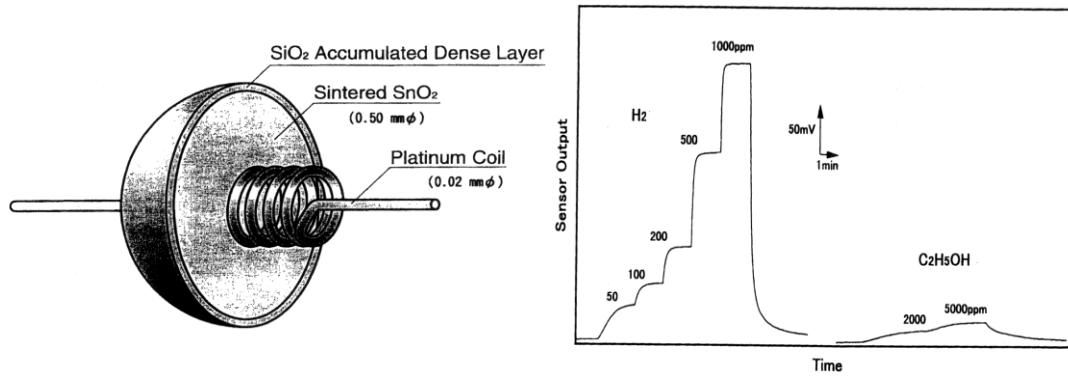
Figure 18 : Dispositif sélectif à H 2 proposé par A. Katsuki [44].
