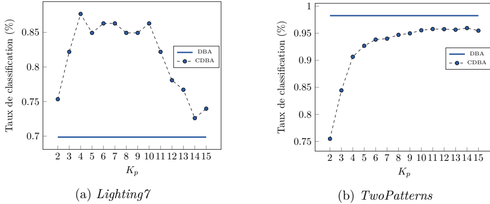
FIGURE 3.12 – Taux de classification en fonction de K_p pour deux bases de données : (a) Lighting7 qui contient des signaux peu décalés et (b) TwoPatterns qui contient des signaux très décalés. Il convient de noter que la valeur optimale de K_p dépend des décalages des signaux intraclasse.
