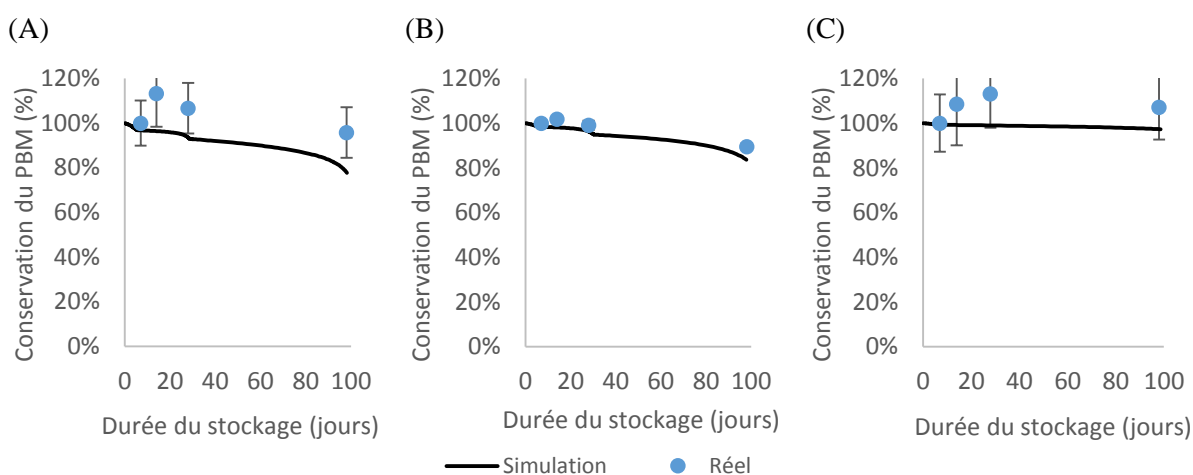
Figure 5-13 – Estimations avec les résultats des simulations et données expérimentales pour la conservation du potentiel bio-méthanogène de la CIVE 2. (A) TS10%E ; (B) TS14%E ; (C) TS39%E.
