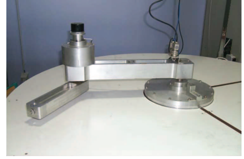
Fig. 8. Scara robot prototype.
