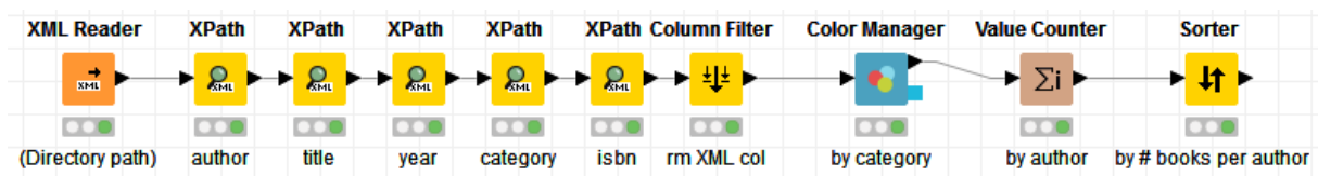
FIGURE 5.15 : Un exemple d'un workflow KNIME.
