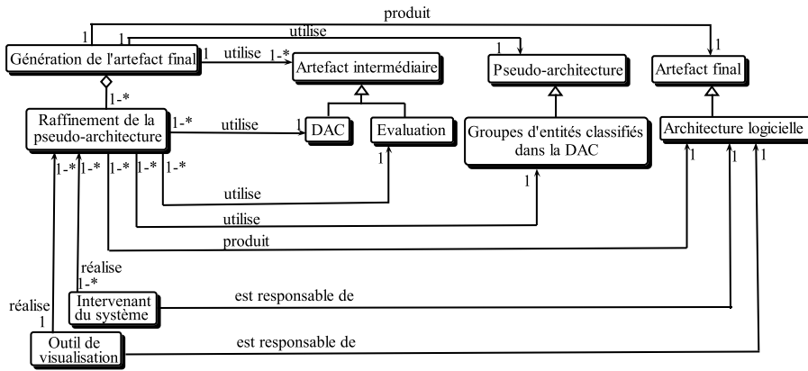
FIGURE 3.12 : Le mécanisme opératoire de la génération de l'artefact final.
