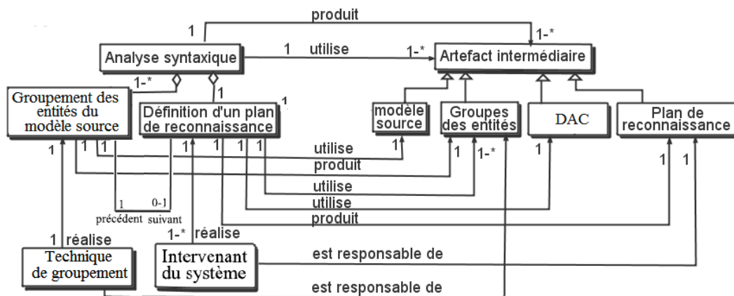
FIGURE 3.9 : Le mécanisme opératoire de l'analyse syntaxique.
