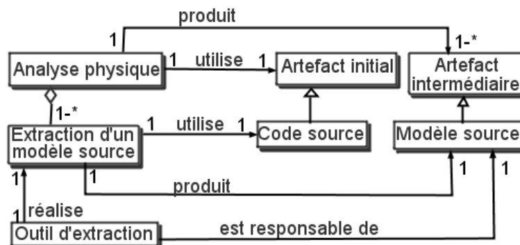
FIGURE 3.8 : Le mécanisme opératoire de l'analyse physique.
