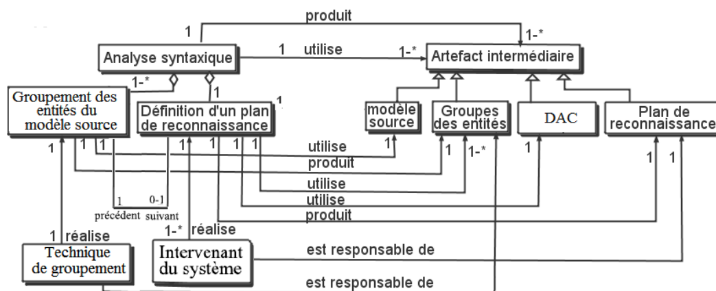
FIGURE 3.9 : Le mécanisme opératoire de l'analyse syntaxique.
