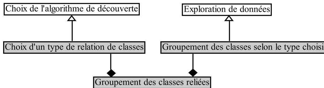
FIGURE 5.9 : Les relations entre le groupement des classes reliées d'une part et le choix de l'algorithme de découverte et l'exploration de données d'autre part.
