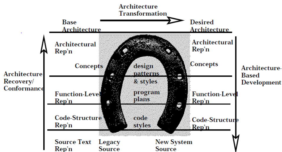
FIGURE 1.2 : Le modèle conceptuel du fer à cheval : extrait du [Kazman et al., 1998].
