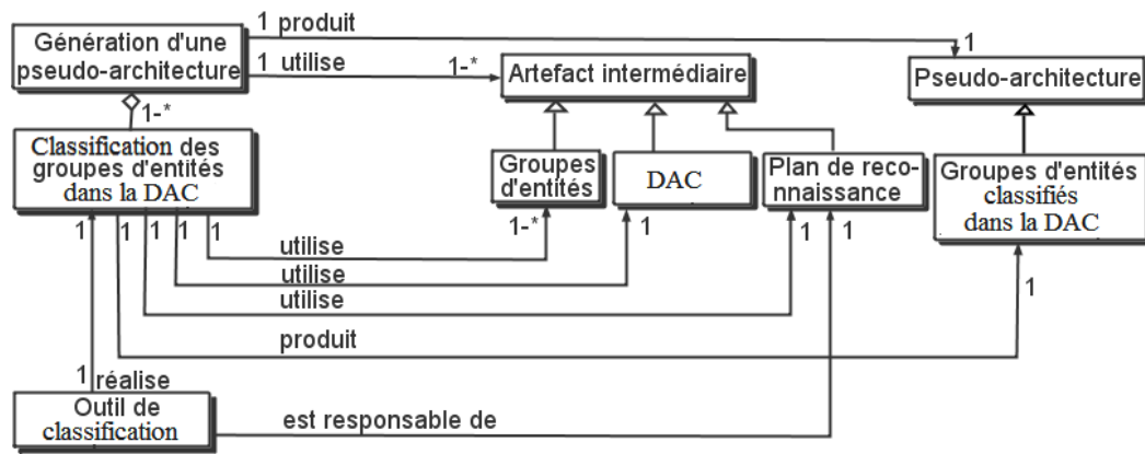
FIGURE 3.10 : Le mécanisme opératoire de la génération d'une pseudo-architecture.
