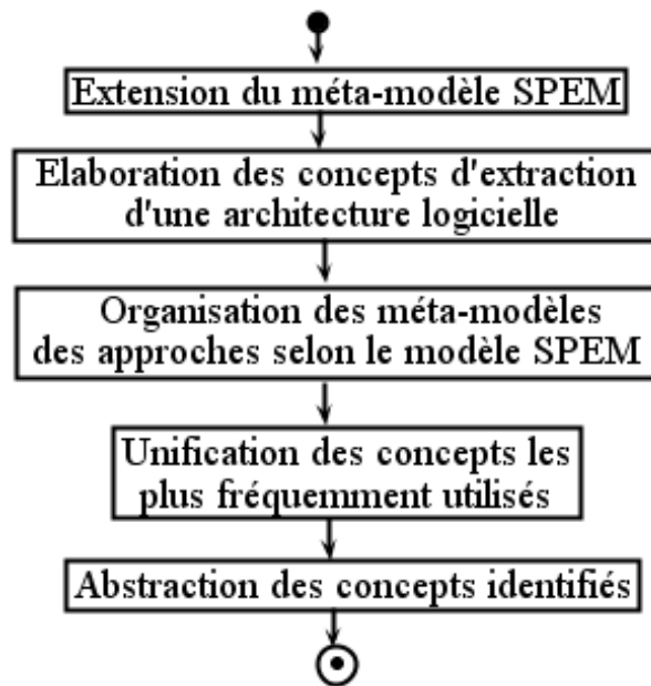
FIGURE 3.2 : Les activités réalisées pour l'élaboration du méta-modèle SAREM.
