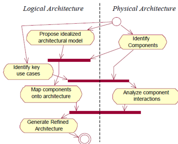
FIGURE 1.6 : Les différentes activités de l'approche Focus pour la reconstruction d'une l'architecture : extrait du [Ding et Medvidovic, 2001]
