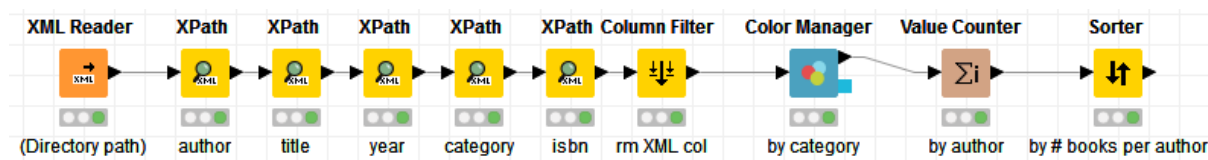
FIGURE 5.15 : Un exemple d'un workflow KNIME.
