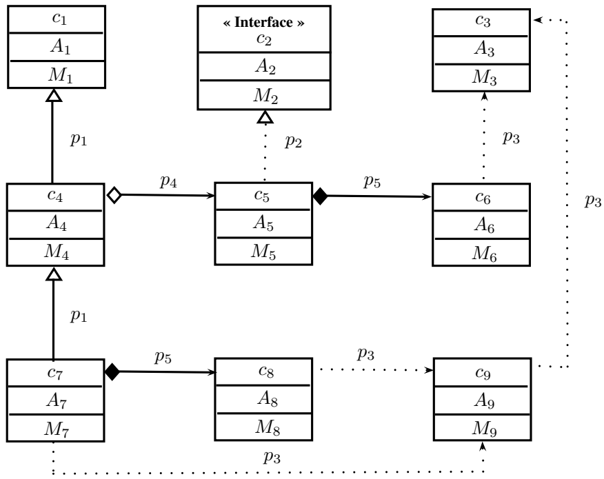
FIGURE 4.4 : Un diagramme de classes avec les relations de classes pondérées.
