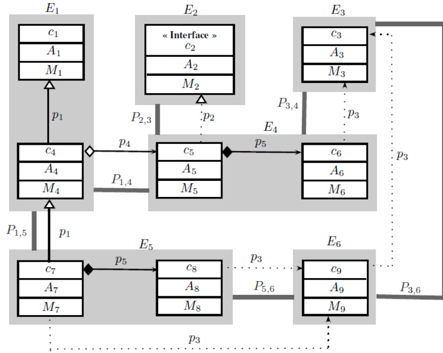
FIGURE 4.5 : Les éléments et leurs connecteurs.
