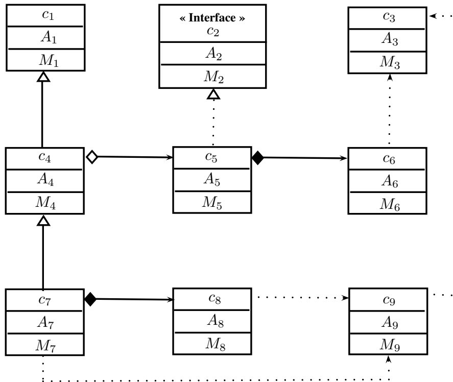
FIGURE 4.2 : Un diagramme de classe selon la notation UML.
