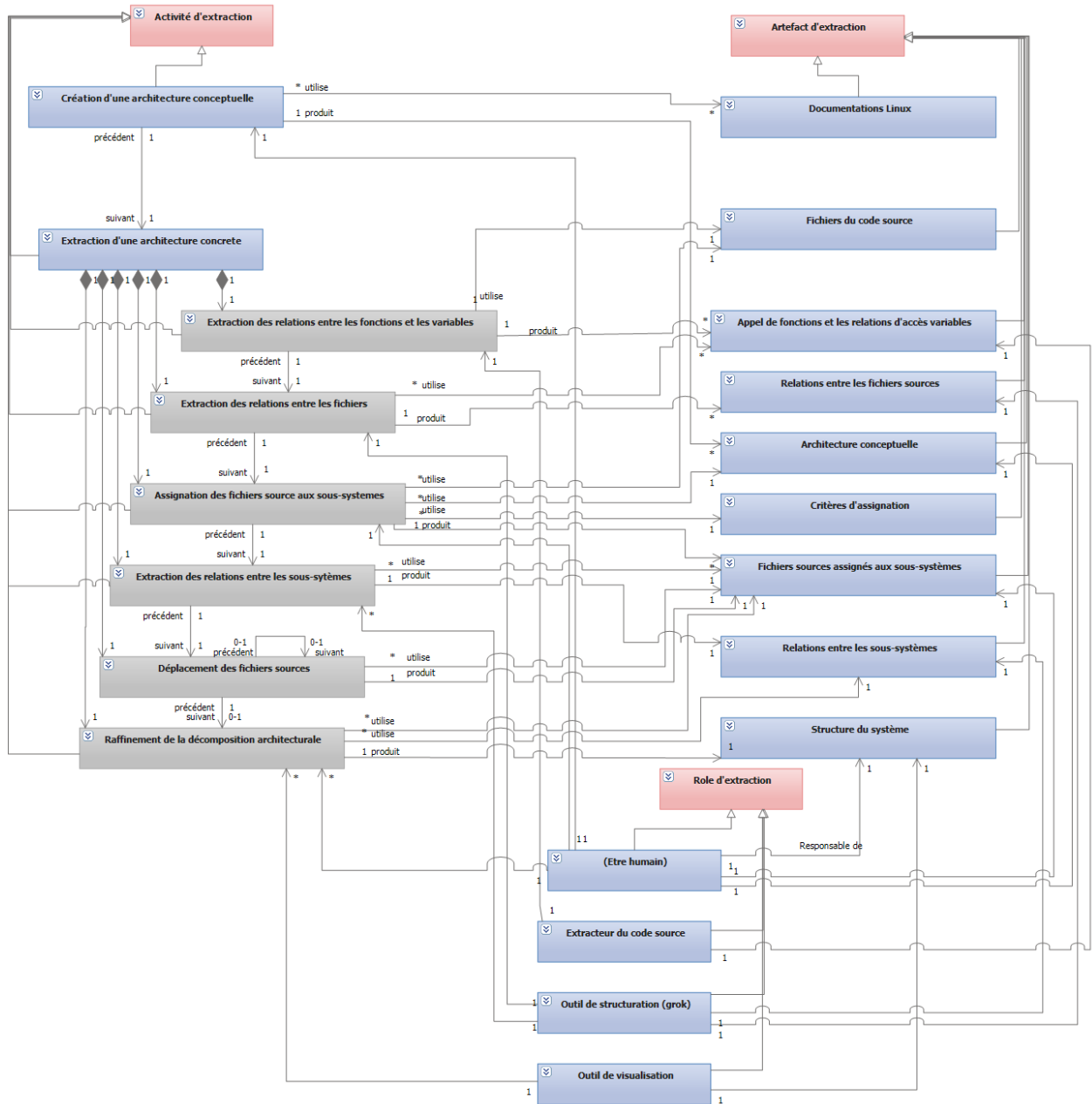
FIGURE 3.15 : Le méta-modèle élaboré de l'approche proposée par Bowman et al.
