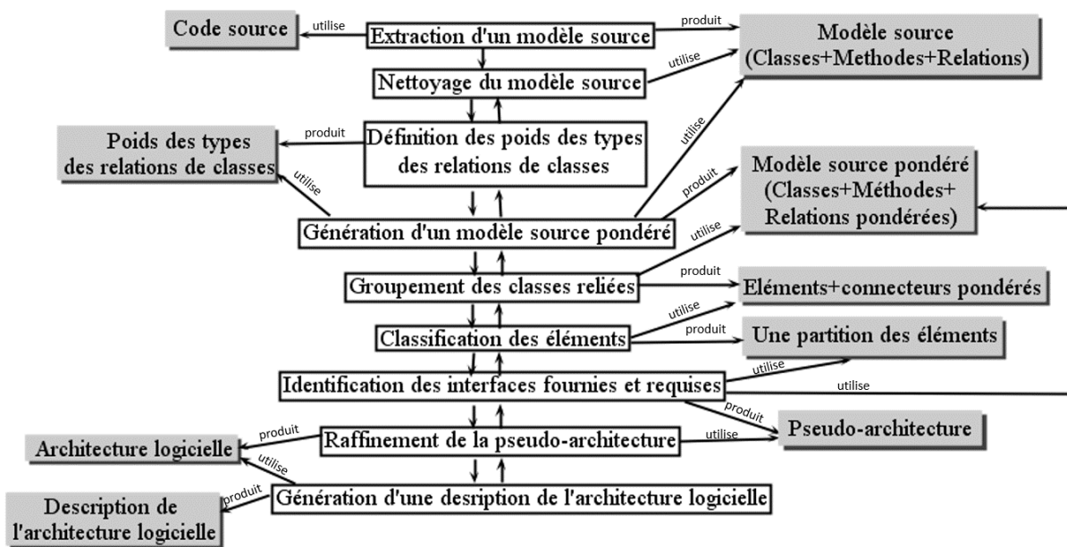
FIGURE 4.1 : Les activités et les artefacts du modèle SAD.
