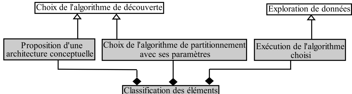
FIGURE 5.10 : Les relations entre la classification des éléments d'une part et le choix de l'algorithme de découverte et l'exploration de données d'autre part.
