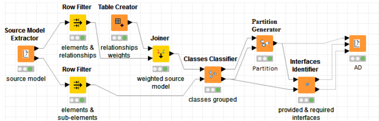
FIGURE 5.16 : Un workflow KNIME qui extrait une architecture de logicielle.
