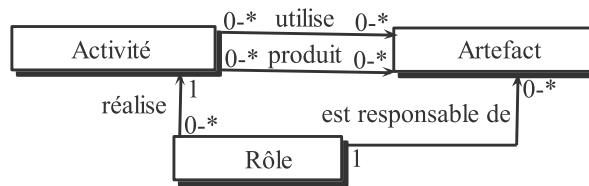
FIGURE 3.1 : Le méta-modèle du SPEM.
