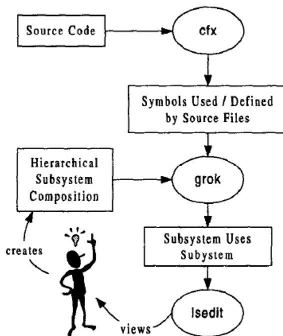
FIGURE 1.5 : Le processus de l'extraction proposé par Bowman : extrait du [Bowman et al., 1999].
