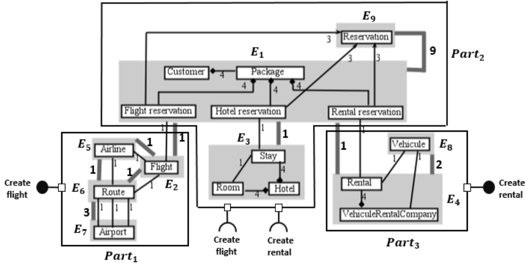
FIGURE 4.13 : Une pseudo-architecture.
