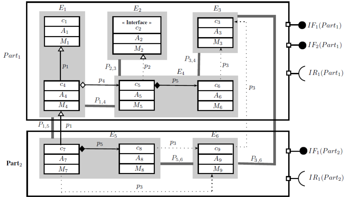
FIGURE 4.7 : Une pseudo-architecture.
