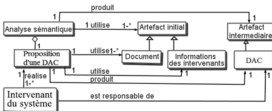
FIGURE 3.7 : Le mécanisme opératoire de l'analyse sémantique.
