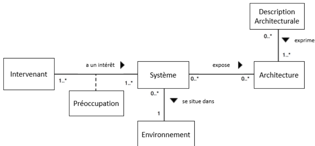
FIGURE 1.1 : Les termes et les concepts liés à l'architecture logicielle et l'AD : extrait de [ISO, 2011].
