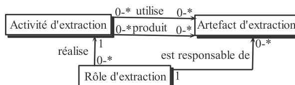
FIGURE 3.3 : Une extension du méta-modèle SPEM.
