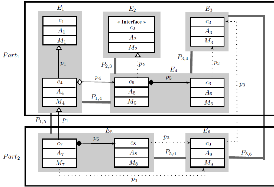
FIGURE 4.6 : La partition des éléments.
