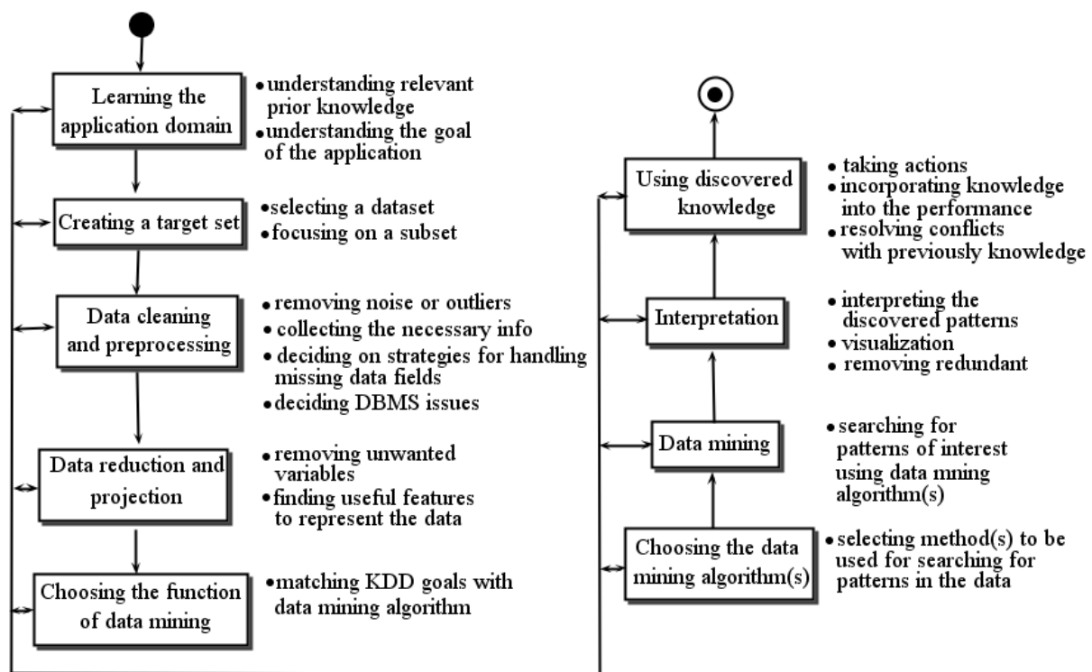
FIGURE 5.3 : Un diagramme d'activité qui illustre le modèle du processus ECD.
