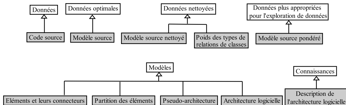
FIGURE 5.14 : Les relations entre les artefacts du modèle SAD et ceux du modèle ECD.
