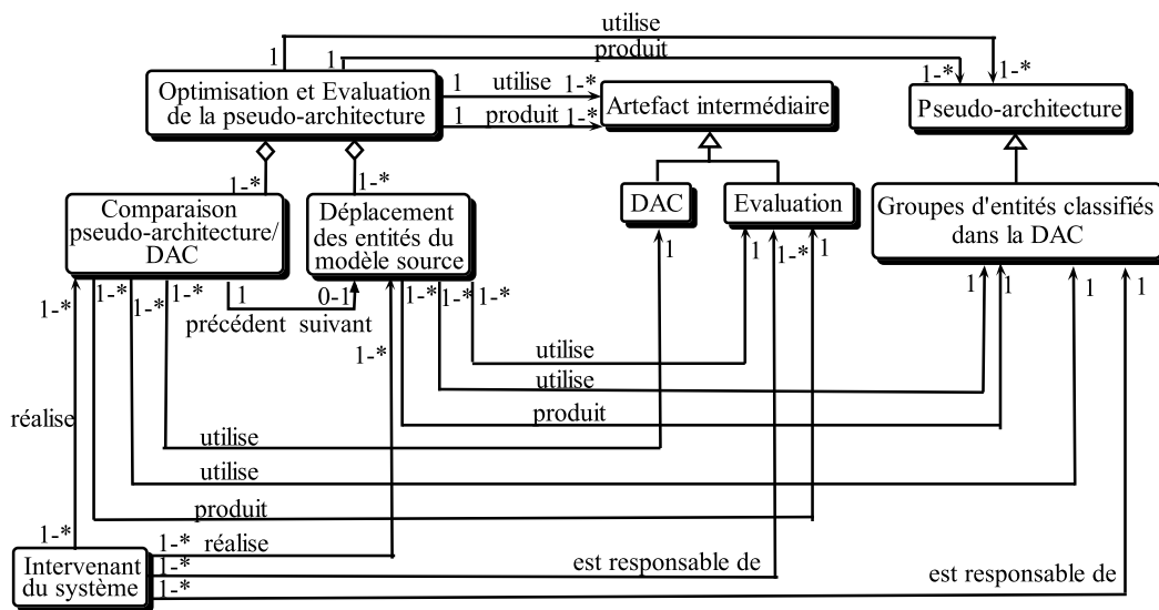
FIGURE 3.11 : Le mécanisme opératoire de l'optimisation et l'évaluation de la pseudo-architecture.
