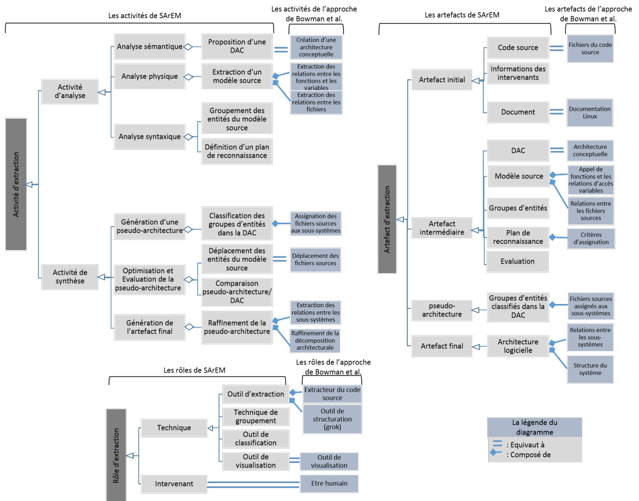
FIGURE 3.16 : La conformité de SAREM à l'approche proposée par Bowman et al.
