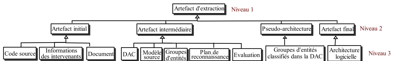
FIGURE 3.4 : Les artefacts d'extraction de SArEM
