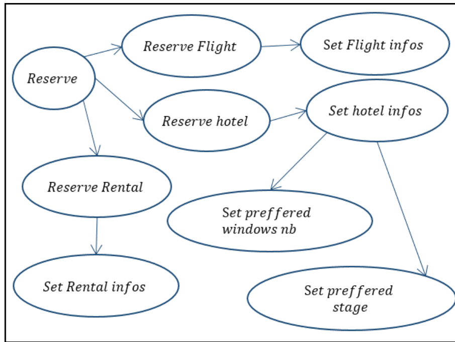
FIGURE 4.9 : Les appels des méthodes du modèle source représentés par un graphe d'appels.
