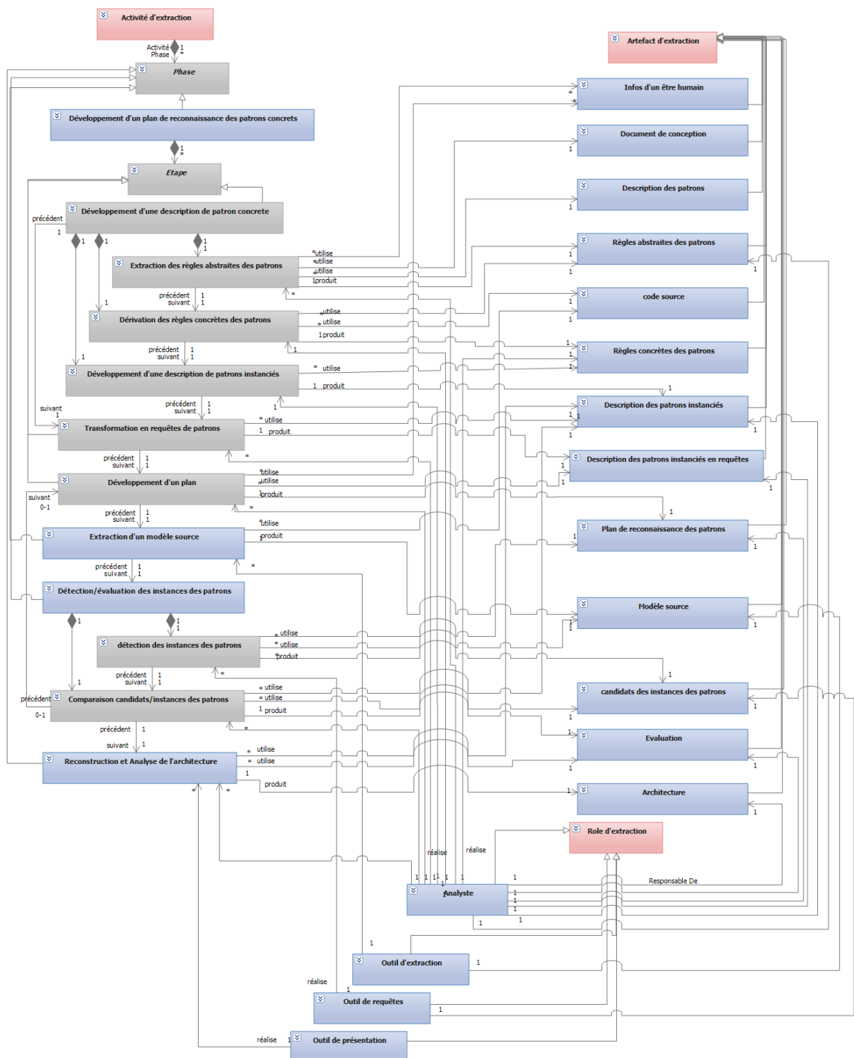
FIGURE 3.13 : Le méta-modèle élaboré de l'approche ARM.
