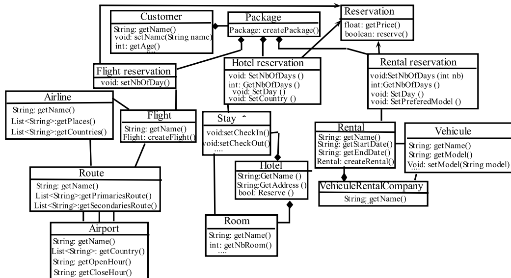
FIGURE 4.8 : Les classes, leurs opérations et relations du modèle source.
