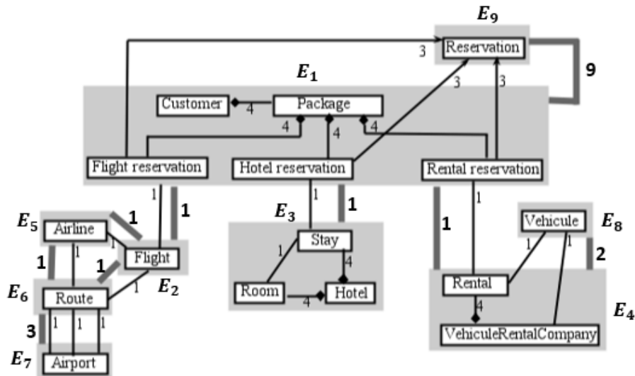
FIGURE 4.11 : Les éléments et leurs connecteurs pondérés.
