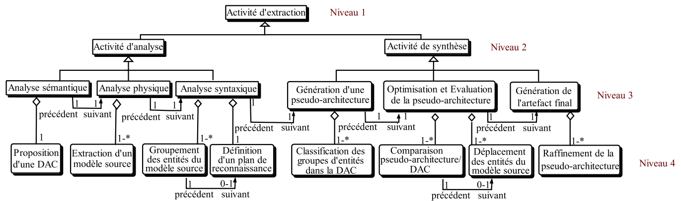
FIGURE 3.5 : Les activités d'extraction de SAREM
