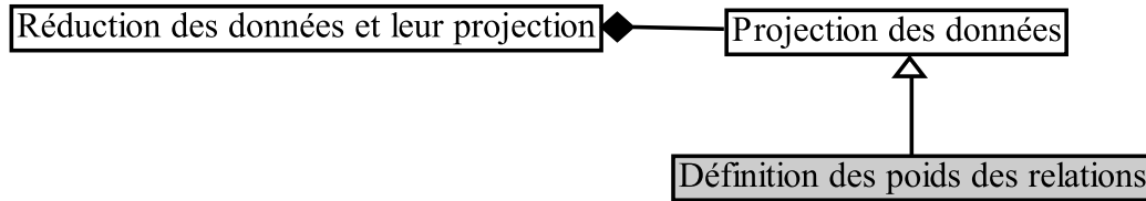
FIGURE 5.7 : Les relations entre la définition des poids des relations et la projection des données.
