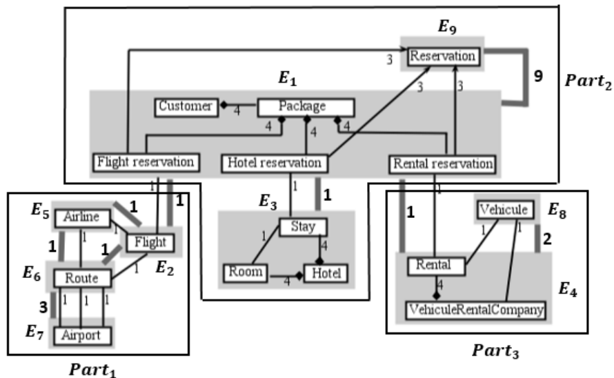
FIGURE 4.12 : Une pseudo-architecture.
