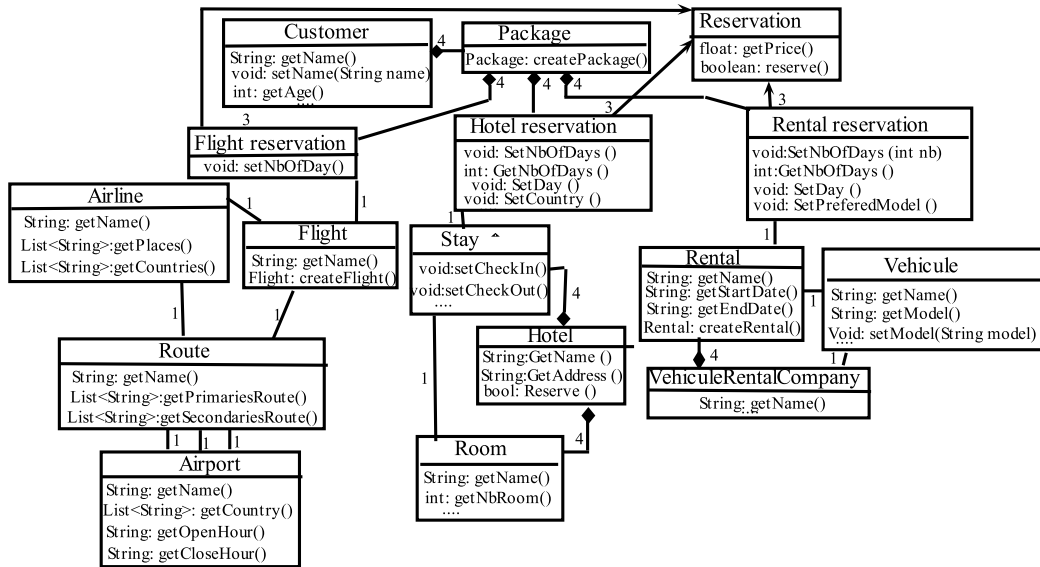
FIGURE 4.10 : Un modèle source pondéré extrait d'un système de réservation.
