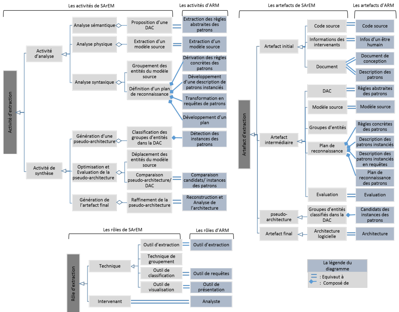
FIGURE 3.14 : La conformité de SAREM à l'approche ARM.
