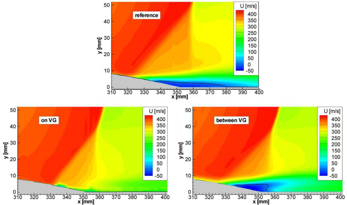
Figure 19 - Iso-contours de la composante de vitesse longitudinale de l'interaction onde de choc / couche limite sans contrôle (haut) et avec contrôle par les VGs « contra-rotatifs » C2 (bas), et ligne U = 0 en noir
