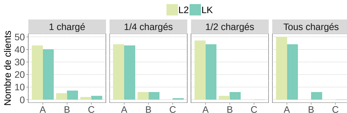
FIGURE 4.11 – Distribution des requêtes déléguées pour Ladda 2 (L2) et Ladda K (LK), dans les configurations : 1 chargé , 1/4 chargés , 1/2 chargés et Tous chargés ; où la catégorie A correspond aux clients ayant effectués moins de 60 requêtes déléguées, la catégorie B correspond aux clients ayant effectués entre 60 et 120 requêtes déléguées et la catégorie C correspond aux clients ayant effectués plus de 120 requêtes déléguées. Moyenne sur 3 exécutions.
