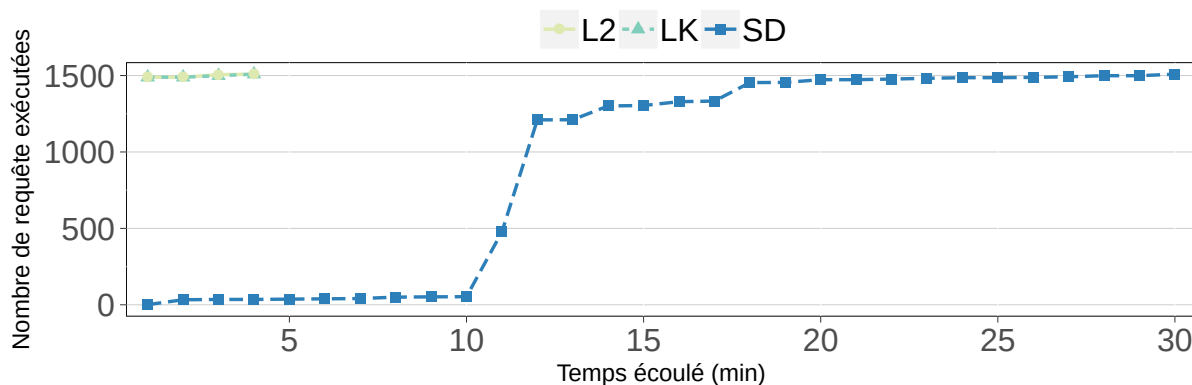
FIGURE A.3 – Nombre de requêtes exécutées par minute par Ladda 2 (L2), Ladda K (LK) et l'approche de référence Sans délégation (SD) dans la configuration 1 chargée.
