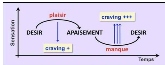
Figure 23 : Sinusoïde Manque-Désir-Plaisir-Apaisement (48)
