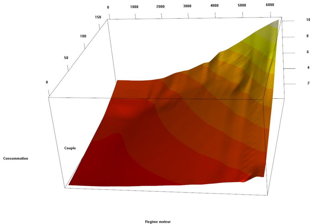
Figure 27 : Interpolation de la cartographie moteur d'une Laguna II permettant de calculer la consommation instantanée (en gr/sec) en fonction du couple et du régime du moteur (en tours/min).
