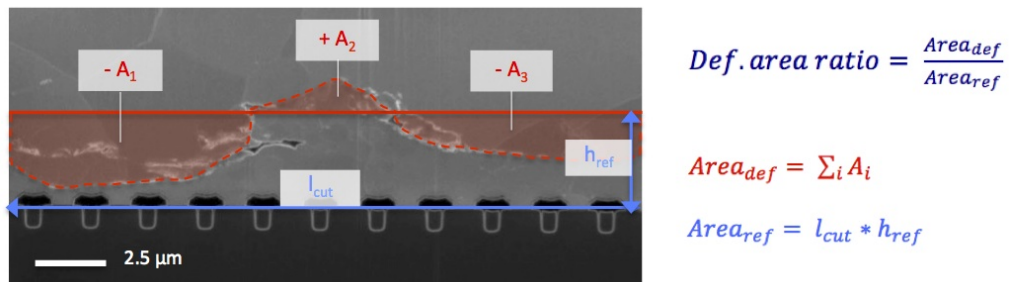
Figure 151: Méthode de mesure de la déformation plastique imposée par les fils de bonding (en haut) à la métallisation de la source (en bas).
