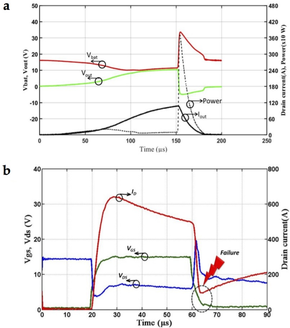
Figure 142: Formes d'onde au moment de la défaillance pour un composant (a) To7D17 soumis à des tests de qualification standard chez NXP et (b) SPD06 vieilli au sein du laboratoire SATIE par de test de court-circuit extrêmes.
