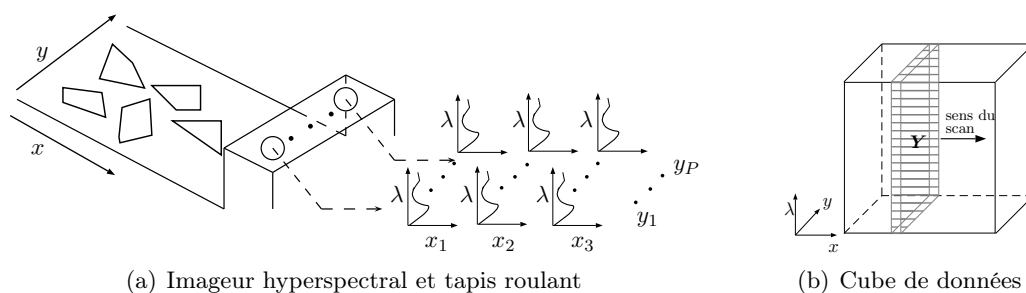
FIGURE 4.2 : Images hyperspectrales acquises par un spectro-imageur NIR industriel. La matrice \mathbf{Y} est une tranche du cube de données. (x, y) dimensions spatiales ; (\lambda) dimension spectrale
