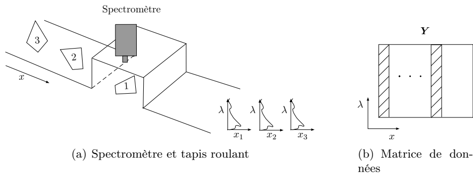
FIGURE 4.1 : Construction de la matrice de données composée de spectres acquis par un spectromètre placé dans une cabine. Le tapis roulant entraîne les pièces à scanner. (x) dimension spatiale ; (\lambda) dimension spectrale
