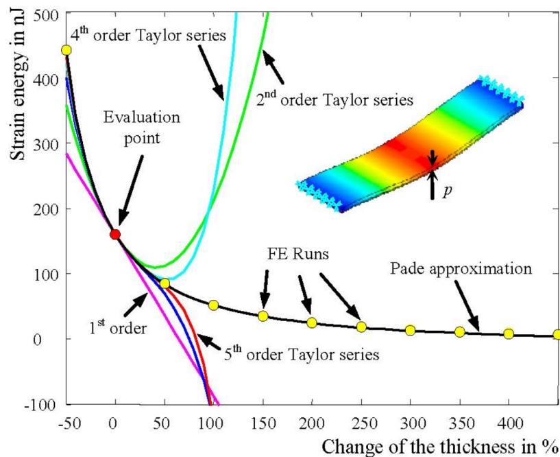
FIGURE 5.1 – Sensibilité de haut-degré de l'énergie de contrainte d'une poutre encadrée par rapport à son épaisseur [Issu de Kolchuzhin et al. , 2007]. La poutre est modélisée par éléments finis et la précision des approximations de haut-degré comparées à un calcul direct par éléments finis pour d'autres valeurs des paramètres.
